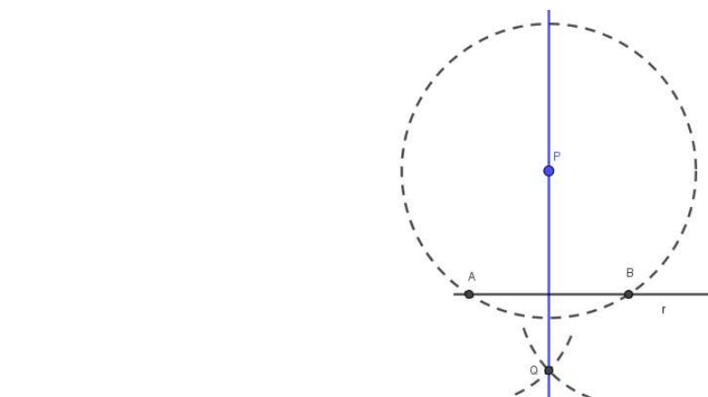
Figura 2.15: Reta perpendicular por um ponto P \notin r
