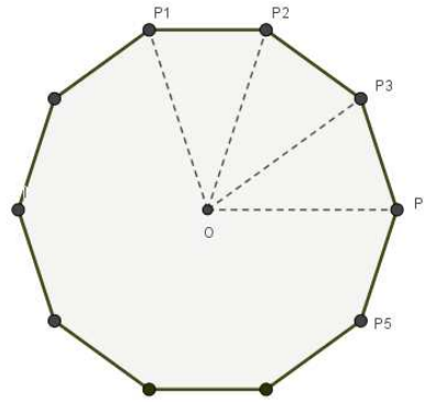
Figura 3.3: Polígono inscrito em um círculo
