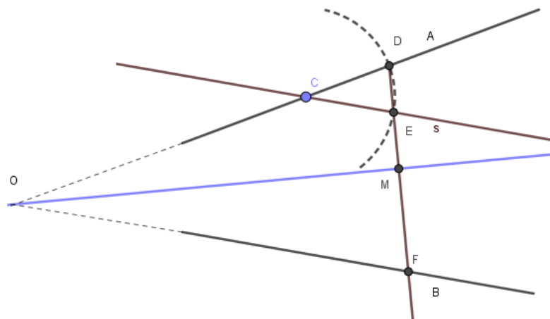
Figura 2.19: Bissetriz desconhecendo o vértice
