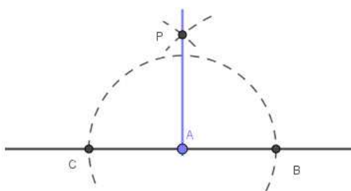
Figura 2.25: Ângulo de 90^\circ através do ângulo raso
