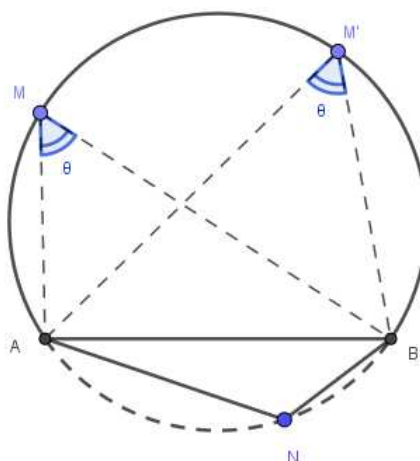
Figura 2.28: Arco capaz
