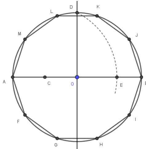
Figura 3.9: Decágono inscrito na circunferência
