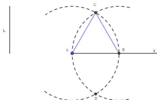
Figura 2.20: Triângulo equilátero
