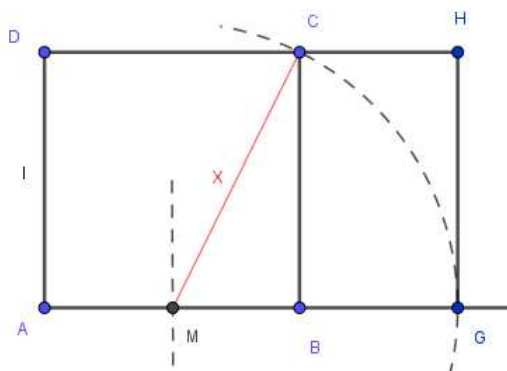
Figura 2.40: Retângulo áureo
