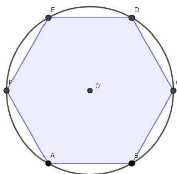
Figura 3.1: Polígono inscrito
