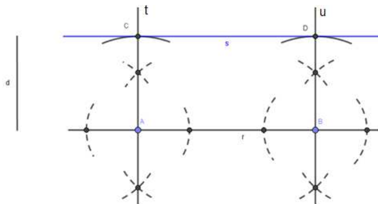
Figura 2.16: Retas paralelas
