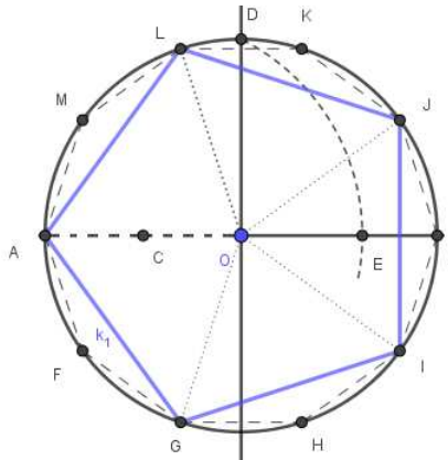
Figura 3.11: Pentágono regular
