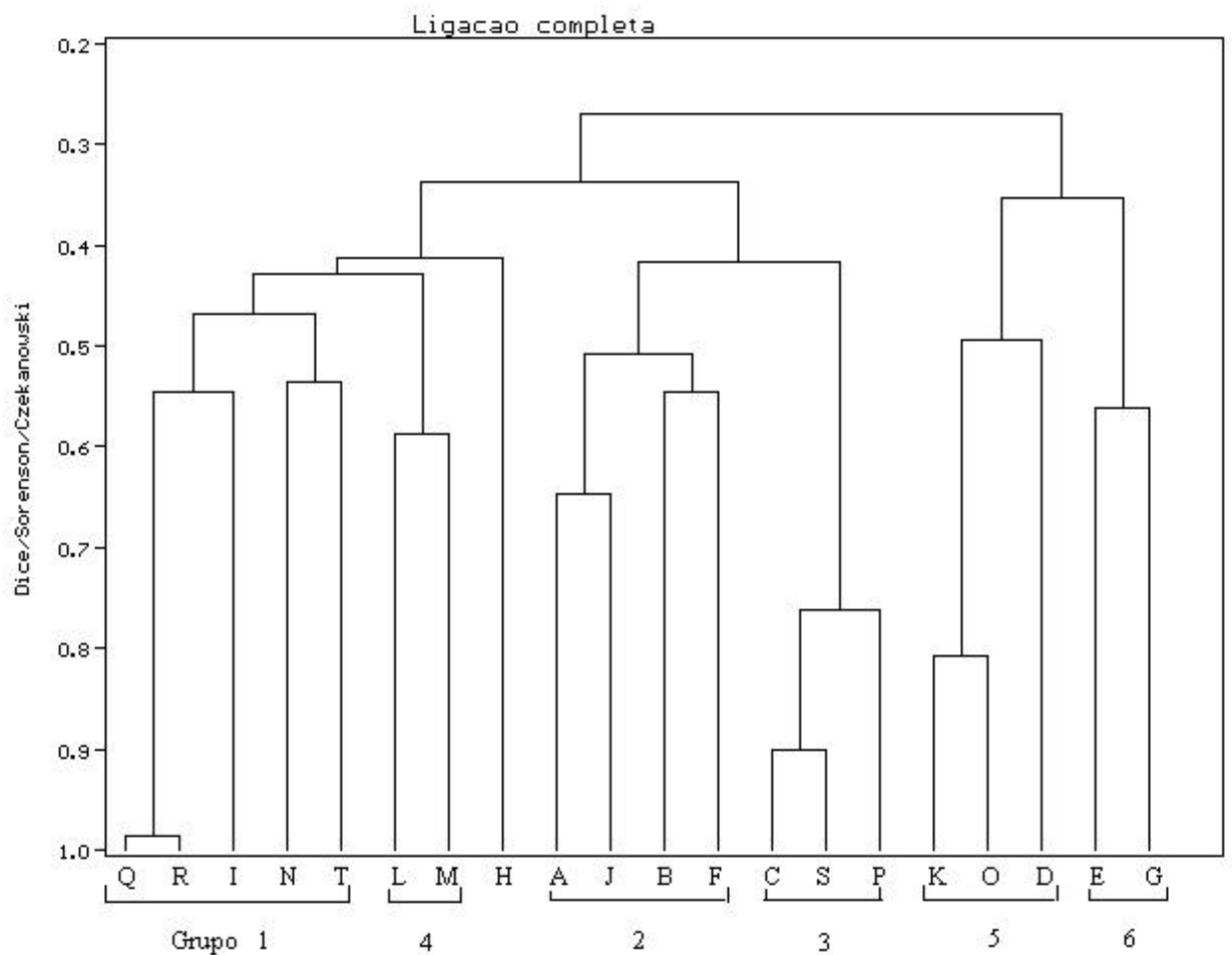
FIGURA 5 – Dendrograma da análise de agrupamentos por ligações completas das similaridades florísticas (Sørensen) entre 20 remanescentes florestais do município de Viçosa-MG. A = UFV (Lopes et al., 2002); B = Mata da Silvicultura - UFV (Meira-Neto & Martins, 2000); C = Mata da Biologia - UFV (Paula et al., 2002); D = Mata da Pedreira (Marangon et al., 2003); E = Fazenda Bom Sucesso (Irsigler, 2002); F = Mata do Juquinha (Silva et al., 2004); G = Fazenda Bom Sucesso (Campos, 2002); H = Fazenda Tico-Tico (Soares Júnior, 2000); I = Fazenda Rancho Fundo (Senra, 2000); J = Fazenda São Geraldo (Silva et al., 2003a); K = Mata do Paraíso (Silva, 2003); L = Área 1 (Almeida Júnior, 1999); M = Área 4 (Almeida Júnior, 1999); N = Sítio Palmital (Ribas et al., 2003); O = Mata do Paraíso (Fernandes, 1998); P = Mata da Biologia - UFV (Silva et al., 2000); Q = Mata da Garagem (Silva et al., 2003b); R = Mata da Garagem (Silva et al., 2002); S = Mata da Biologia (Gasparini-Júnior, 2004); T = Mata da Agronomia (Presente estudo).
