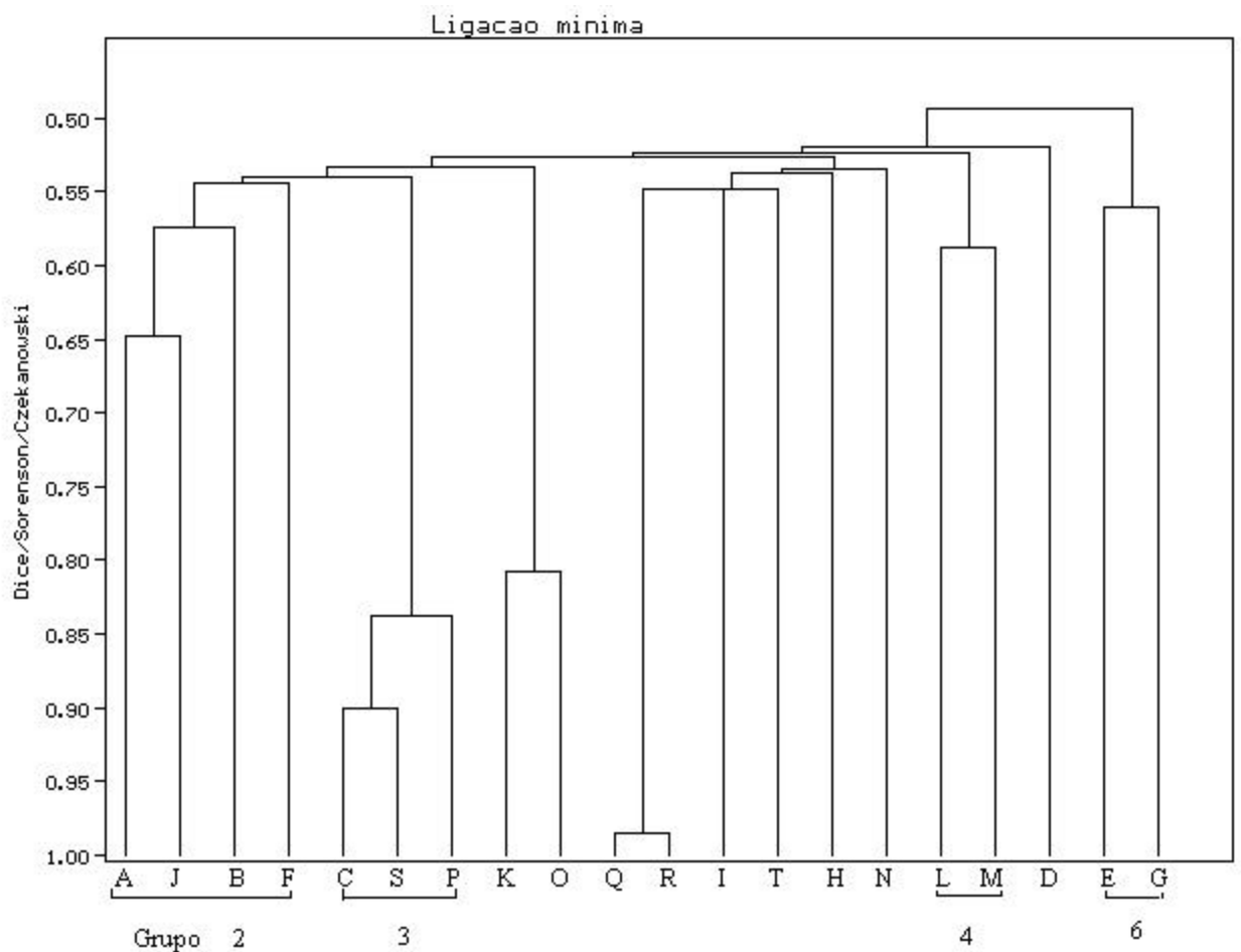
FIGURA 6 – Dendrograma da análise de agrupamentos por ligações simples das similaridades florísticas (Sørensen) entre 20 remanescentes florestais do município de Viçosa-MG. A = UFV (Lopes et al., 2002); B = Mata da Silvicultura - UFV (Meira-Neto & Martins, 2000); C = Mata da Biologia - UFV (Paula et al., 2002); D = Mata da Pedreira (Marangon et al., 2003); E = Fazenda Bom Sucesso (Irsigler, 2002); F = Mata do Juquinha (Silva et al., 2004); G = Fazenda Bom Sucesso (Campos, 2002); H = Fazenda Tico-Tico (Soares Júnior, 2000); I = Fazenda Rancho Fundo (Senra, 2000); J = Fazenda São Geraldo (Silva et al., 2003a); K = Mata do Paraíso (Silva, 2003); L = Área 1 (Almeida Júnior, 1999); M = Área 4 (Almeida Júnior, 1999); N = Sítio Palmital (Ribas et al., 2003); O = Mata do Paraíso (Fernandes, 1998); P = Mata da Biologia - UFV (Silva et al., 2000); Q = Mata da Garagem (Silva et al., 2003b); R = Mata da Garagem (Silva et al., 2002); S = Mata da Biologia (Gasparini-Júnior, 2004); T = Mata da Agronomia (Presente estudo).
