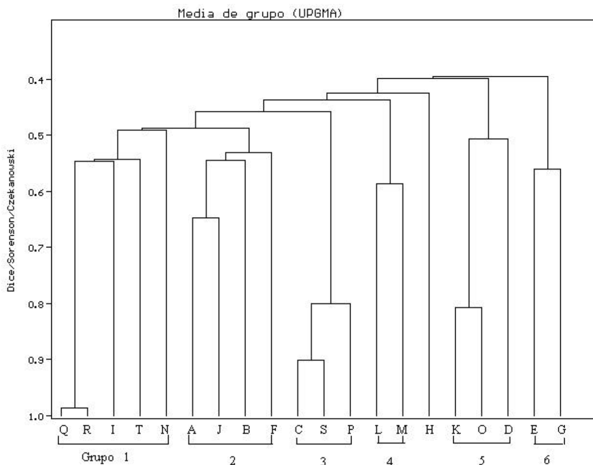
FIGURA 4 – Dendrograma da análise de agrupamentos por médias não ponderadas (UPGMA) das similaridades florísticas (Sørensen) entre 20 remanescentes florestais do município de Viçosa-MG. A = UFV (Lopes et al., 2002); B = Mata da Silvicultura - UFV (Meira-Neto & Martins, 2000); C = Mata da Biologia - UFV (Paula et al., 2002); D = Mata da Pedreira (Marangon et al., 2003); E = Fazenda Bom Sucesso (Irsigler, 2002); F = Mata do Juquinha (Silva et al., 2004); G = Fazenda Bom Sucesso (Campos, 2002); H = Fazenda Tico-Tico (Soares Júnior, 2000); I = Fazenda Rancho Fundo (Senra, 2000); J = Fazenda São Geraldo (Silva et al., 2003a); K = Mata do Paraíso (Silva, 2003); L = Área 1 (Almeida Júnior, 1999); M = Área 4 (Almeida Júnior, 1999); N = Sítio Palmital (Ribas et al., 2003); O = Mata do Paraíso (Fernandes, 1998); P = Mata da Biologia - UFV (Silva et al., 2000); Q = Mata da Garagem (Silva et al., 2003b); R = Mata da Garagem (Silva et al., 2002); S = Mata da Biologia (Gasparini-Júnior, 2004); T = Mata da Agronomia (Presente estudo).
