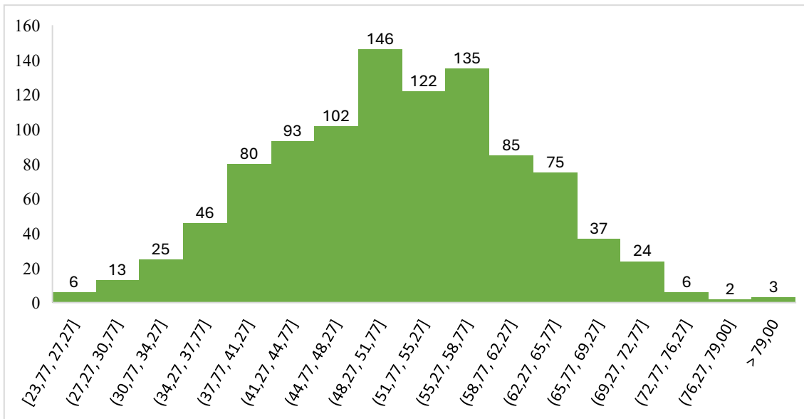
Figura 15 - Histograma de frequência para variável produtividade \text{m}^3/\text{hora} do forwarder
