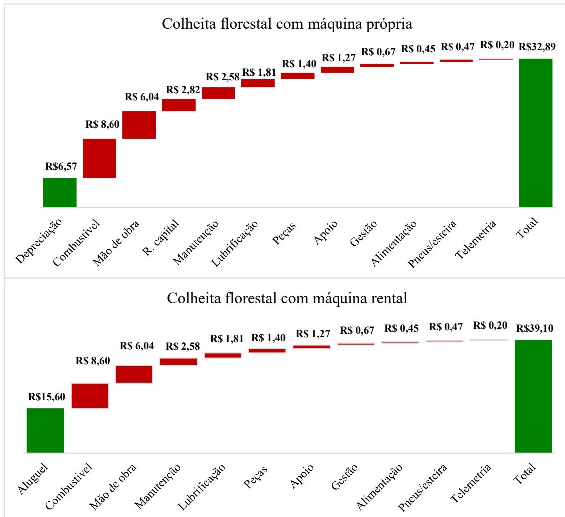
Figura 4 - Custos da colheita florestal R$/m 3 na modalidade de máquinas própria e rental
