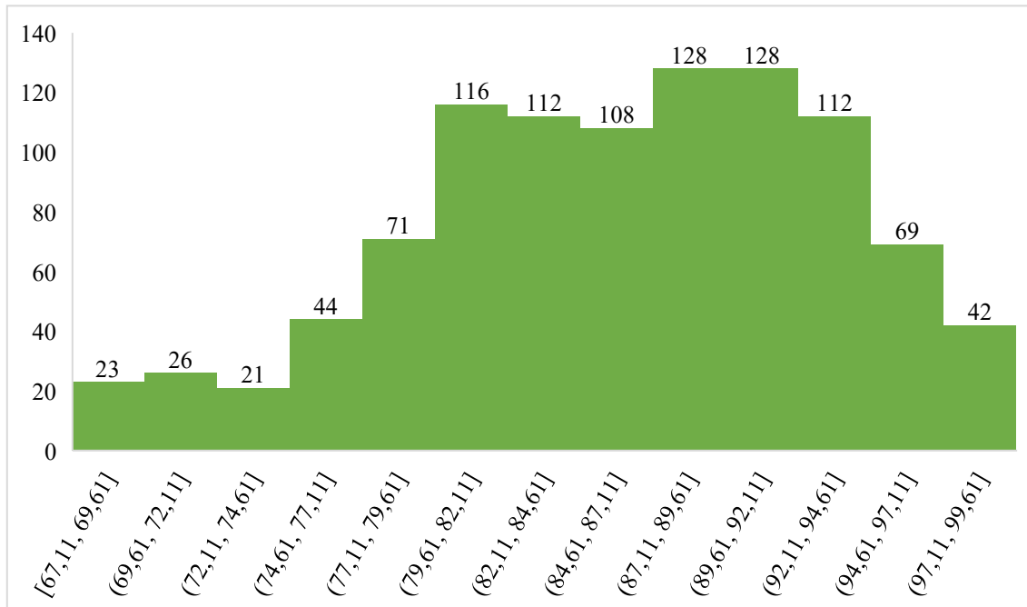
Figura 10 - Histograma de frequência para a disponibilidade mecânica (%) do corte com harvester
