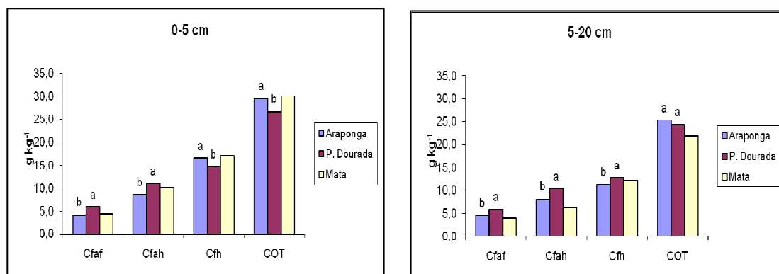
Figura 1: Teor de Carbono Orgânico Total (COT) e na fração húmica (Cfh), ácidos fúlvicos (Cfaf) e ácidos húmicos (Cfah) nas profundidades de 0-5 e 5-20 cm no municípios de Araçuaia e Pedra Dourada na Zona da Mata Mineira.
