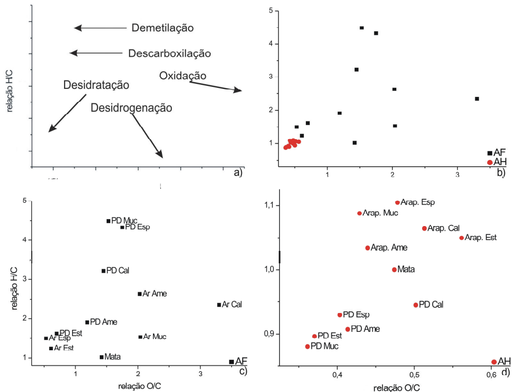
Figura 1: Diagrama de van Krevelen nos AF e AH de solos sob cafezal em Araponga (Ar), Pedra Dourada (PD) e solo sob mata. a) Principais reações envolvidas nos processos de humificação (adaptado de RICE e MACCARTHY, 1991); b) Diagrama com AF e AH juntos; c) Diagrama AF; d) Diagrama AH; Ame: amendoim; Cal: calopogônio; Est:estilosantes; Muc: mucuna; Esp: espontâneas.
