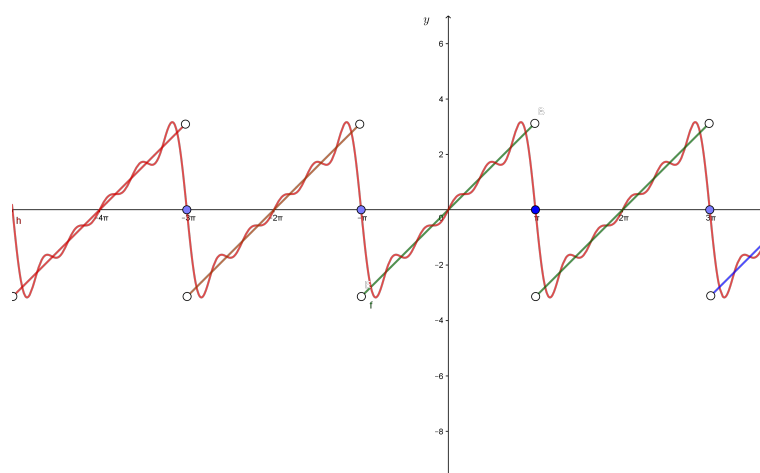
Figura 5.2: Série de fourier de f(x) calculada até n = 5
