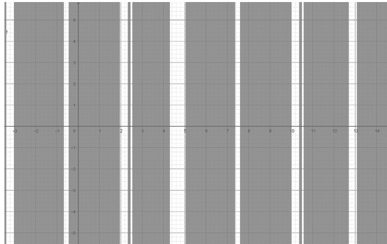
Figura 6.2: Gráfico da função série da nota Mi_5
