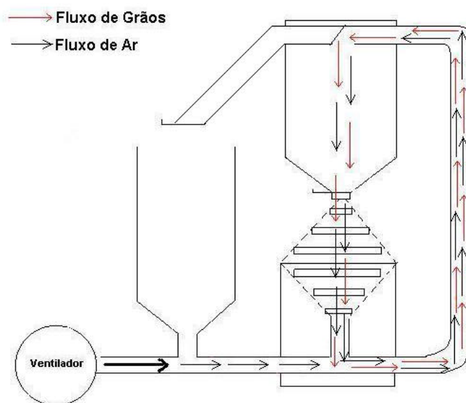
Figura 9- Fluxo de ar e movimentação dos grãos no abastecimento do secador
