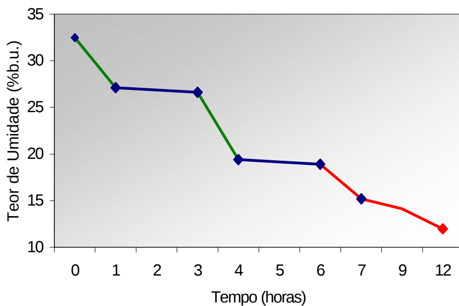
Figura 30- Curva de secagem para o café descascado com movimentação dos grãos a cada uma hora (teste 5).
