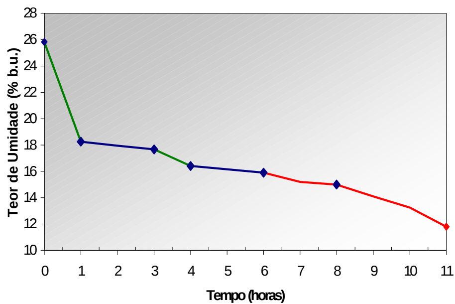
Figura 26 - Curva de secagem para o café natural com movimentação dos grãos a cada uma hora (teste 1).
