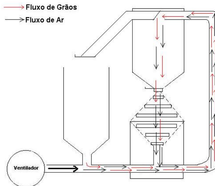
Figura 7- Fluxo de ar e grãos no abastecimento do secador.
