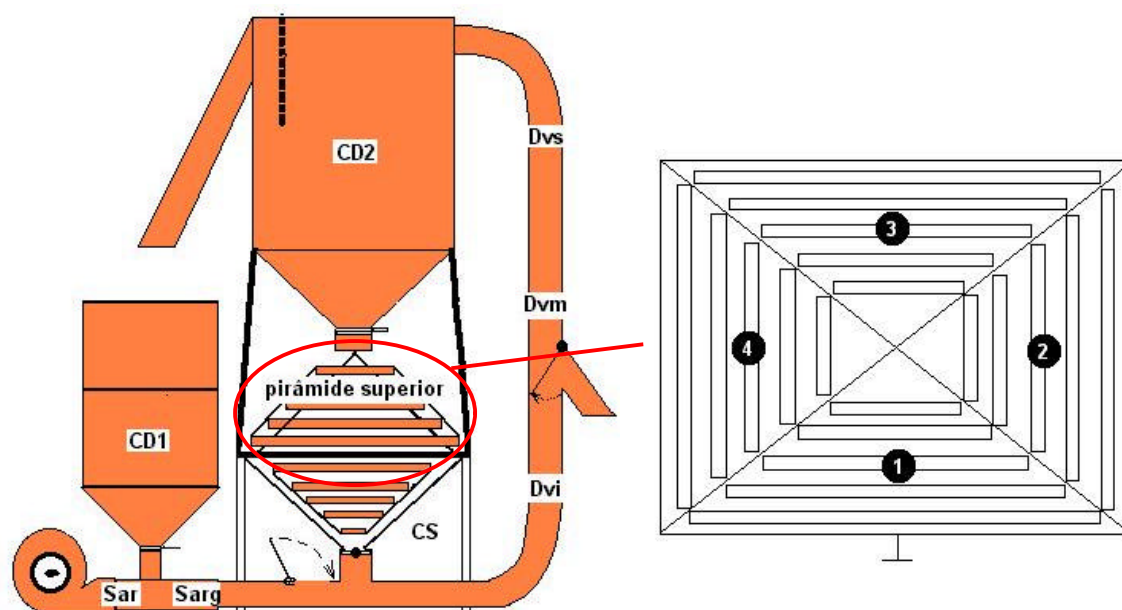
Figura 14 - Detalhes do posicionamento dos sensores de temperatura na massa de grãos (Temperatura na massa de grãos – superior 1 / superior 2 / superior 3 / superior 4).
