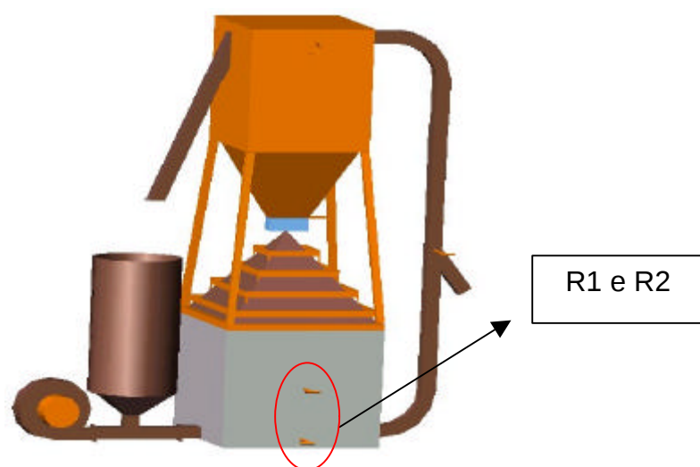
Figura 5 - Vista lateral do secador pneumático e do posicionamento dos registros para direcionamento do fluxo de ar para secagem ou movimentação dos grãos.
