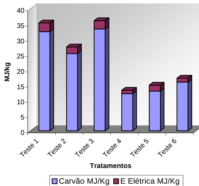
Figura 32 - Consumo específico de energia elétrica e de combustível (carvão).
