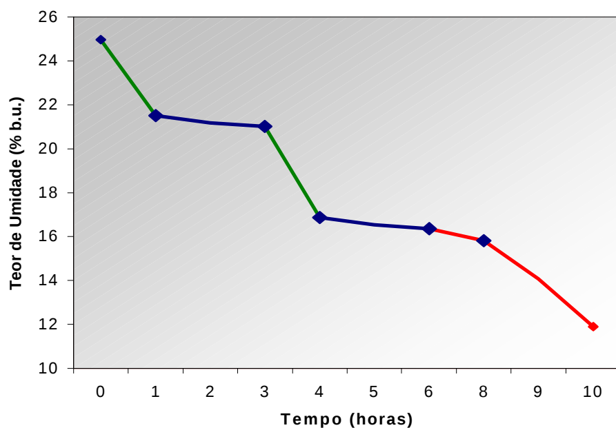
Figura 27- Curva de secagem para o café natural com movimentação dos grãos a cada uma hora (teste 2).
