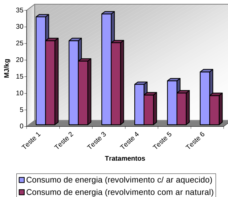
Figura 33 - Comparação do consumo específico de energia elétrica e de combustível (carvão), fazendo-se a movimentação do produto com ar aquecido e natural.
