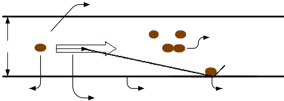
Figura 2- Causas da fricção durante o transporte pneumático.
