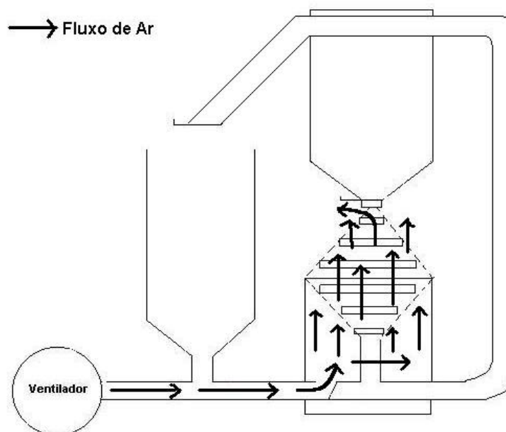
Figura 8 - Fluxo de ar durante a secagem.
