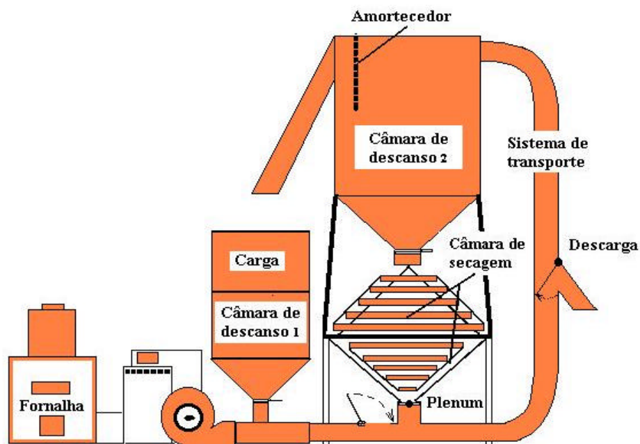
Figura 3 - Secador de café com sistema de transporte pneumático.
