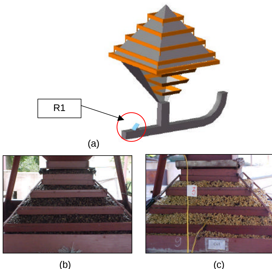
Figura 4 – (a) Detalhe do formato da câmara de secagem e do registro do direcionamento do fluxo de ar para secagem ou movimentação; (b) detalhe da câmara de secagem com café natural; (c) café cereja descascado.
