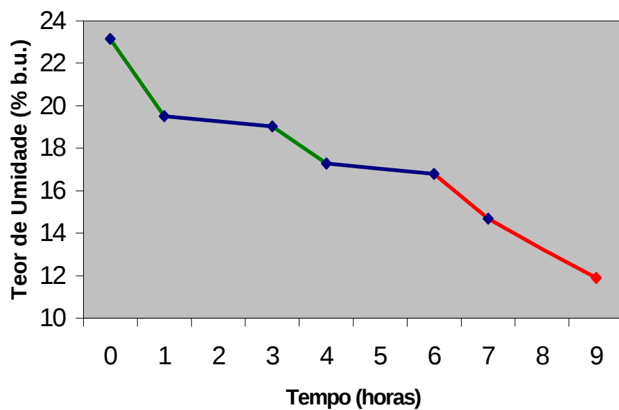
Figura 28 - Curva de secagem para o café natural com movimentação dos grãos a cada uma hora (teste 3).
