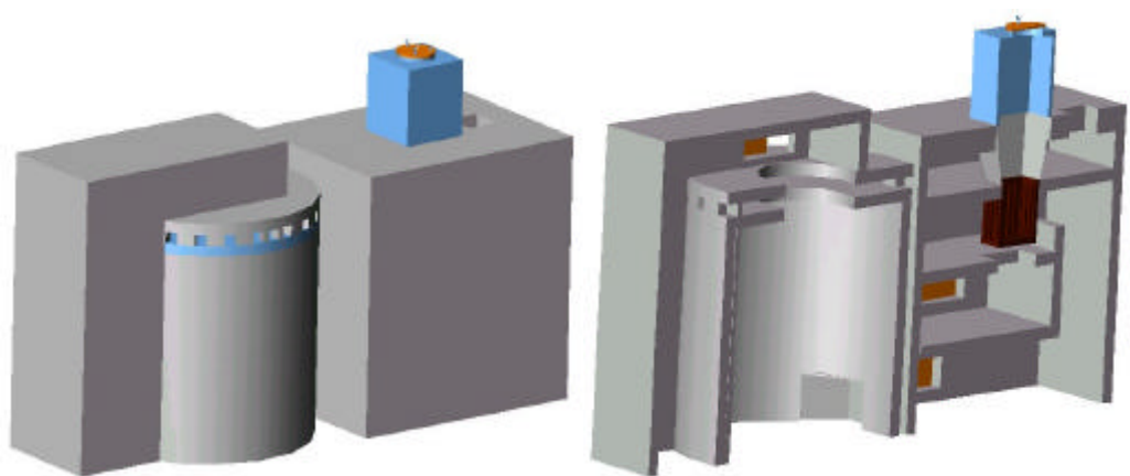
Figura 13 - Vista geral e corte longitudinal da fornalha a carvão vegetal e do ciclone.
