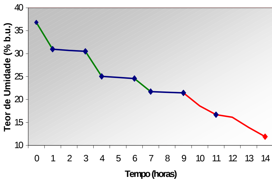
Figura 29 - Curva de secagem para o café descascado com movimentação dos grãos a cada uma hora (teste 4).
