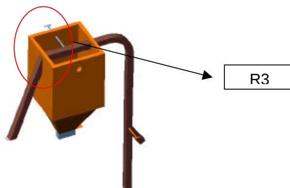
Figura 6 - Vista da câmara de descanso 2 e do registro para direcionamento do fluxo de grãos para câmara de secagem ou movimentação dos grãos.
