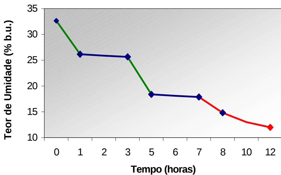
Figura 31- Curva de secagem para o café descascado com movimentação dos grãos a cada uma hora (teste 6).
