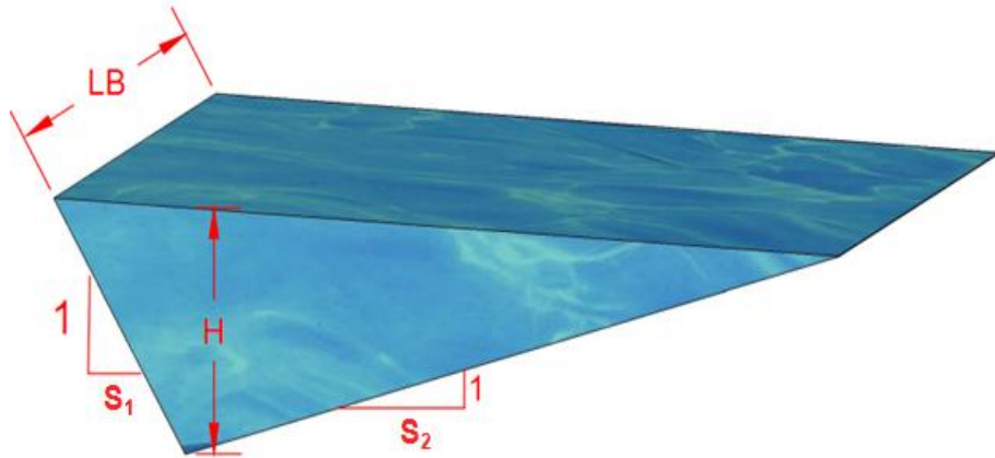
Figura 9 - Bacia de infiltração retangular com seção transversal triangular.
