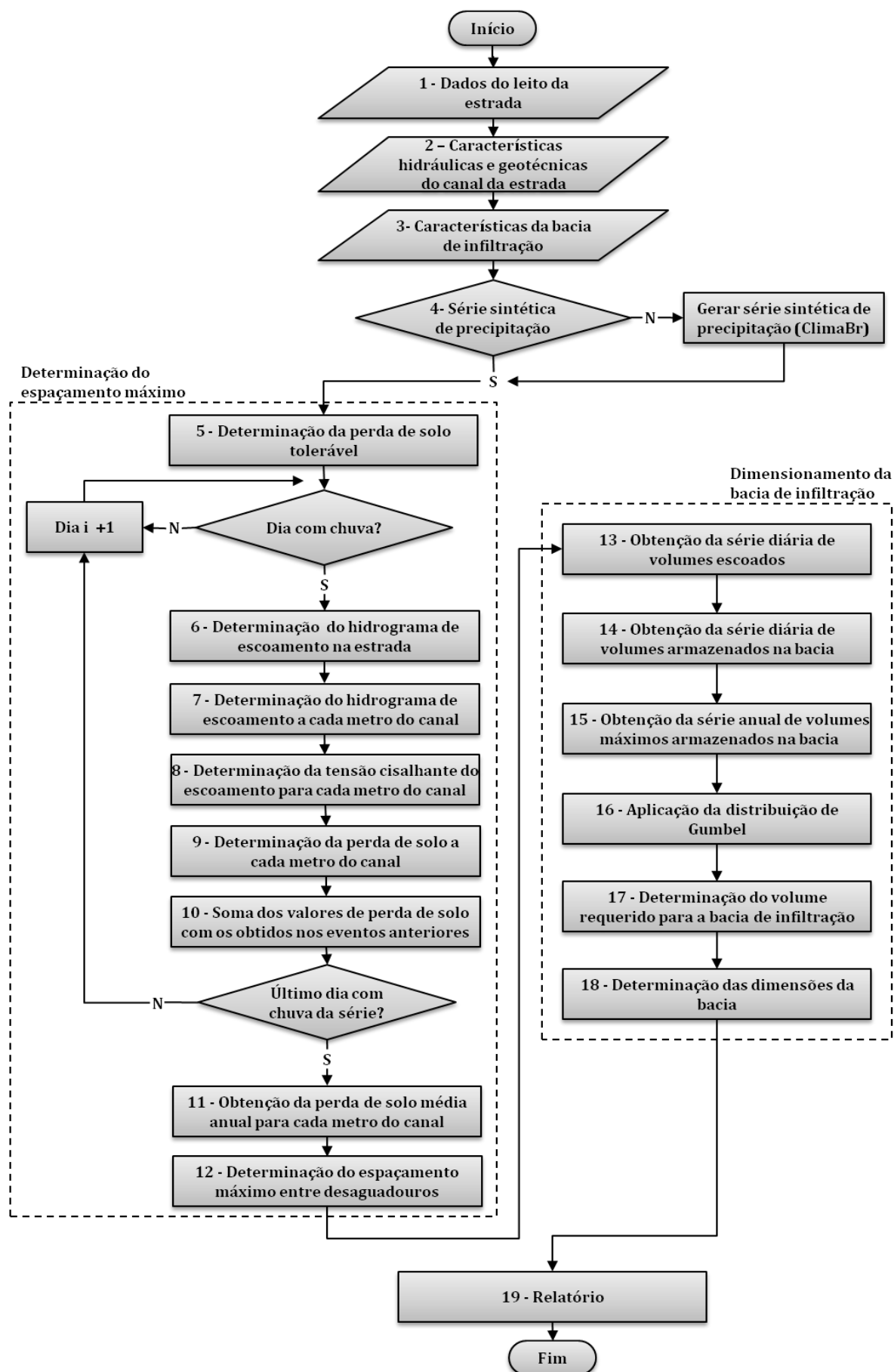
Figura 15 - Fluxograma simplificado do algoritmo para a aplicação do modelo.
