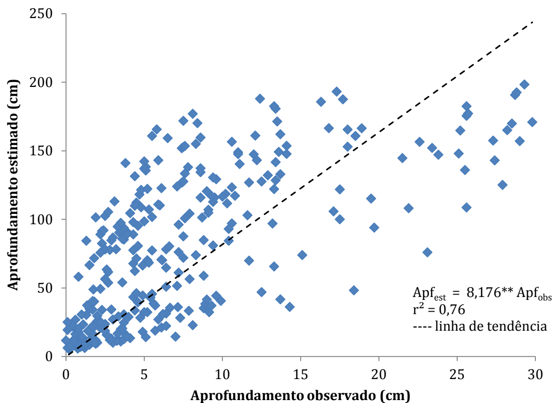
Figura 33 - Dados de aprofundamento estimados pelo modelo versus os observados em campo obtidos ao longo do canal e em diferentes datas, sendo os valores estimados obtidos com o modelo, considerando-se o cálculo da tensão cisalhante realizado por meio da equação da resistência ao cisalhamento utilizando a profundidade de escoamento ( y ) (equação 11).
