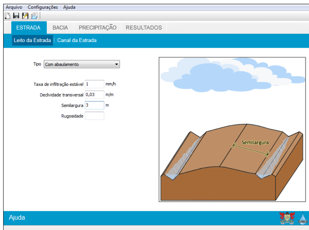
Figura 22 – Telas para orientar o preenchimento dos valores das variáveis taxa de infiltração estável (A), semilargura (B).
