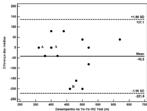
Figura 3 – Plotagem do viés (média das diferenças) e limites de concordância ( \pm 1,96 IC95%) entre os desempenhos obtidos no teste de Yo-Yo Intermitente Recovery Test Level 2 (Yo-Yo IR2), de acordo com os procedimentos de Bland-Altman (N=18). Nota: “A” representa sobreposição de três jogadores e “B” dois jogadores.
