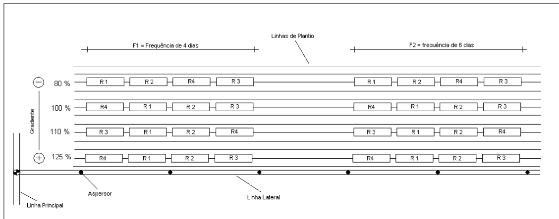
Figura 1 - Detalhes gerais do experimento de irrigação por aspersão convencional na cultura da batata na região de São Gonçalo do Sapucaí - MG, 2007.
