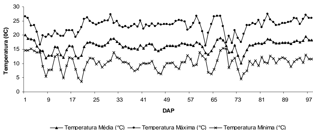
Figura 4 - Temperatura máxima, média e mínima ao longo do ciclo da cultura. Fazenda São Geraldo - São Gonçalo do Sapucaí - MG, 2007.
