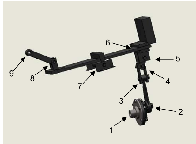
Figura 3.2 – Representação das articulações
