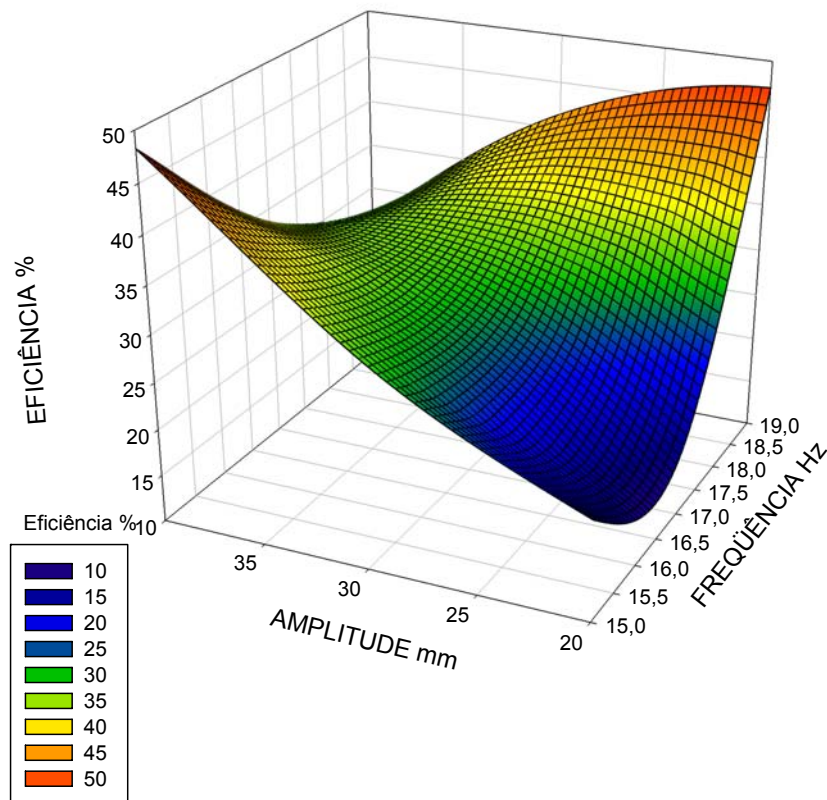
Figura 4.7 - Superfície de resposta da eficiência de derrifa do café verde
