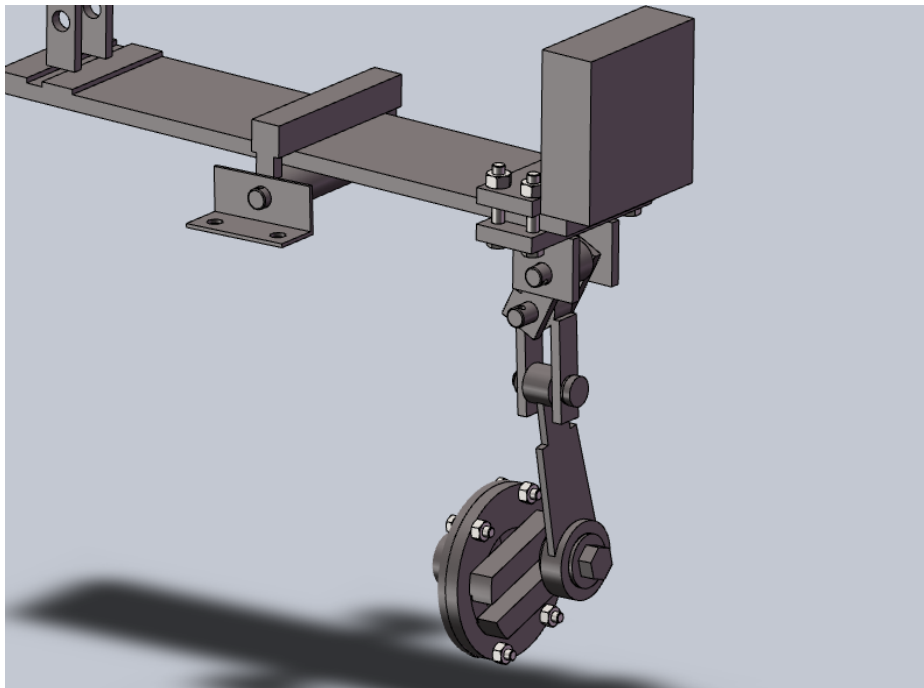
Figura 2.6 - Desenho das articulações do protótipo dispositivo de derrixa.
