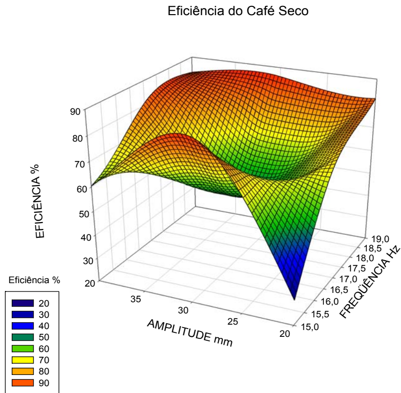
Figura 4.9 - Superfície de resposta da eficiência de derriza do café seco.
