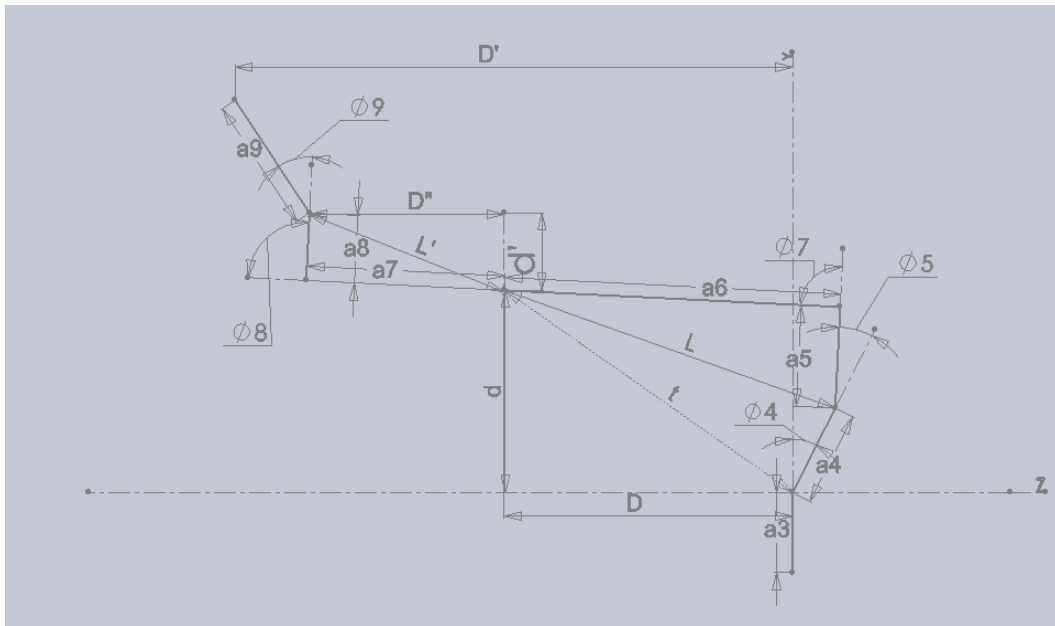
Figura 3.5 - Croqui das articulações no plano ZY.
