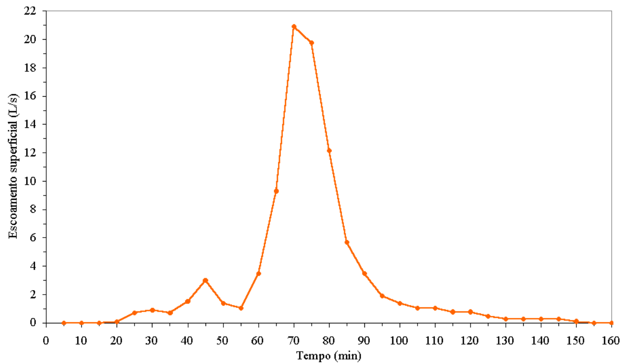
Figura 37 - Hidrograma de escoamento superficial ocorrido no dia 02/02/2002.
