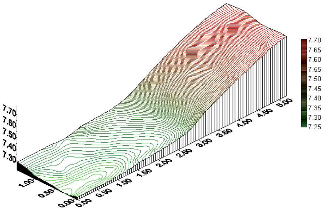
Figura 30 - Representação do fundo do canal construído na seção de desagüe para concentração e condução do escoamento superficial.
