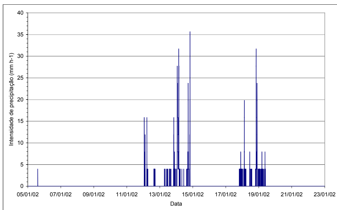
Figura 4C – Precipitações ocorridas na bacia hidrográfica entre os dias 04/01/2002 e 22/01/2002.
