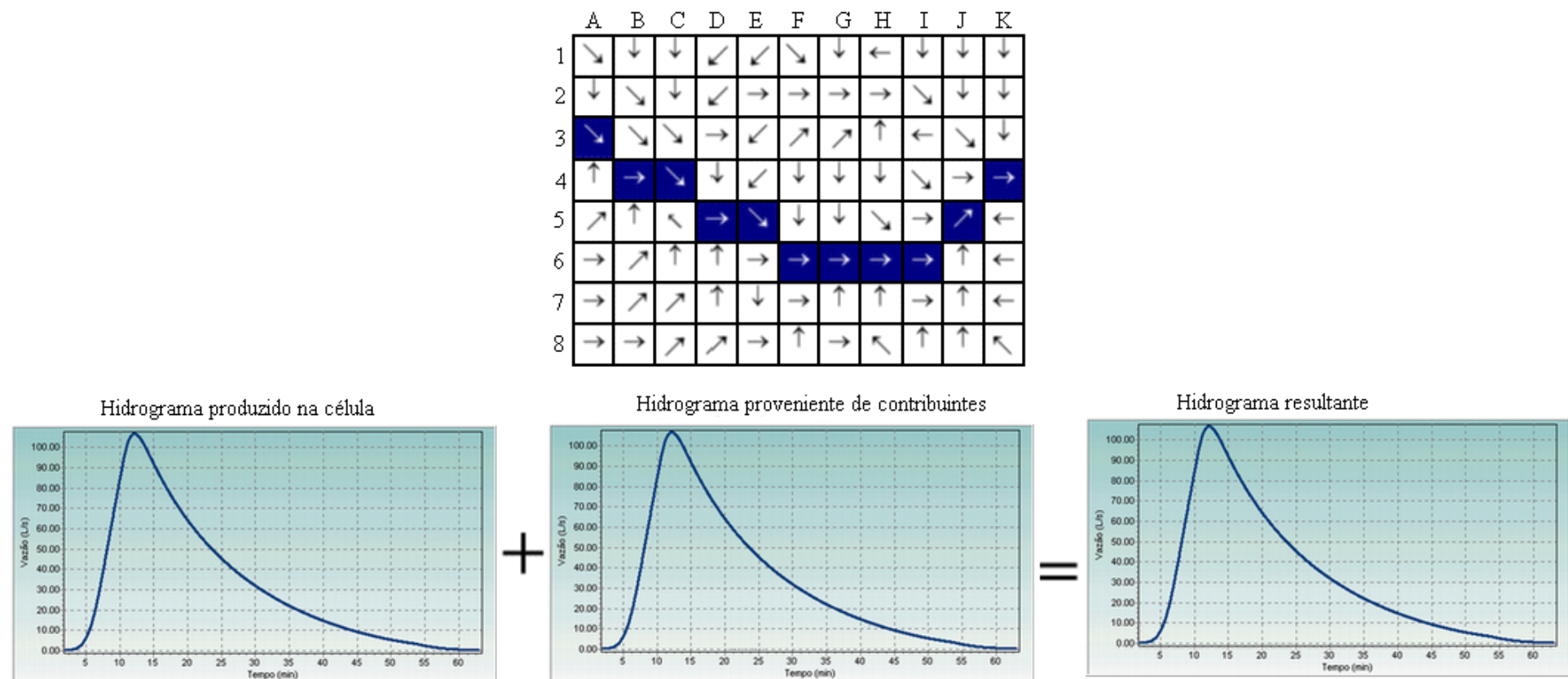
Figura 12 - Representação esquemática do processo de soma dos hidrogramas para a obtenção do hidrograma resultante em uma célula.
