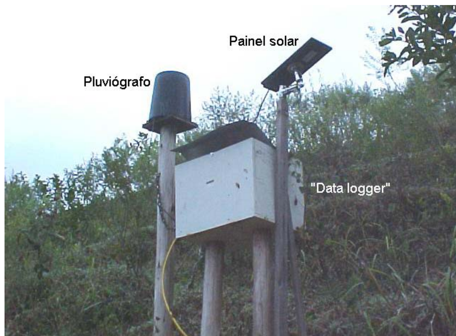
Figura 28 - Foto representativa do “data logger” e do pluviôgrafo instalados na estação de monitoramento.
