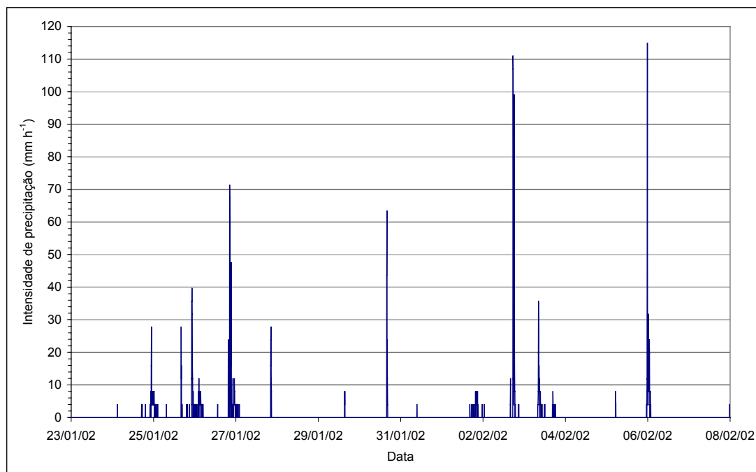
Figura 5C – Precipitações ocorridas na bacia hidrográfica entre os dias 22/01/2002 e 07/02/2002.
