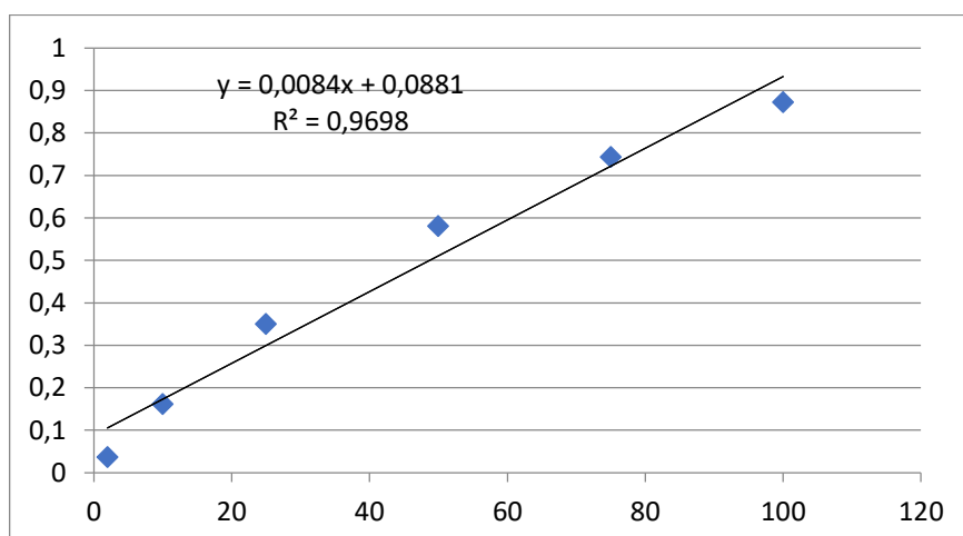
Figura 1: Curva de calibração de \text{Li}^+ .
