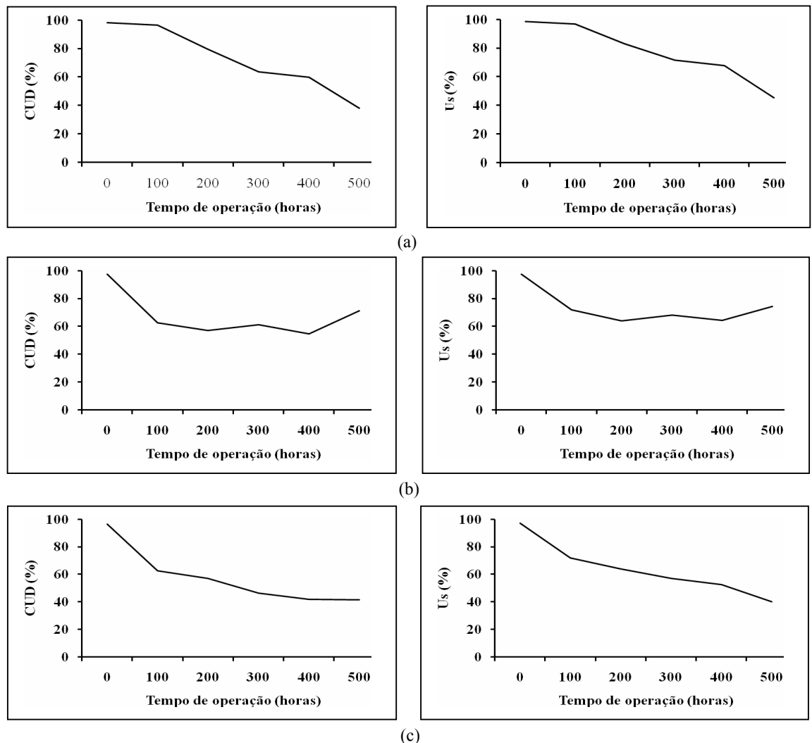
Figura 3. Variação dos valores de coeficientes de uniformidade CUD e U_s , em função dos tempos de operação para aplica-
