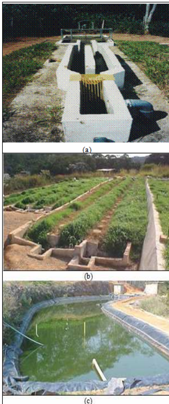
Figura 1. Tratamento preliminar (a), tratamento secundário (b) e tratamento terciário (c) do esgoto doméstico na Unidade Piloto de Tratamento de Água Residuária e Agricultura Irrigada (UTAR) do DEA/UFV, em Viçosa-MG.
