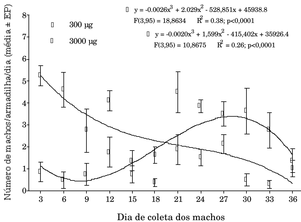
Figura 3 – Captura de machos de Leucoptera coffeella , com feromônio sexual, 5,9-dimetilpentadecano, na forma racêmica, impregnado em septos de borracha. Viçosa, MG.
