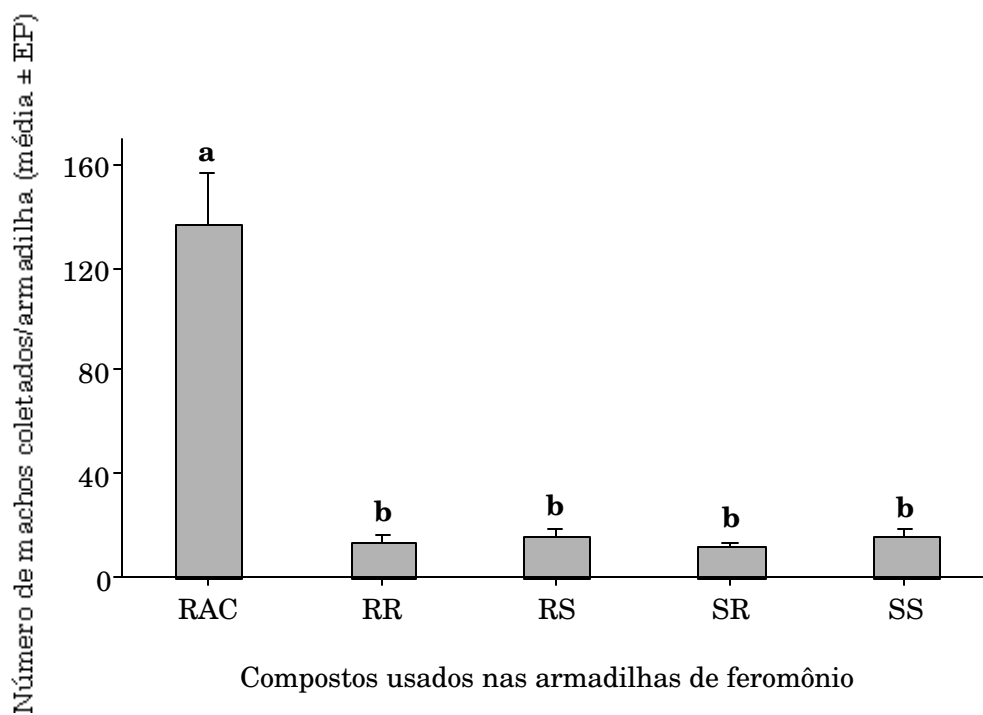
Figura 4 – Coleta de machos de Leucoptera coffeella em armadilhas de feromônio impregnadas com a mistura racêmica e isômeros do 5,9-dimetilpentadecano. Patrocínio, MG. Tratamentos seguidos da mesma letra não diferem estatisticamente (ANOVA seguido de Duncan; p < 0,05 ).
