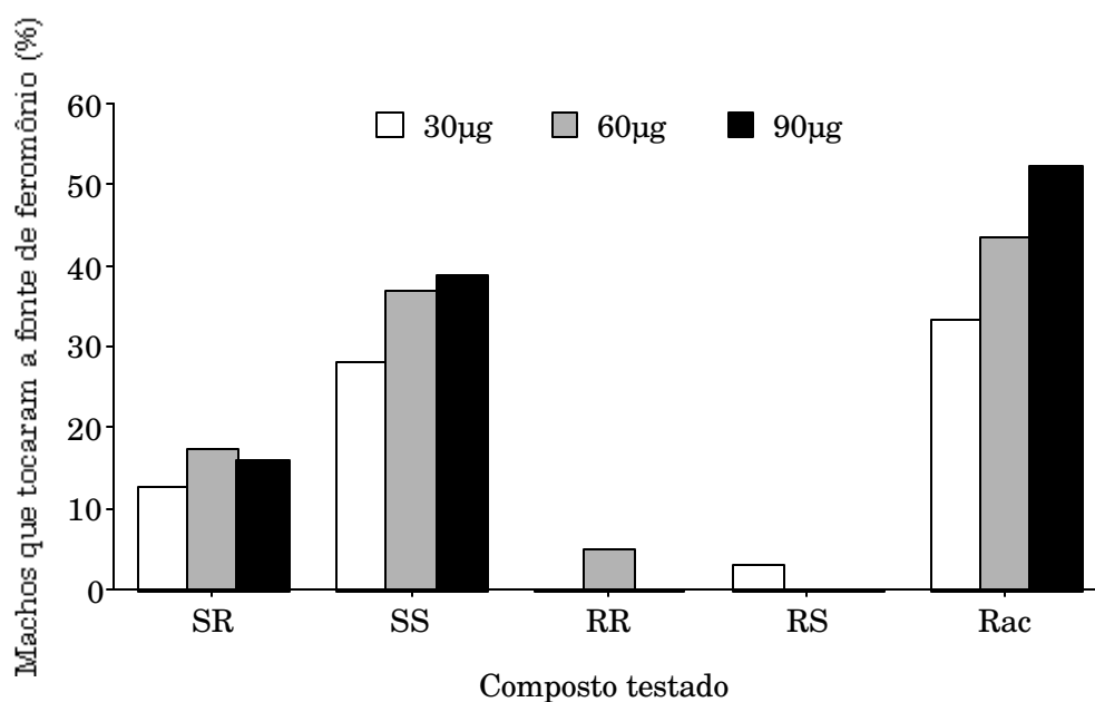
Figura 3 – Porcentagem de machos de Leucoptera coffeella que tocaram a fonte de feromônio quando testados em túnel-de-vento. SR, SS, RR, RS e Rac representam os isômeros possíveis isômeros do 5,9-dimetilpentadecano e a mistura racêmica, respectivamente em tres doses.
