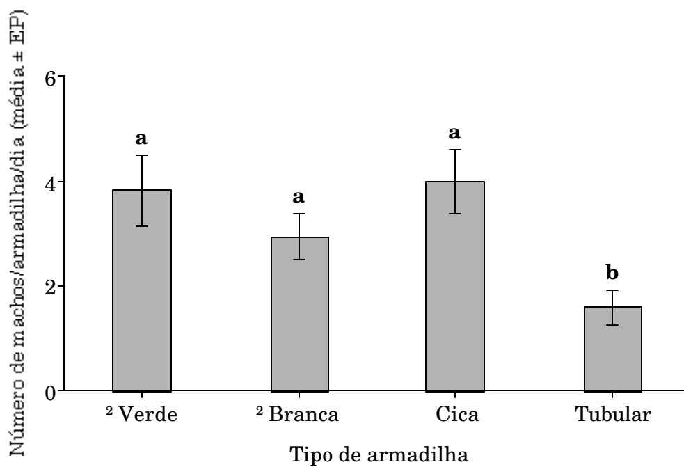
Figura 5 – Captura de machos de Leucoptera coffeella , com feromônio sexual, 5,9-dimetilpentadecano, na forma racêmica, impregnado em septos de borracha. Manhuaçu, MG. Tratamentos seguidos da mesma letra não diferem estatisticamente (ANOVA seguido de Tukey; p < 0,05 ).
