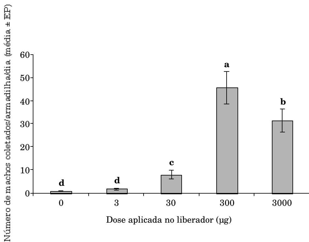
Figura 2 – Captura de machos de Leucoptera coffeella , com feromônio sexual, 5,9-dimetilpentadecano, na forma racêmica, impregnado em septos de borracha. Viçosa, MG. Tratamentos seguidos da mesma letra não diferem estatisticamente (ANOVA seguido de Tukey; p > 0,05 ).
