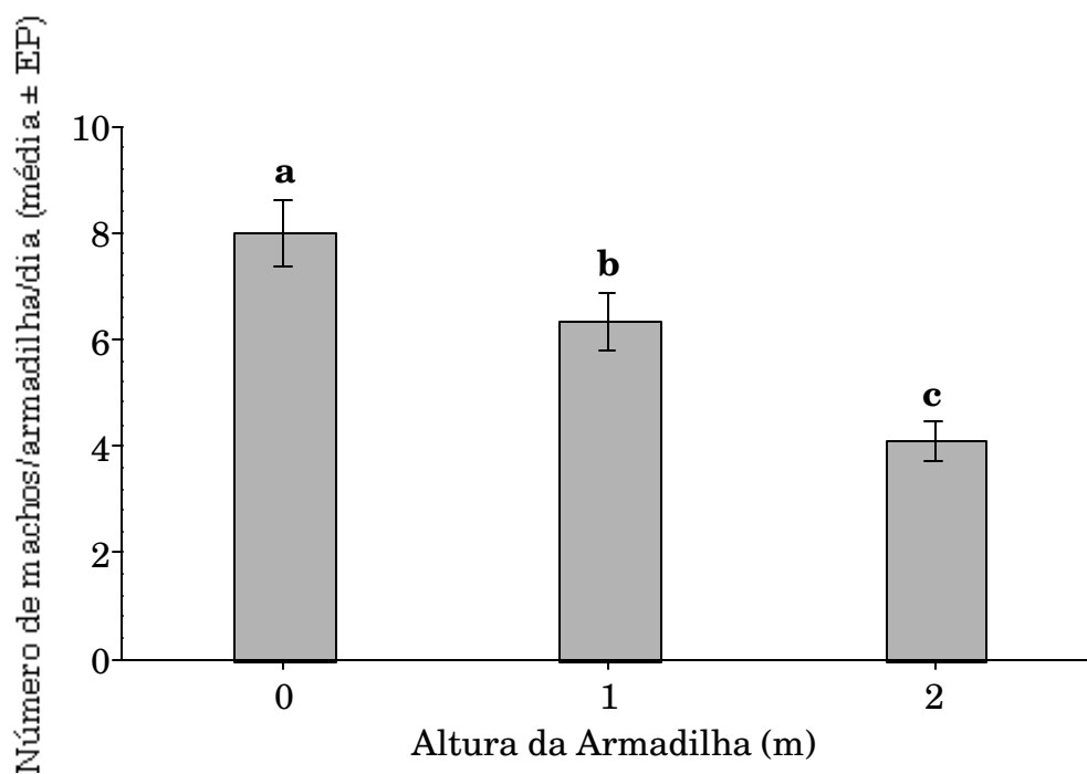
Figura 6 – Captura de machos de Leucoptera coffeella , com feromônio sexual, 5,9-dimetilpentadecano, na forma racêmica, impregnado em septos de borracha. Manhuaçu, MG. Os histogramas seguidos pela mesma letra não diferem, entre si, pelo teste Tukey ( p > 0,05 ).
