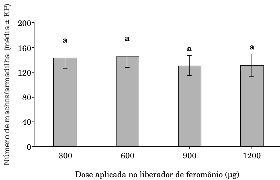
Figura 4 – Captura de machos de Leucoptera coffeella , com feromônio sexual, 5,9-dimetilpentadecano, na forma racêmica, impregnado em septos de borracha. Patrocínio, MG. Tratamentos seguidos da mesma letra não diferem estatisticamente (ANOVA seguido de Tukey; p > 0,05 ).
