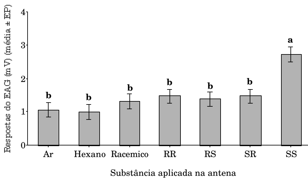
Figura 1 – Eletroantenogramas em de machos de Leucoptera coffeella aos compostos 5,9-dimetilpentadecano na forma racêmica e seus respectivos isômeros. Tratamentos seguidos da mesma letra não são estatisticamente diferentes. (ANOVA seguido de Duncan) p < 0,05 (n=15).
