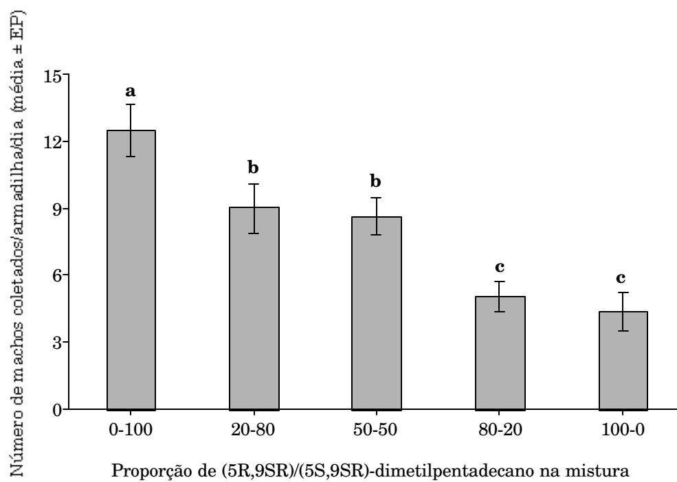
Figura 2 – Machos de Leucoptera coffeella coletados em armadilhas tipo Delta contendo diferentes proporções dos isômeros parciais do 5,9-dimetilpentadecano. Patrocínio, MG.
