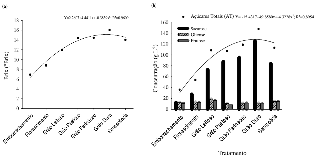
Figura 8. (a) Concentração de açúcares (em graus Brix- °Brix) e (b) Participação, em g L -1 , de sacarose, glicose e frutose na concentração de açúcares totais (AT) no caldo do sorgo sacarino BRS 511 ao longo dos estádios fenológicos.
