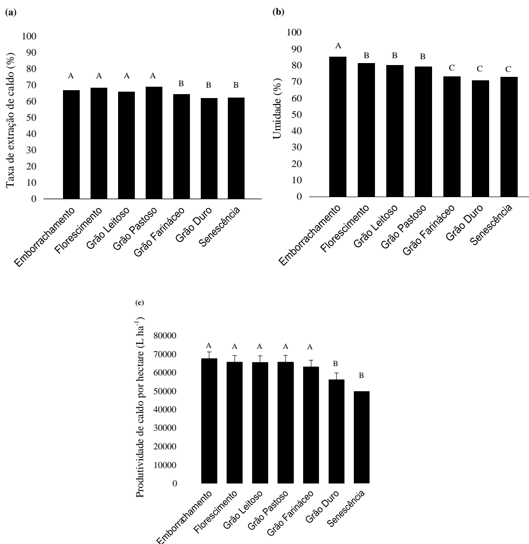
Figura 7. (a) Taxa de extração de caldo do colmo (TE); (b) Percentual de umidade do colmo (c) Produtividade de caldo por hectare (PCH), em L ha -1 , do caldo extraído do colmo de sorgo sacarino BRS 511 ao longo dos estádios fenológicos. Médias (em barras) seguidas pela mesma letra não diferem significativamente entre si, ao nível de 5% de probabilidade, pelo teste Scott-Knott.
