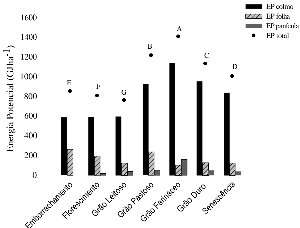
Figura 9: Energia potencial total (EP total), da folha (EP folha), do colmo (EP colmo) e da panícula (EP panícula) ao longo dos estádios fenológicos do sorgo biomassa BRS 716.
