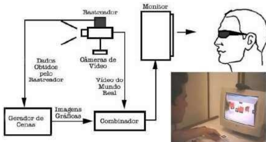
Figura 7: Sistema de visão por vídeo baseada em monitor.
