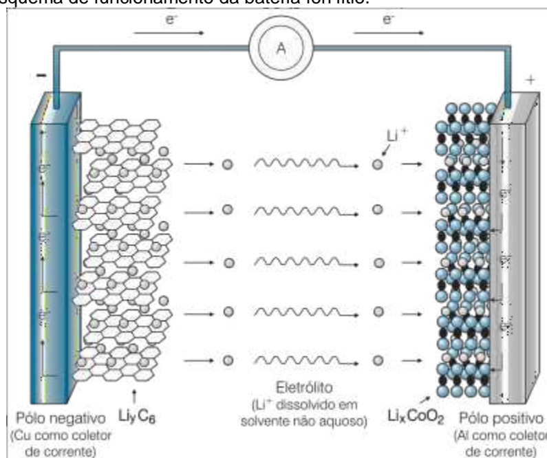
Figura 35: Esquema de funcionamento da bateria íon lítio.
