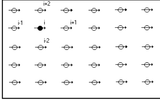
Figura 2.3: Rede quadrada 2D ferromagnética com interação entre primeiros vizinhos.
