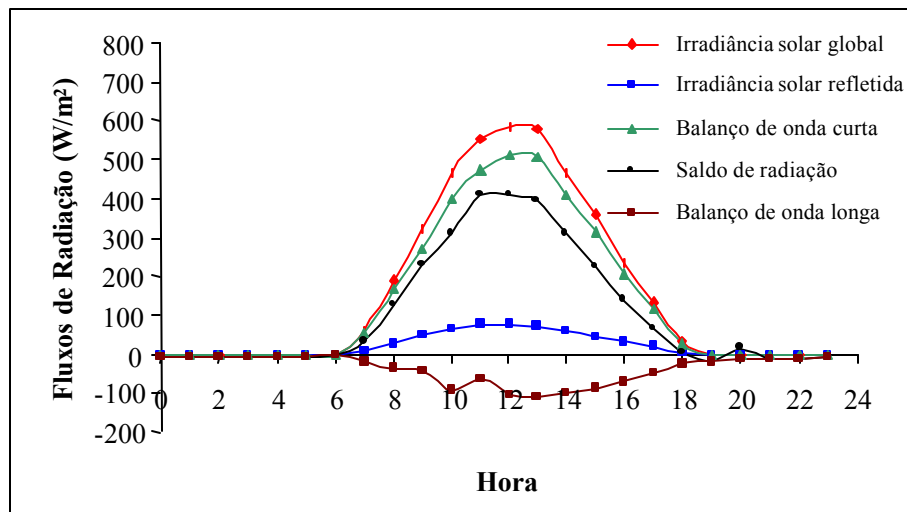
Figura 8 - Balanço de radiação médio horário em dezembro de 1995
