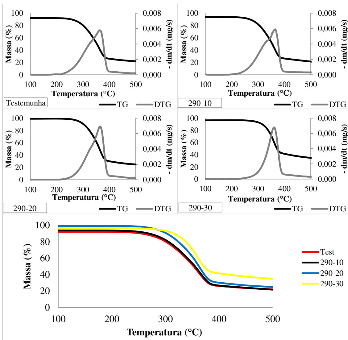
Figura 5 – Curvas de TG (massa) e DTG ( - dm/dt ) para a testemunha e pellets torreficados a 290 °C nos tempos 10, 20 e 30 minutos (Atmosfera de nitrogênio, taxa de aquecimento 10 °C/min e amostras a 0% de umidade)
