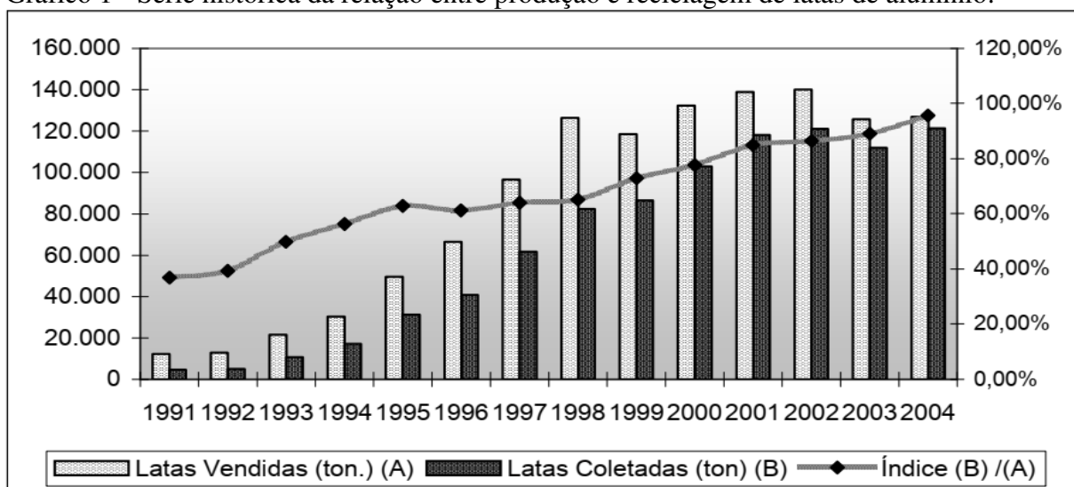
Gráfico 1 - Série histórica da relação entre produção e reciclagem de latas de alumínio.
