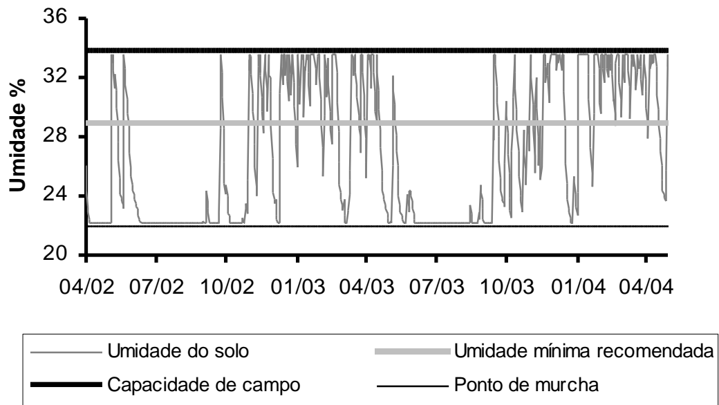
Figura 11 – Curva de evolução da umidade do solo para T1.
