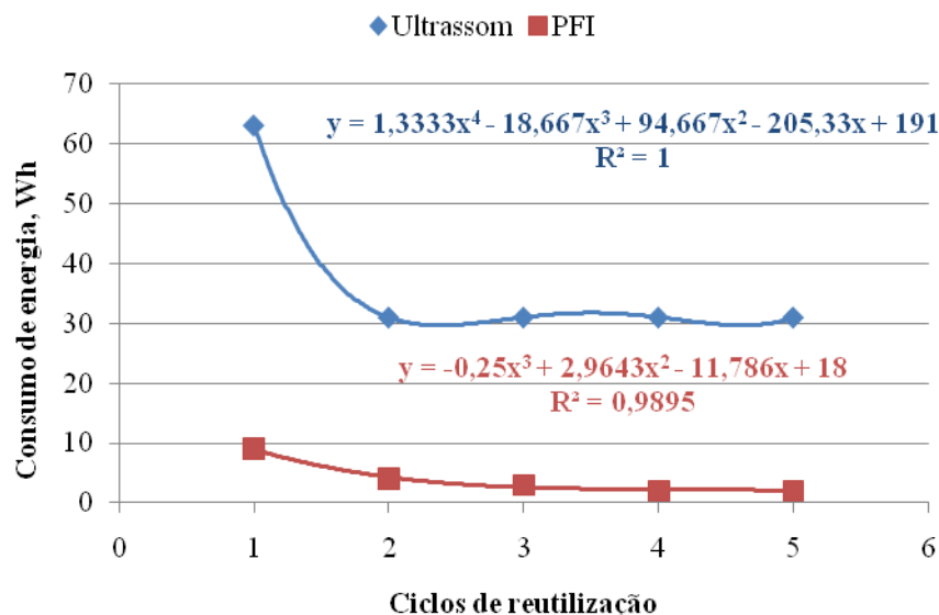
Figura 12. Consumo de energia para o refino convencional e tratamento ultrassônico ao longo dos 5 ciclos de reciclagem da polpa.
