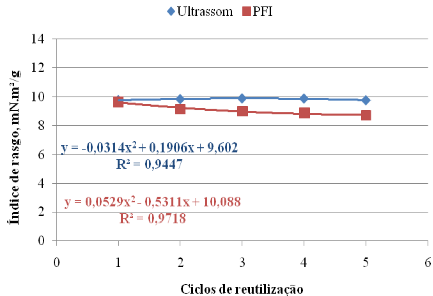
Figura 13. Índice de rasgo das polpas submetidas ao refino convencional e tratamento ultrassônico ao longo dos 5 ciclos de reciclagem da polpa.
