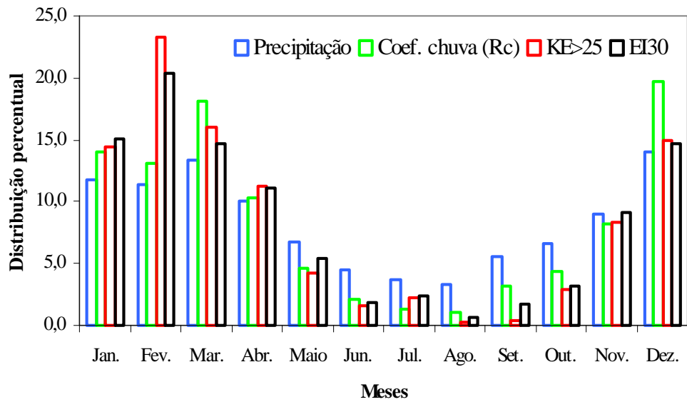
Figura 10 – Distribuição percentual mensal de precipitação, dos índices de erosividade e do coeficiente de chuva na Estação Tanguá.
