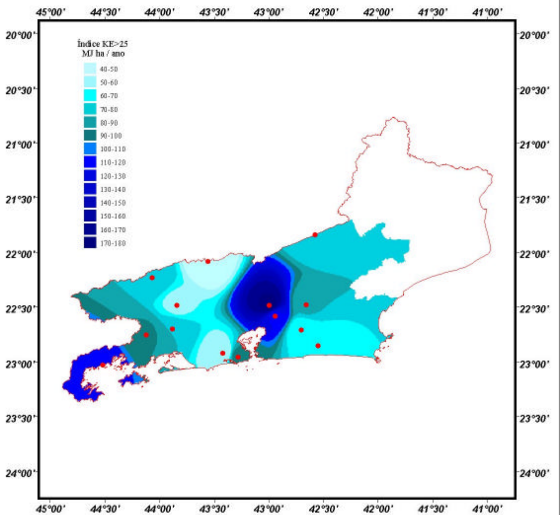
Figura 18 – Mapa de isocorrosividade do Estado do Rio de Janeiro, obtido por meio de interpolação do índice de erosividade KE>25.
