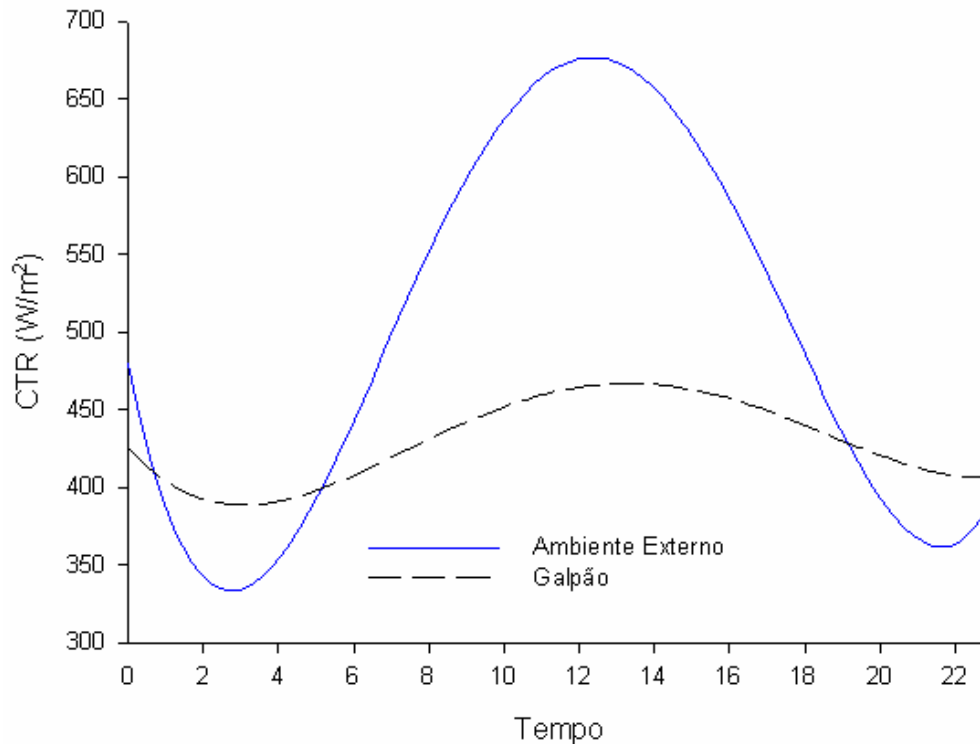
FIGURA 13 – Estimativas da carga térmica radiante (CTR), para o interior do galpão onde estavam alojadas as emas e para o ambiente externo, em função das observações horárias
