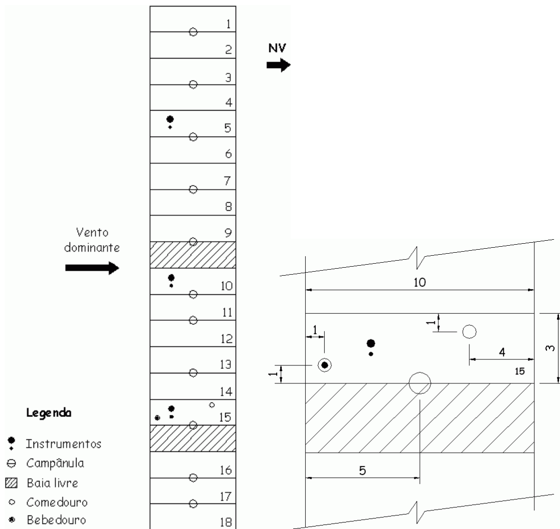
FIGURA 01 - Esquema da divisão do galpão (sem escalas, dimensões em m) utilizado no experimento, com detalhes da disposição dos conjuntos de instrumentos de medida de variáveis ambientais
