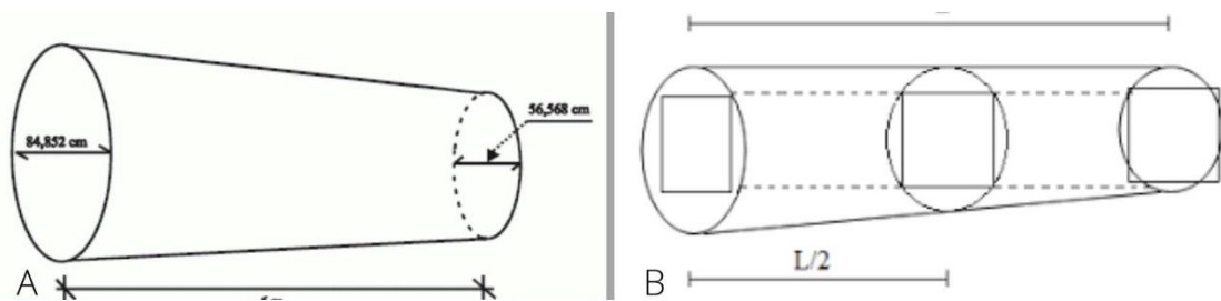
Figura 2-A. Metodologia utilizada para o cálculo do volume geométrico em tora. Figura 2-B. Metodologia utilizada para o cálculo do volume francon. Fonte: Universidade Federal do Espírito Santo (UFES). Elaboração: Autor.
