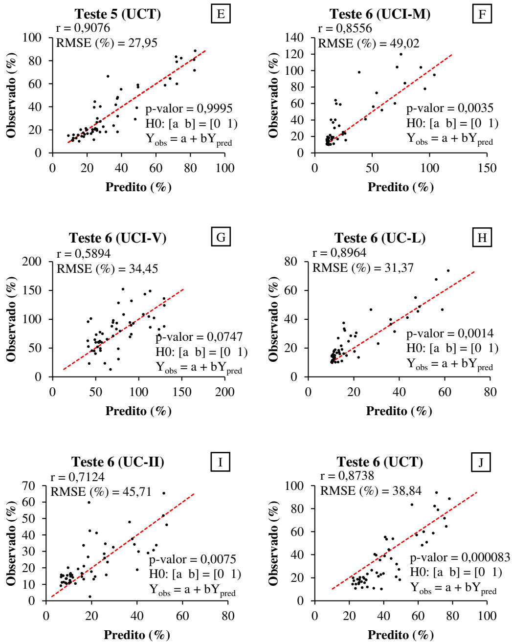
Figura 4 - As variáveis de saída do teste de umidade do material combustível preditas e observadas. Os valores de p-valor do teste F aplicado para avaliar H_0: [a \ b] = [0 \ 1] , sendo Y_{obs} = a + bY_{pred} (Continuação)
