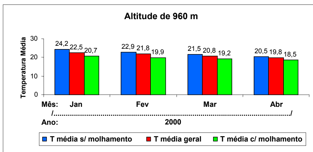
Figura 7- Temperatura média nos meses de janeiro, fevereiro, março e abril de 2000, na altitude de 960 m, nas horas de molhamento foliar, nas horas sem molhamento foliar e nas horas independentes de molhamento foliar, na Zona da Mata de Minas Gerais.
