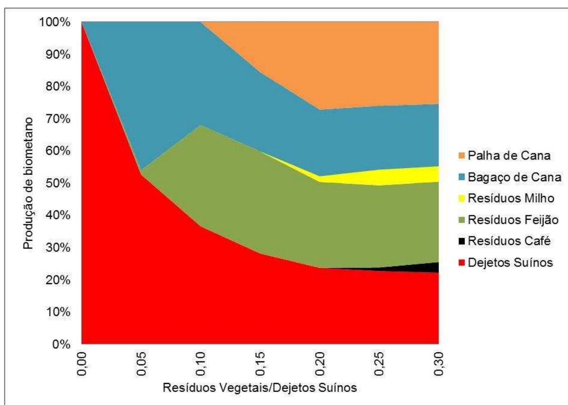
Figura 6.11 – Produção de metano por substrato para uma granja com 2.500 suínos no município de Muriaé.
