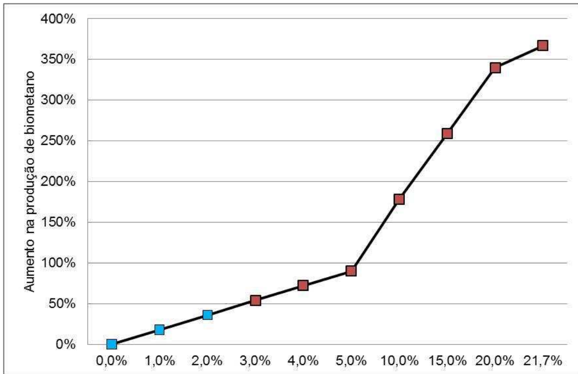
Figura 4.19 – Aumento na produção de biometano com a codigestão.
