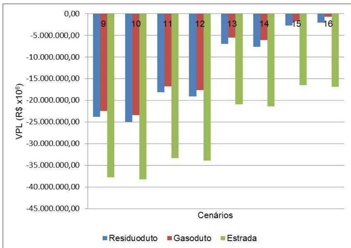
Figura 7.28 – VPL para os cenários de codigestão com 1,5% de razão resíduos vegetais/dejetos suínos.
