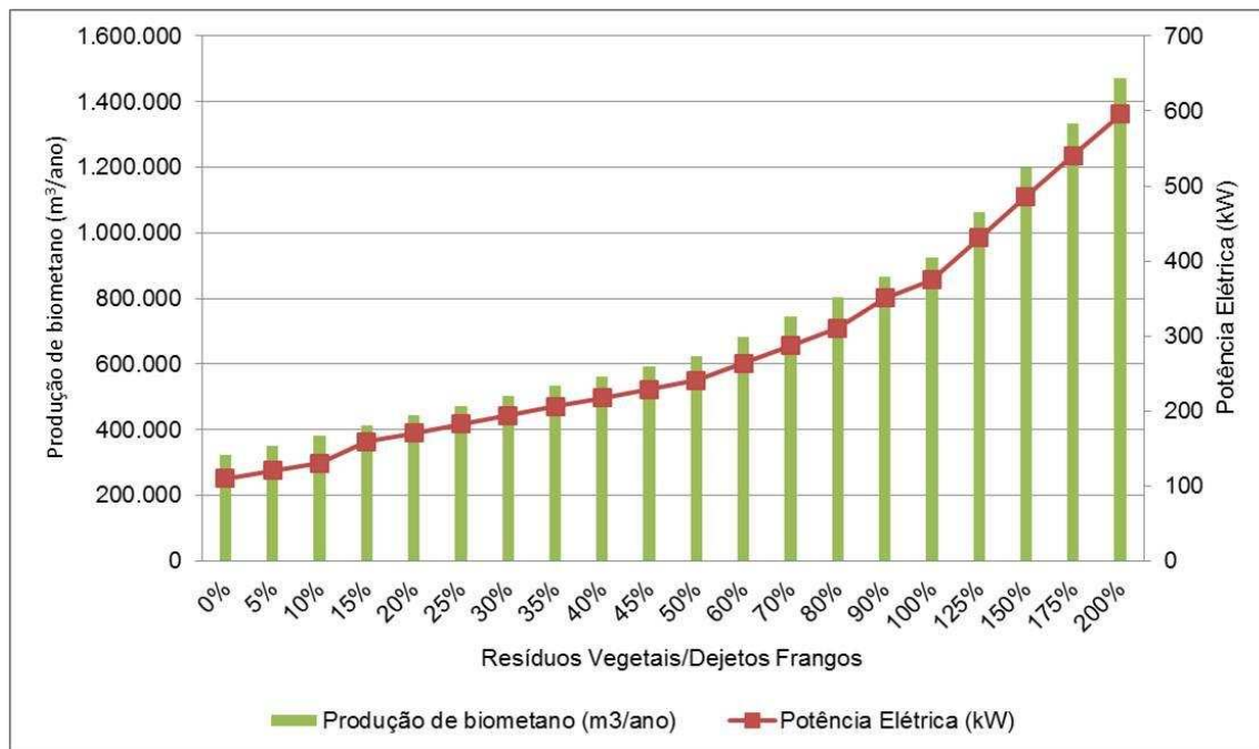
Figura 7.48 – Produção de biometano e potência elétrica.
