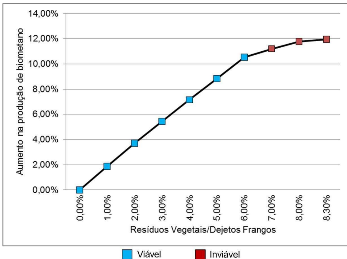
Figura 7.76 – Aumento na produção de biometano com a codigestão.
