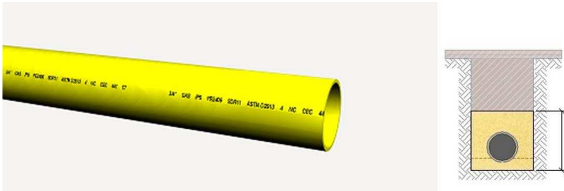
Figura 4.4 – Conceito do gasoduto.
