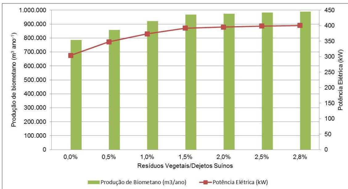
Figura 7.4 – Produção de biometano e potência elétrica.
