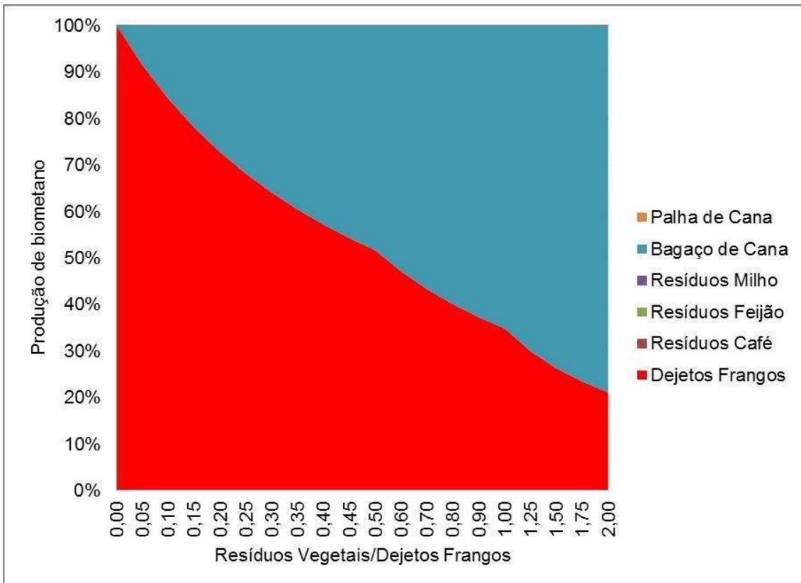
Figura 6.28 – Produção de metano por substrato para uma granja com 20.000 frangos no município de Mirafí.
