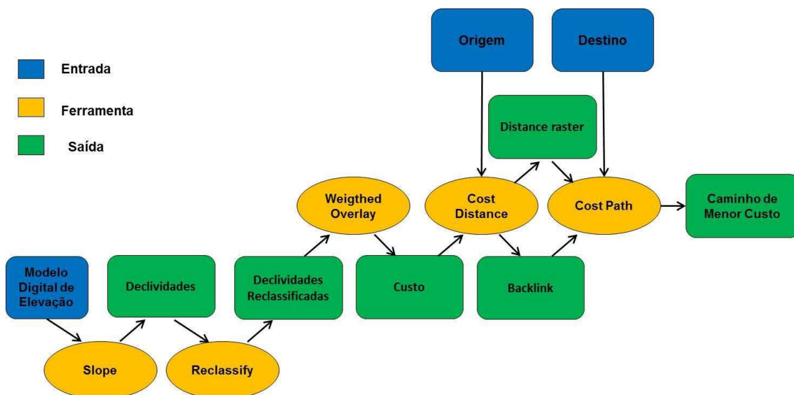
Figura 4.2 – Fluxograma representando a geração do caminho de menor custo para o duto.
