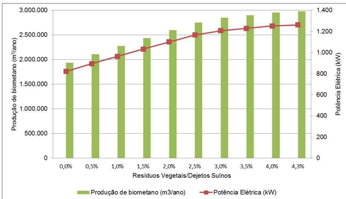
Figura 7.19 – Produção de biometano e potência elétrica.
