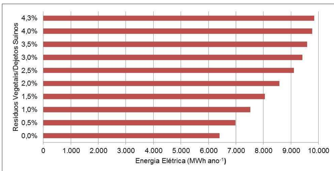
Figura 7.20 – Energia elétrica produzida.
