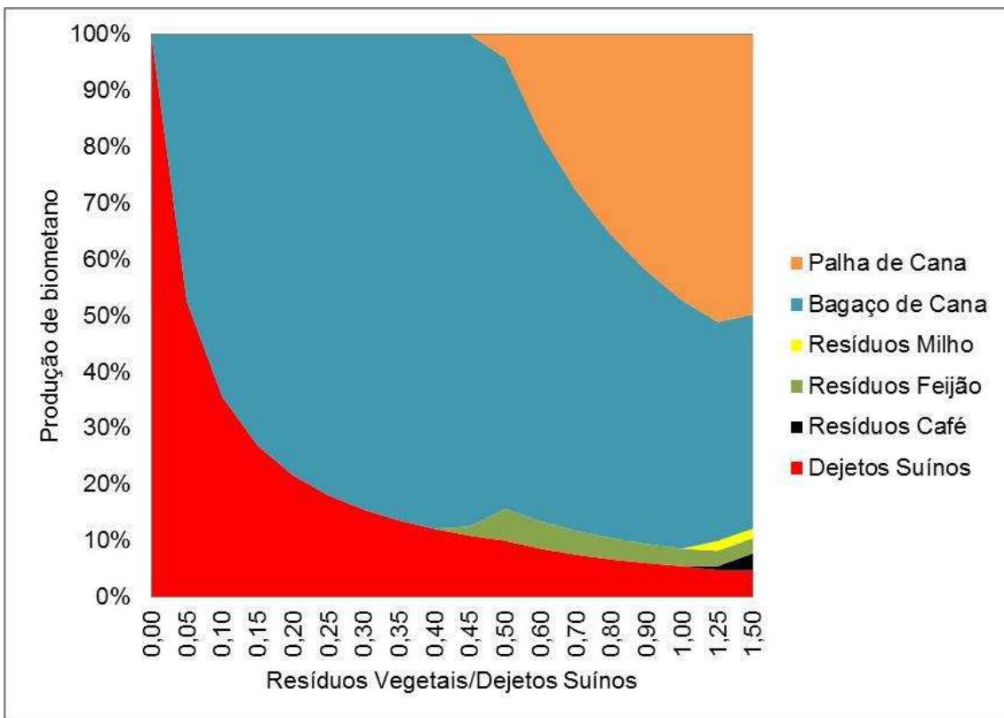
Figura 6.13 – Produção de metano por substrato para uma granja com 2.500 suínos no município de Jequeri.
