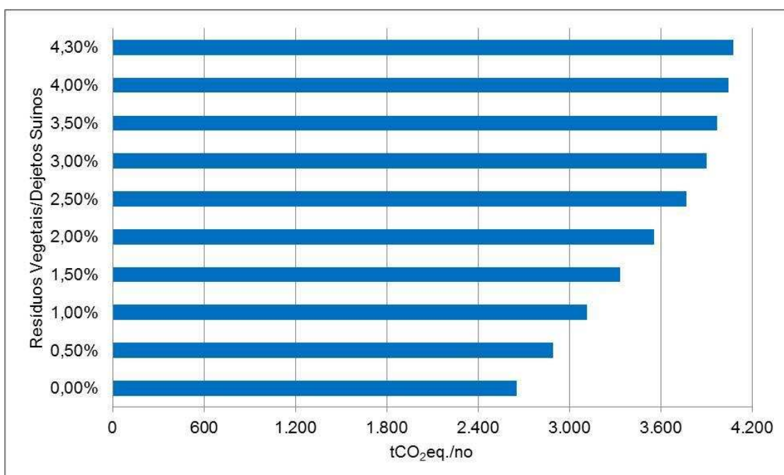
Figura 7.22 – Potencial de mitigação das emissões de CO 2 .
