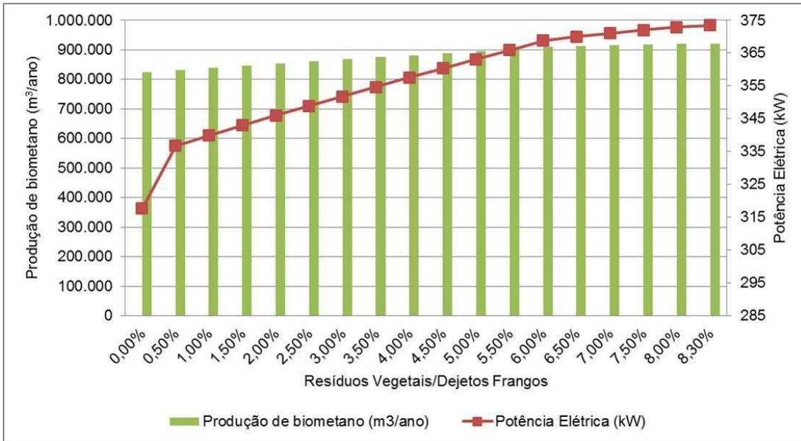
Figura 7.62 – Produção de biometano e potência elétrica.
