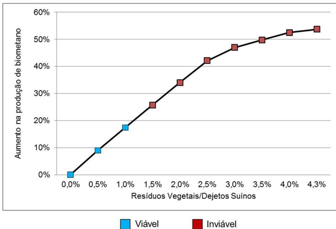
Figura 7.29 – Aumento na produção de biometano com a codigestão.
