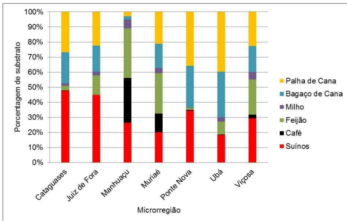
Figura 5.3 – Produção de biometano com dejetos de suínos e resíduos vegetais.
