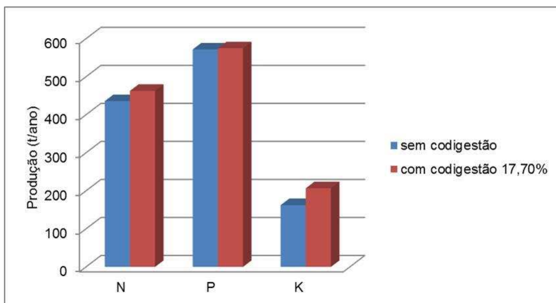
Figura 7.82 – Produção de biofertilizante no Condomínio de Agroenergia de São Miguel do Anta.
