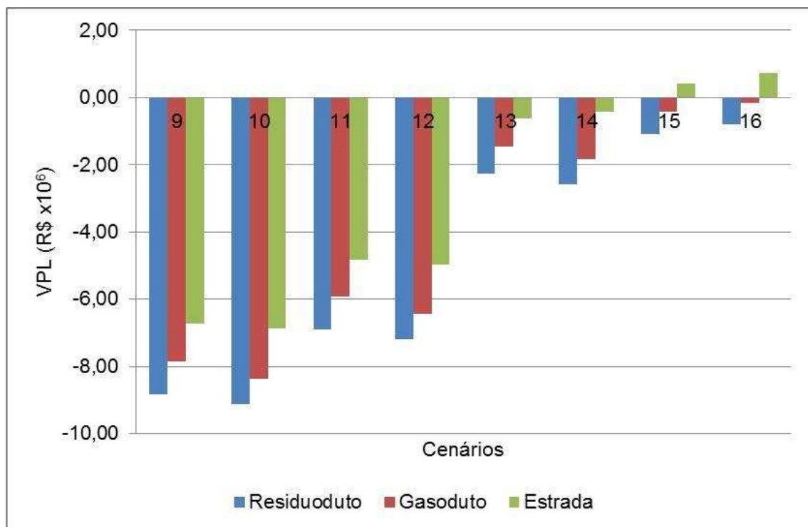
Figura 7.69 – VPL para os cenários de codigestão com 1,0% de razão resíduos vegetais/dejetos de frangos.
