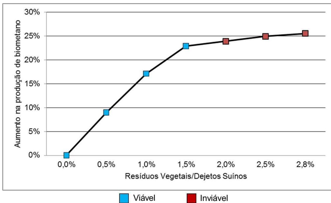
Figura 7.15 – Aumento na produção de biometano com a codigestão.
