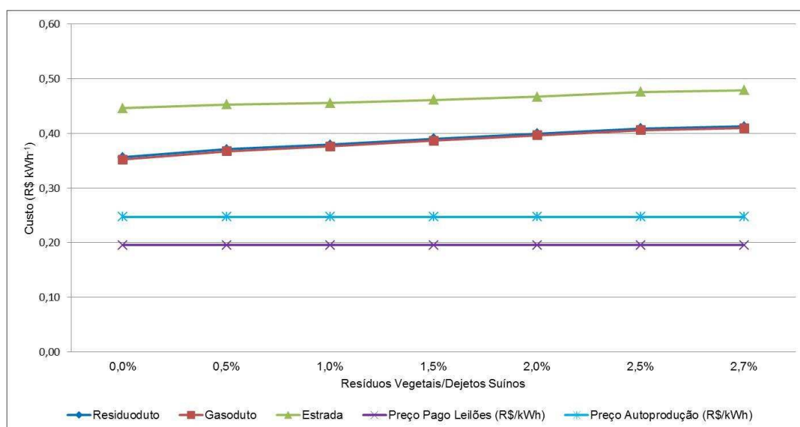
Figura 7.38 – Custo de produção de energia elétrica para diferentes modais de transporte no Condomínio de Agroenergia de Jequeri.
