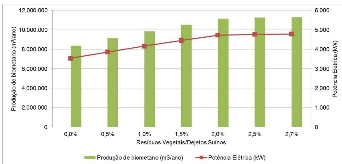
Figura 7.33 – Produção de biometano e potência elétrica.
