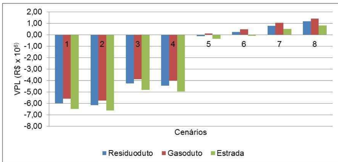
Figura 7.10 – VPL para os cenários sem codigestão.
