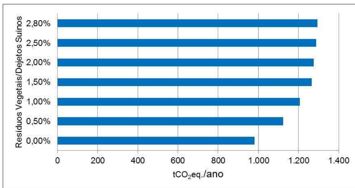
Figura 7.7 – Potencial de mitigação das emissões de CO 2 .
