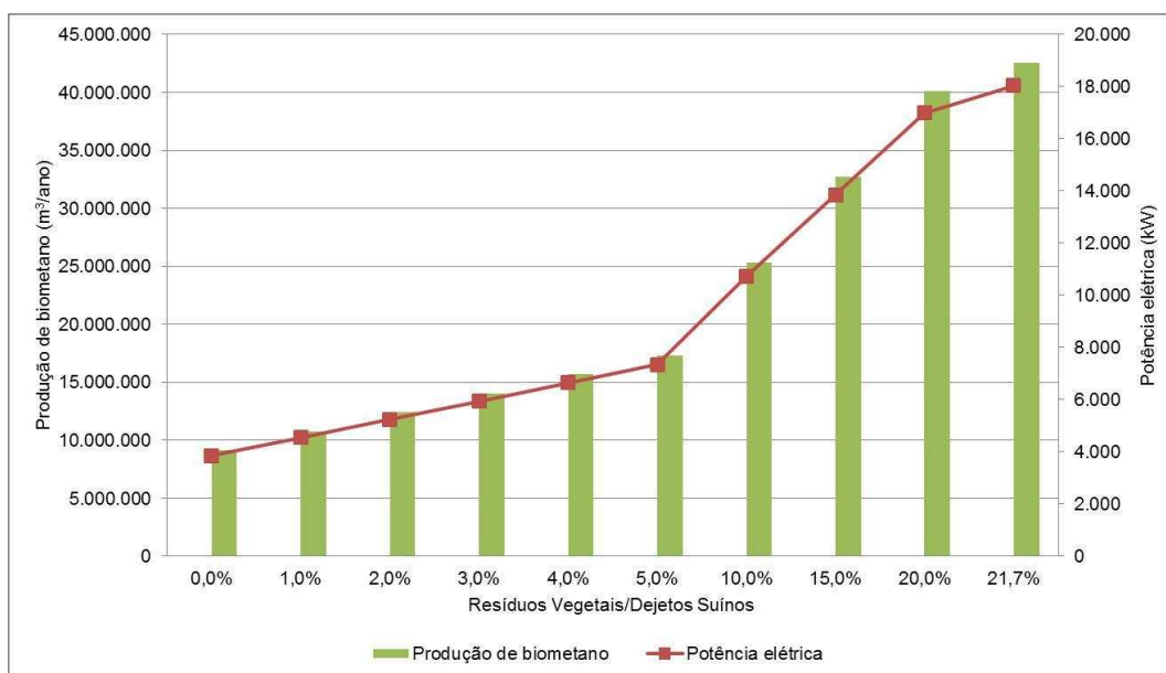
Figura 4.9 – Produção de biometano e potência elétrica.
