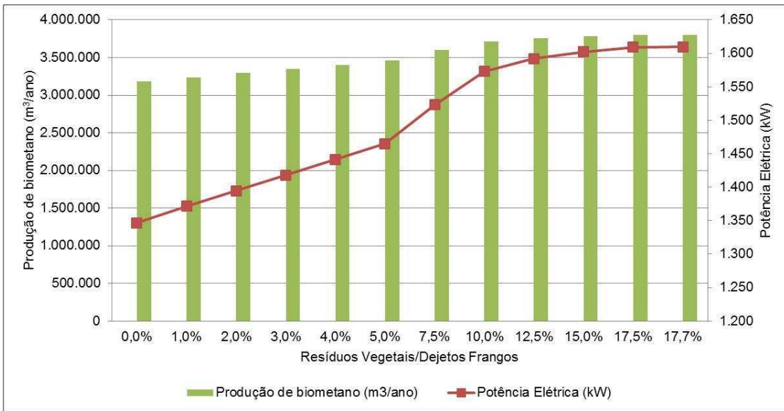
Figura 7.80 – Produção de biometano e potência elétrica.
