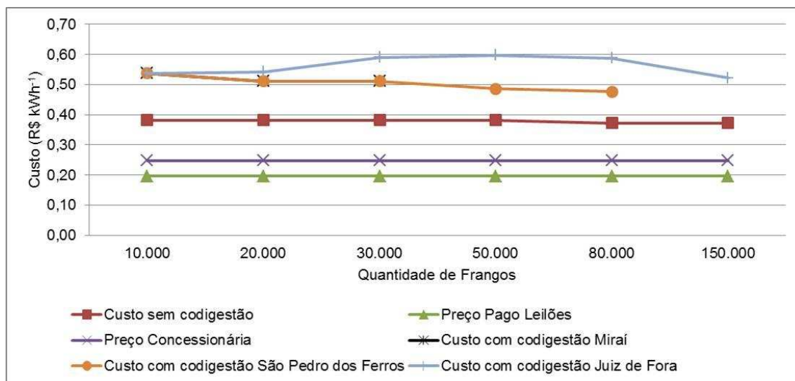
Figura 6.39 – Custo de produção de energia elétrica com codigestão de resíduos agropecuários em granjas com com 10.000, 20.000, 30.000, 50.000, 80.000 e 150.000 frangos nos municípios de Mirai, São Pedro dos Ferros e Juiz de Fora.
