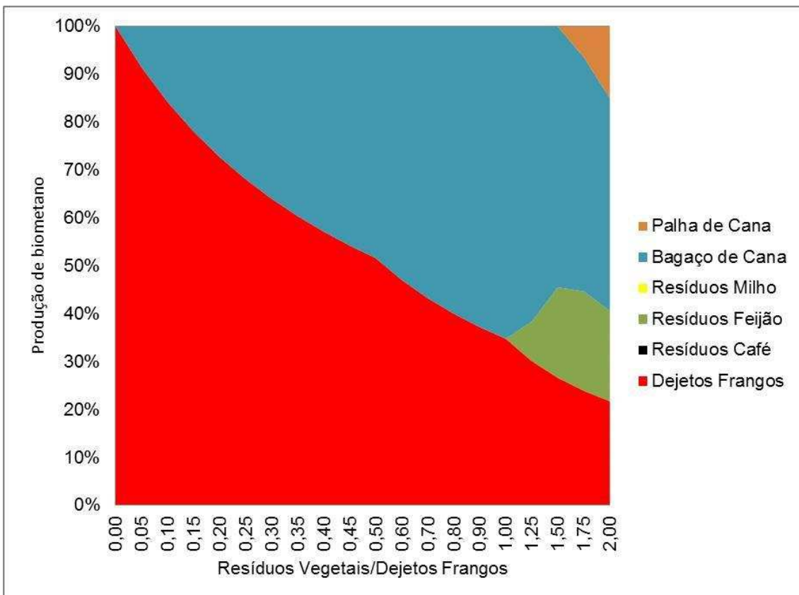
Figura 6.33 – Produção de metano por substrato para uma granja com 30.000 frangos no município de Juiz de Fora.
