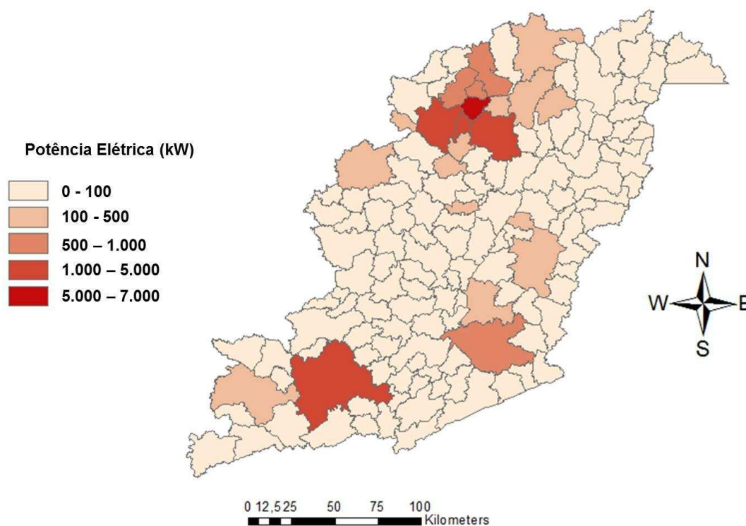
Figura 5.4 – Estimativa da potência elétrica produzida a partir dos dejetos da suinocultura.
