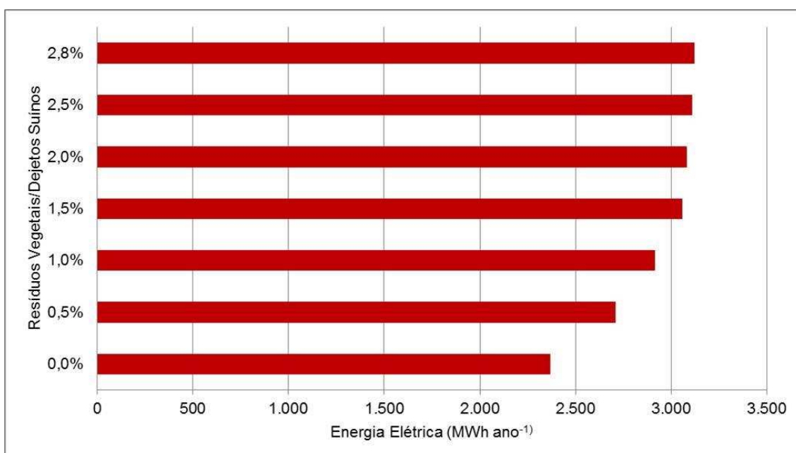
Figura 7.5 – Energia elétrica produzida.
