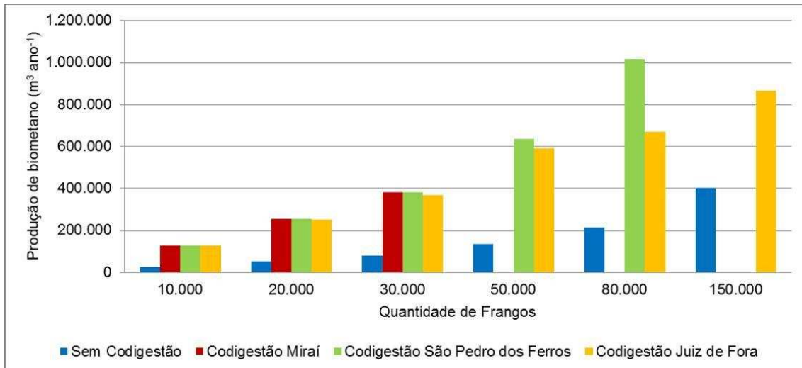
Figura 6.24 – Produção de biometano em granjas dos municípios de Mirai, São Pedro dos Ferros e Juiz de Fora.
