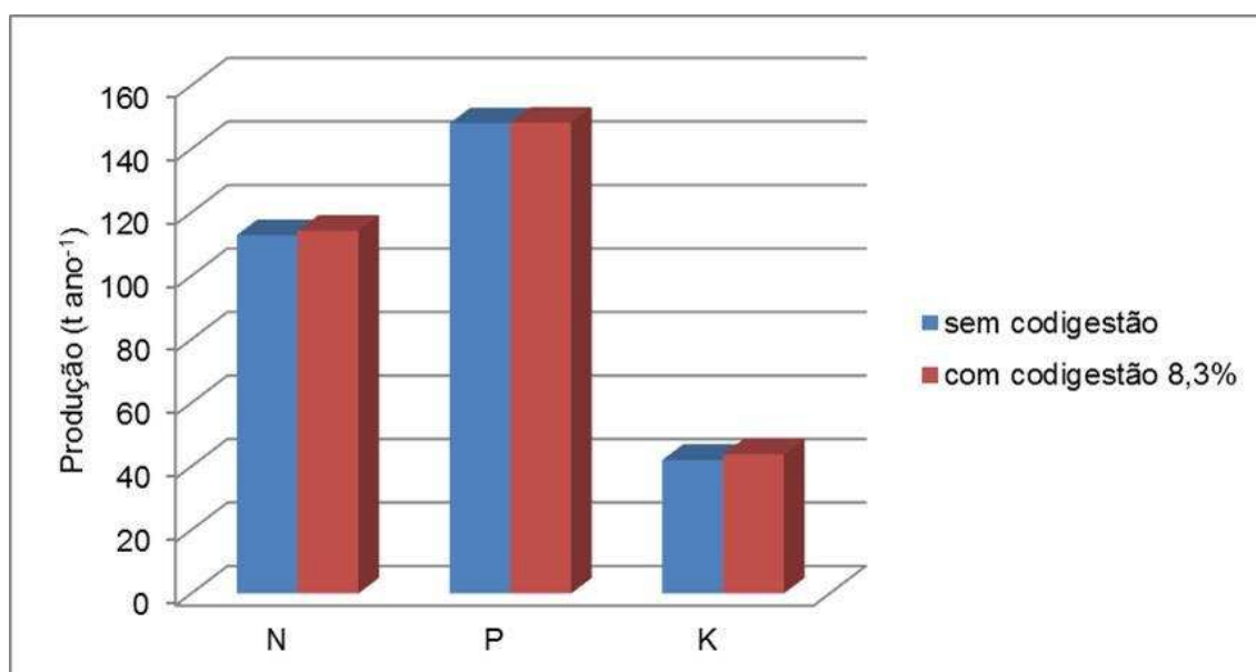
Figura 7.64 – Produção de biofertilizante no Condomínio de Agroenergia de Piraúba.
