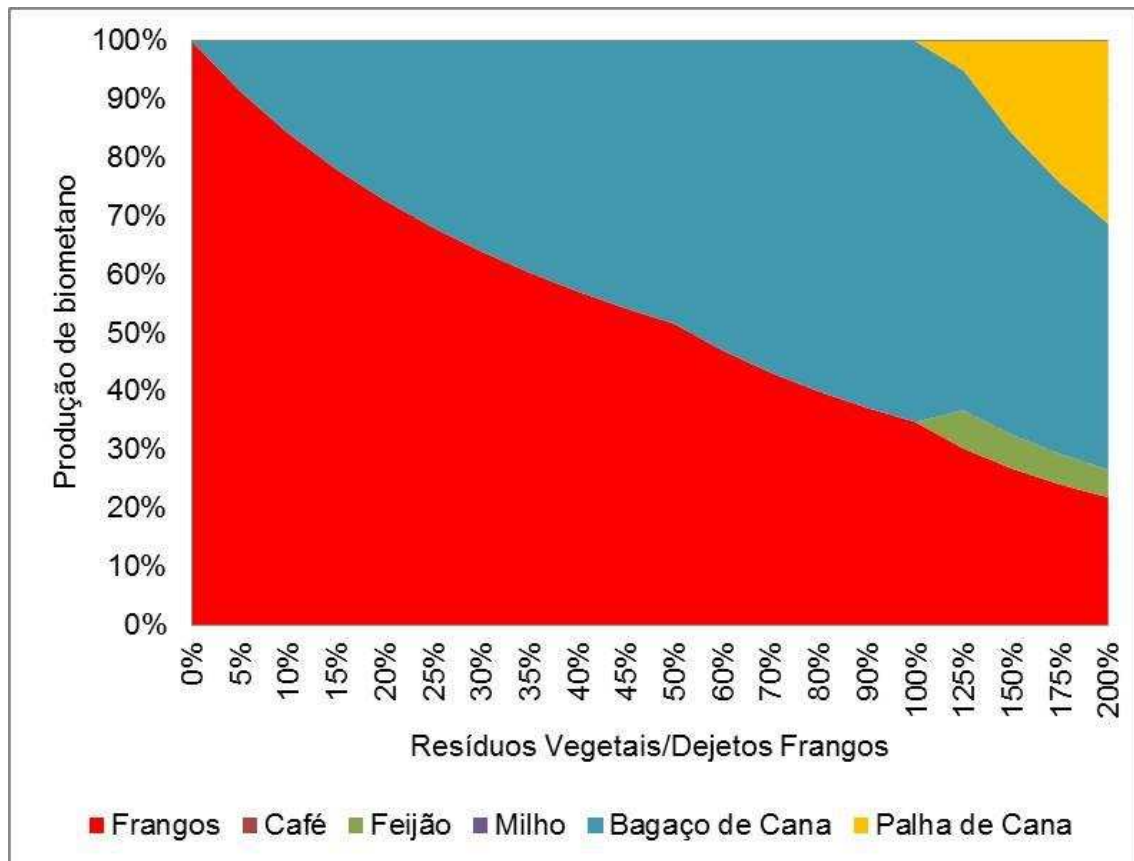
Figura 7.47 – Produção de biometano por substrato.
