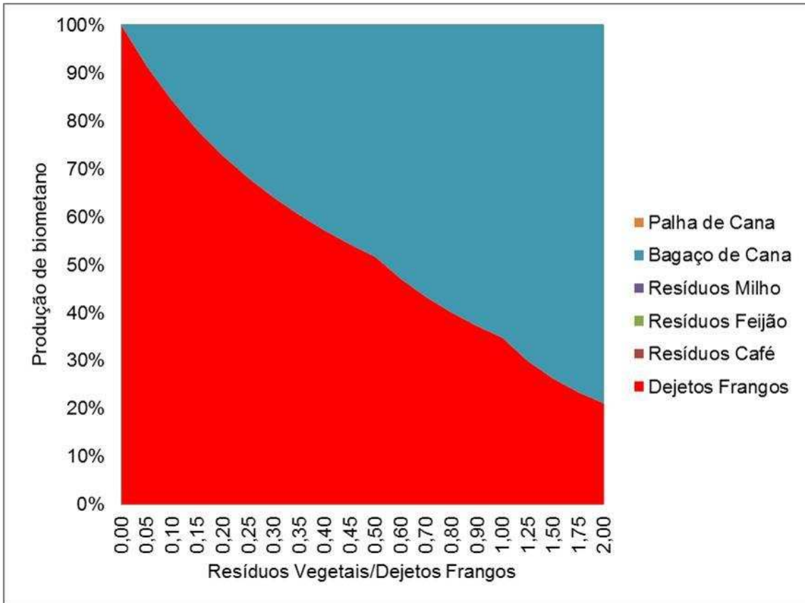
Figura 6.25 – Produção de metano por substrato para uma granja com 10.000 frangos no município de Miraf.
