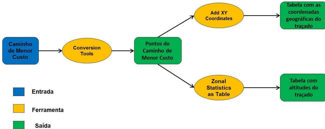
Figura 4.3 – Fluxograma representando a geração das tabelas de altitude e coordenadas geográficas do caminho de menor custo.
