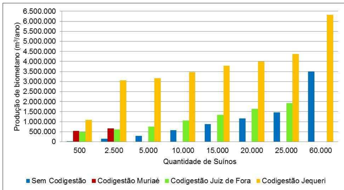
Figura 6.7 – Produção de biometano em granjas dos municípios de Muriaé, Juiz de Fora e Jequeri.
