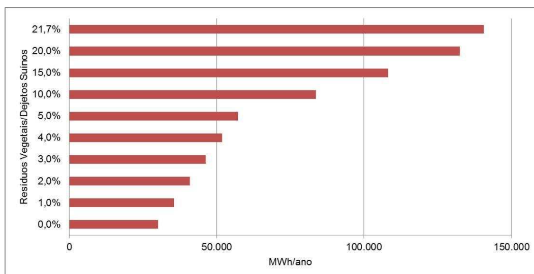
Figura 4.10 – Energia elétrica produzida.
