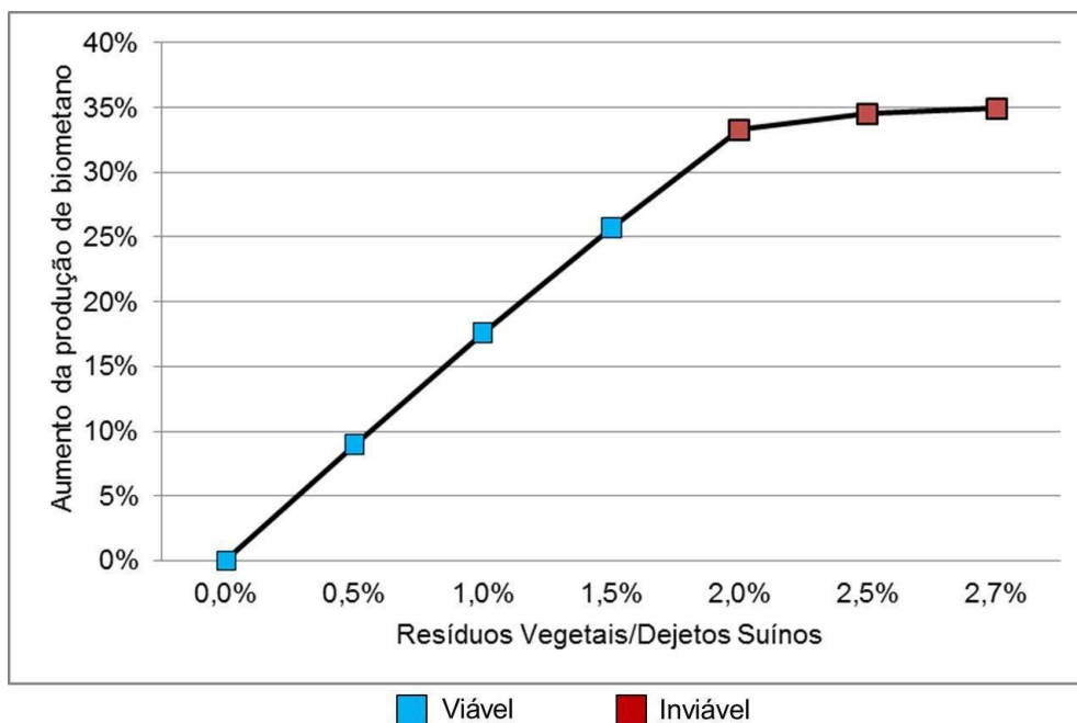
Figura 7.44 – Aumento na produção de biometano com a codigestão.
