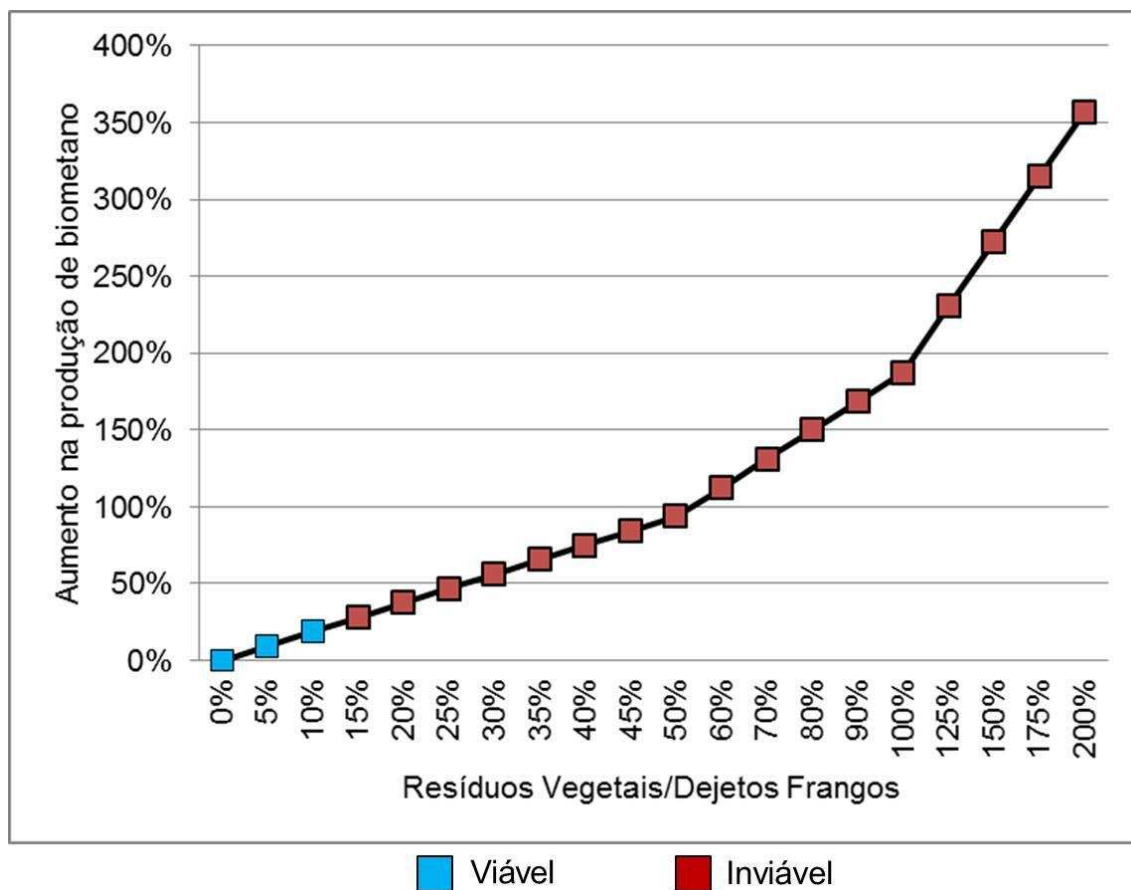
Figura 7.58 – Aumento na produção de biometano com a codigestão.
