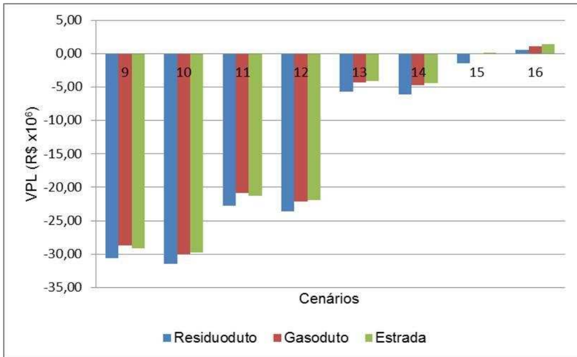
Figura 7.88 – VPL para os cenários de codigestão com 2,0% de razão resíduos vegetais/dejetos de frangos.
