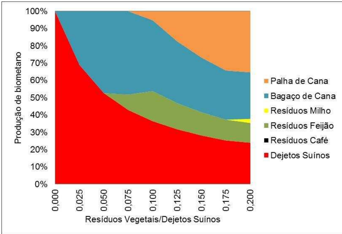
Figura 6.12 – Produção de metano por substrato para uma granja com 2.500 suínos no município de Juiz de Fora.
