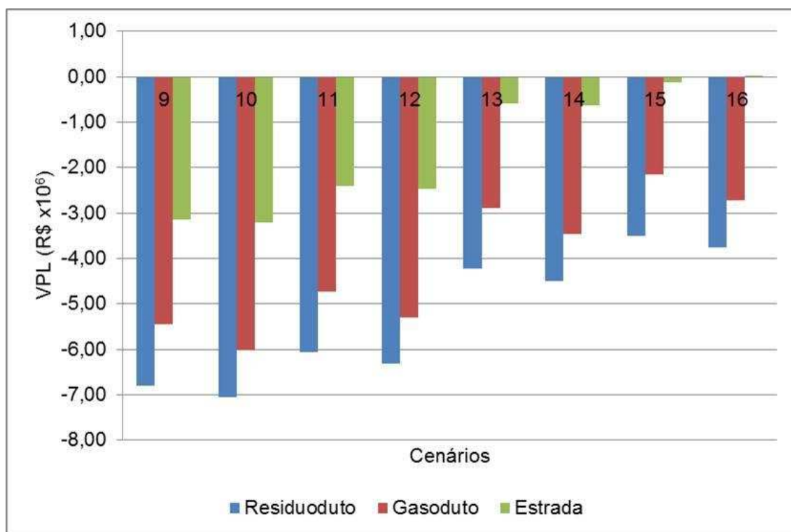
Figura 7.56 – VPL para os cenários de codigestão com 10% de razão resíduos vegetais/dejetos de frangos.
