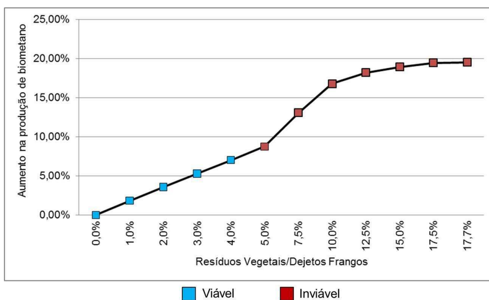
Figura 7.92 – Aumento na produção de biometano com a codigestão.
