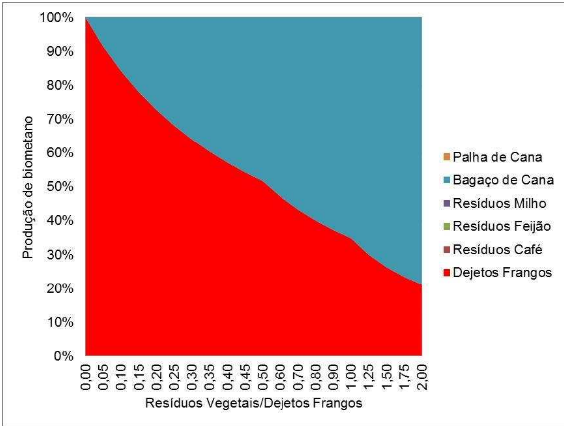
Figura 6.31 – Produção de metano por substrato para uma granja com 30.000 frangos no município de Mirai.
