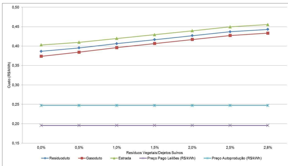
Figura 7.9 – Custo de produção de energia elétrica para diferentes modais de transporte no Condomínio de Agroenergia de Faria Lemos.
