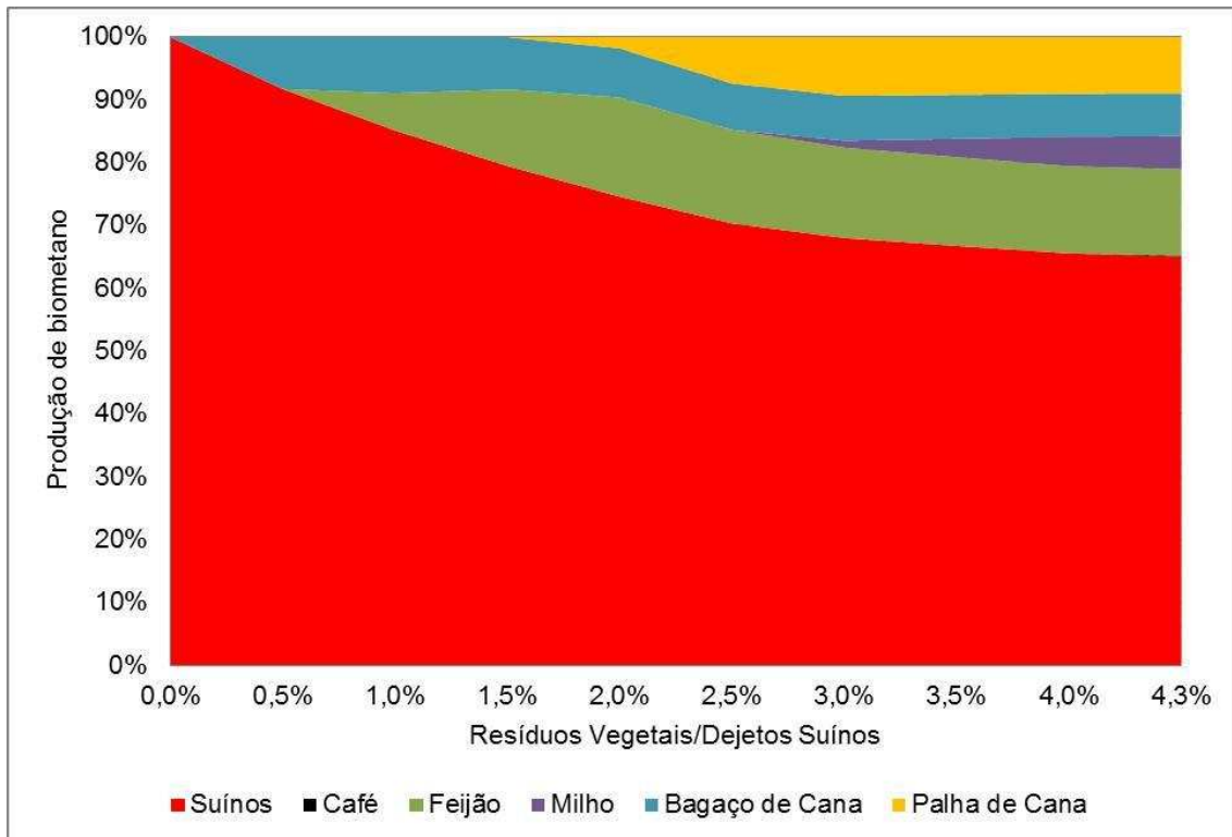
Figura 7.18 – Produção de biometano por substrato.
