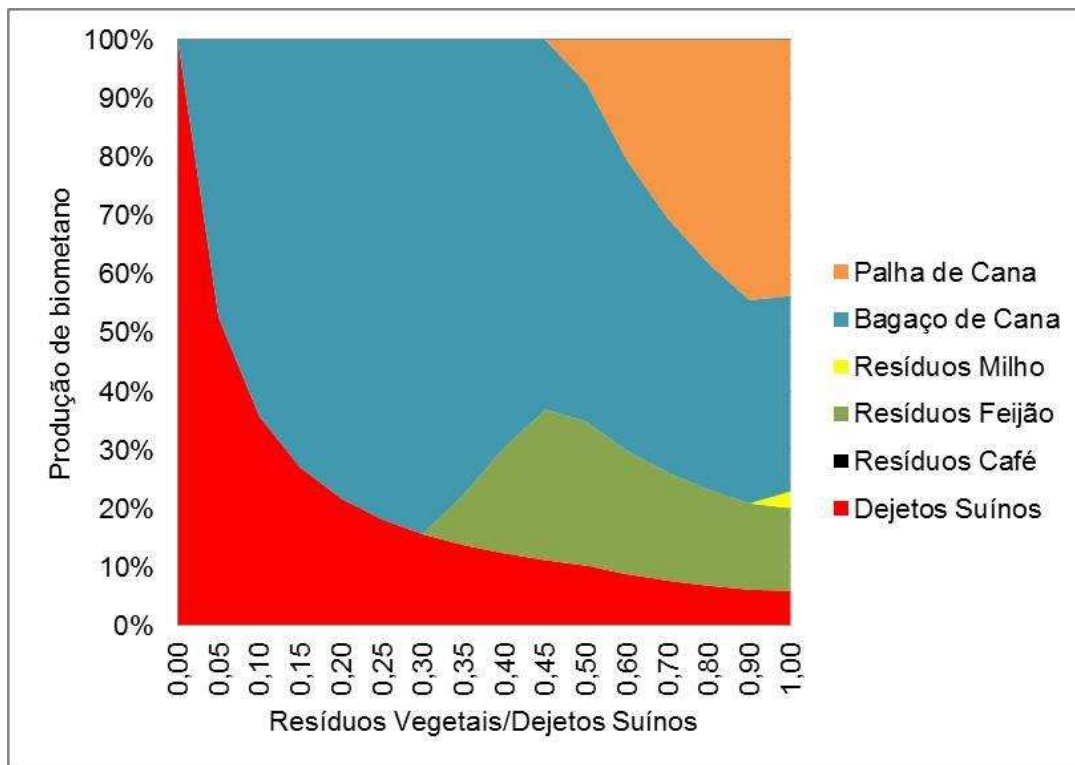
Figura 6.9 – Produção de metano por substrato para uma granja com 500 suínos no município de Juiz de Fora.
