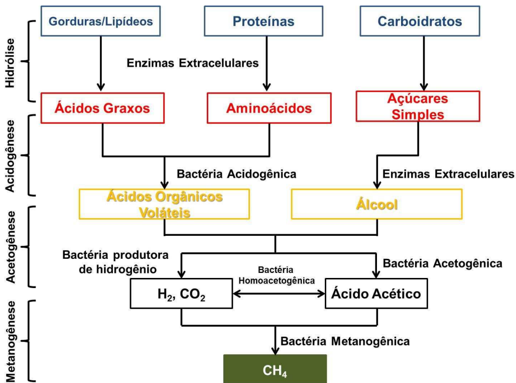
Figura 3.1 – Esquema da digestão anaeróbia.
