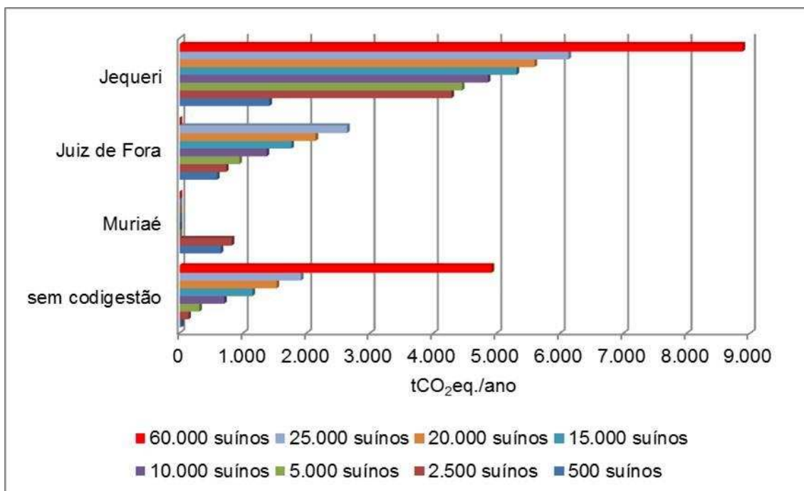
Figura 6.18 – Potencial de toneladas de dióxido de carbono para granjas de suínos nos municípios de Muriaé, Juiz de Fora e Jequeri.
