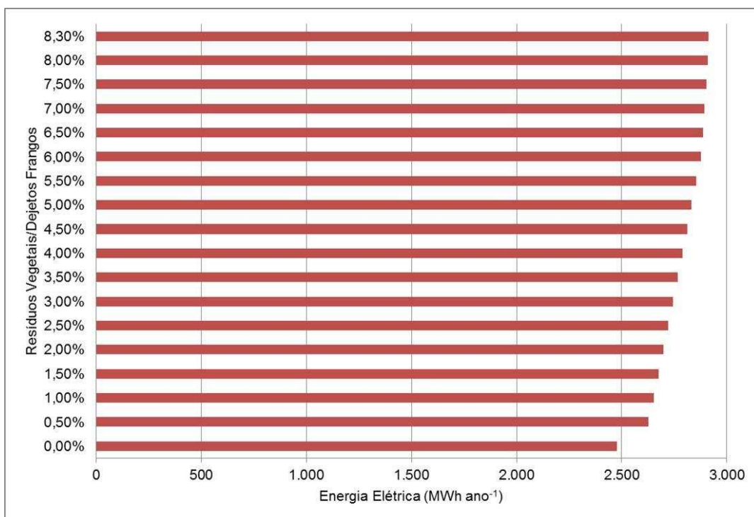
Figura 7.63 – Energia elétrica produzida.
