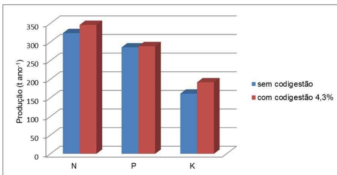
Figura 7.21 – Produção de biofertilizante no Condomínio de Agroenergia de Piranga.
