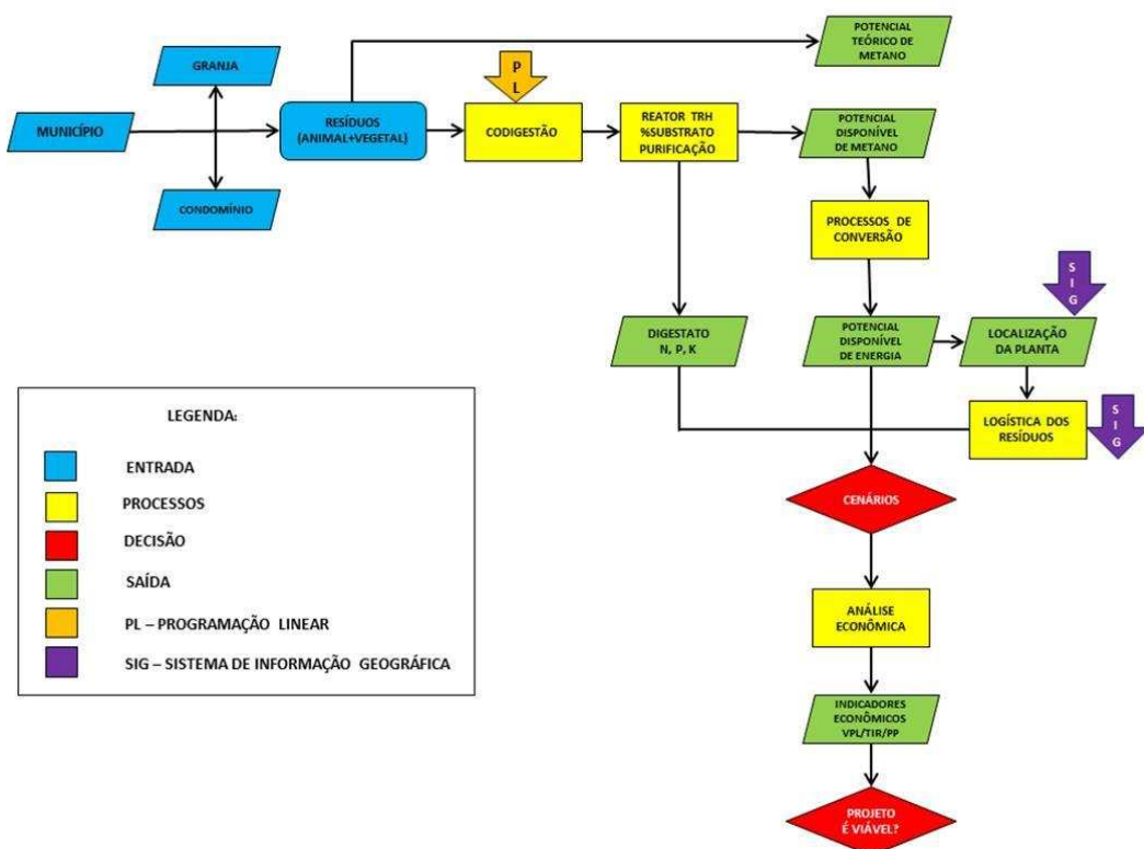
Figura 4.1 – Fluxograma da Ferramenta Computacional SAUDADE.
