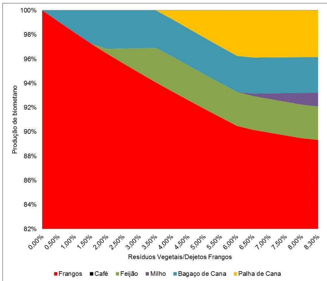
Figura 7.61 – Produção de biometano por substrato.
