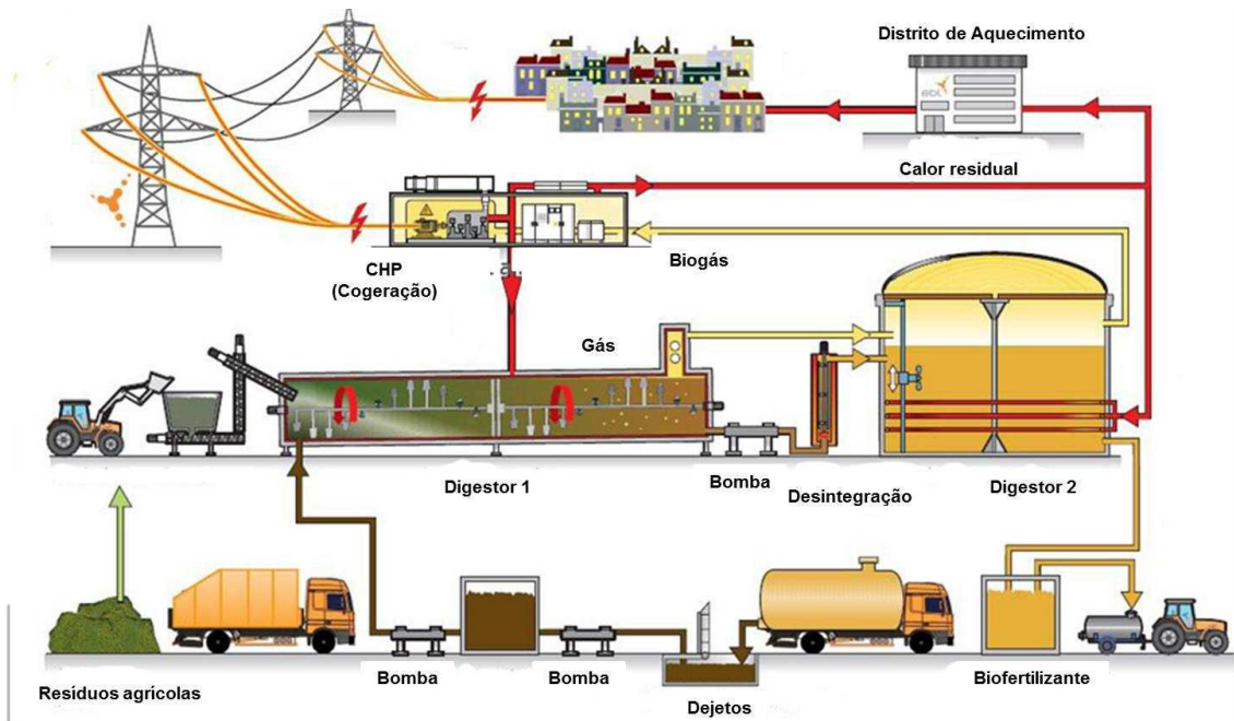
Figura 3.2 – Usina de codigestão.
