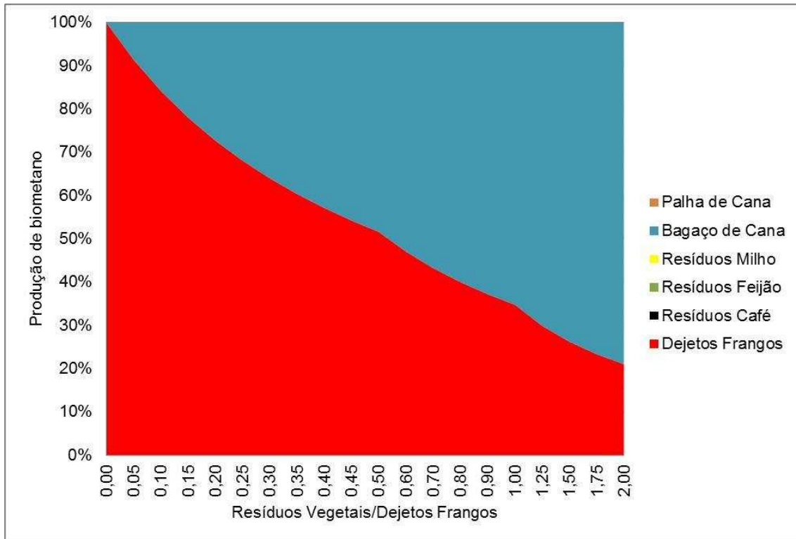
Figura 6.27 – Produção de metano por substrato para uma granja com 10.000 frangos no município de Juiz de Fora.
