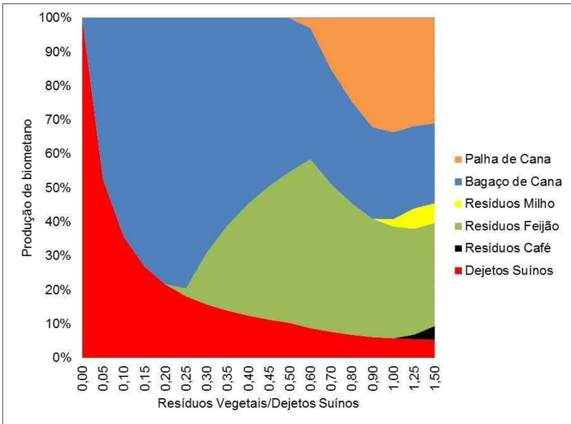
Figura 6.8 – Produção de metano por substrato para uma granja com 500 suínos no município de Muriaé.
