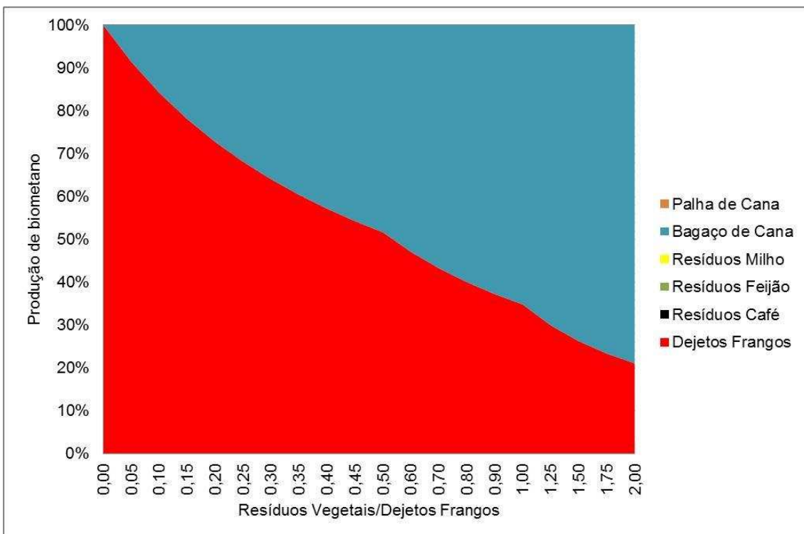
Figura 6.26 – Produção de metano por substrato para uma granja com 10.000 frangos no município de São Pedro dos Ferros.
