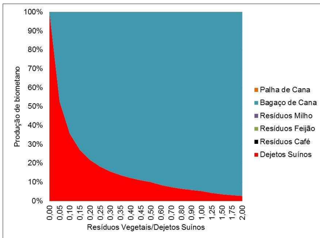
Figura 6.10 – Produção de metano por substrato para uma granja com 500 suínos no município de Jequeri.
