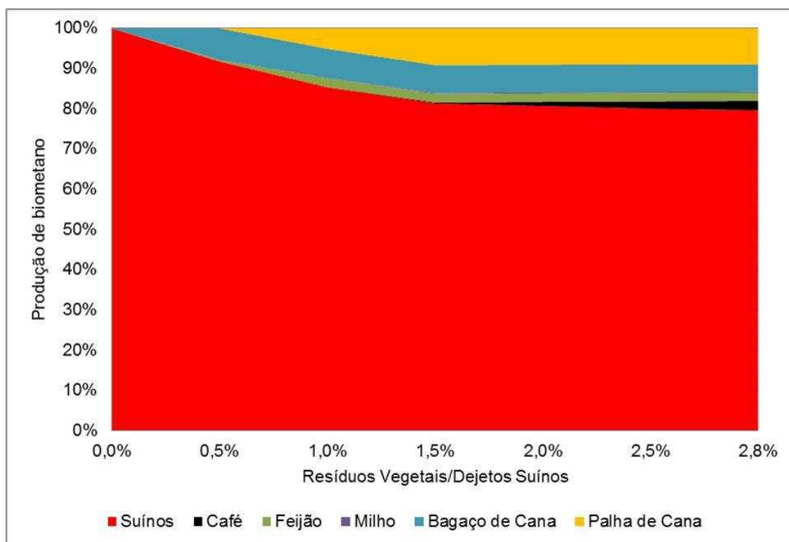
Figura 7.3 – Produção de biometano por substrato.
