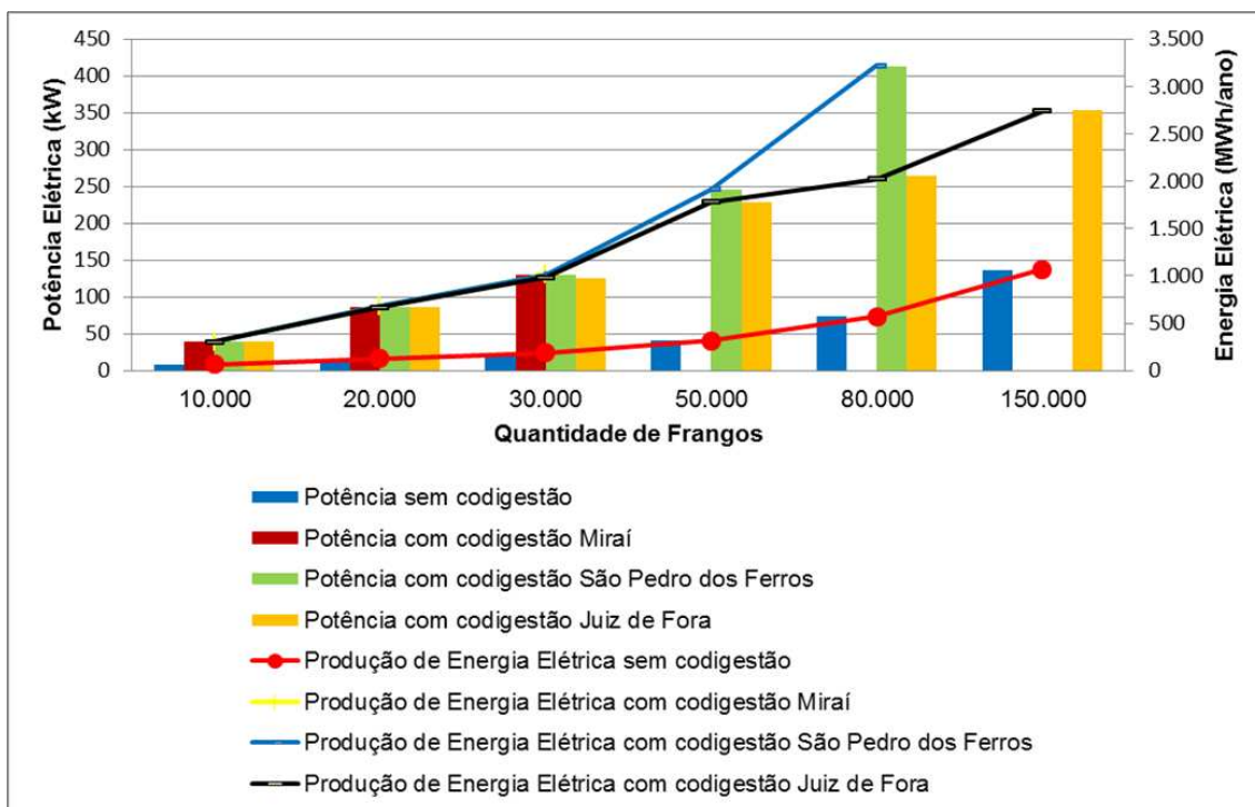
Figura 6.34 – Potência e energia elétrica gerada em granjas dos municípios de Mirai, São Pedro dos Ferros e Juiz de Fora.
