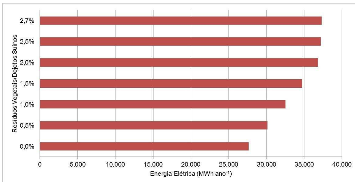
Figura 7.34 – Energia elétrica produzida.
