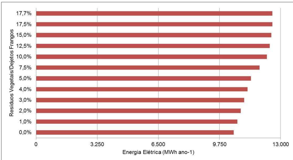
Figura 7.81 – Energia elétrica produzida.
