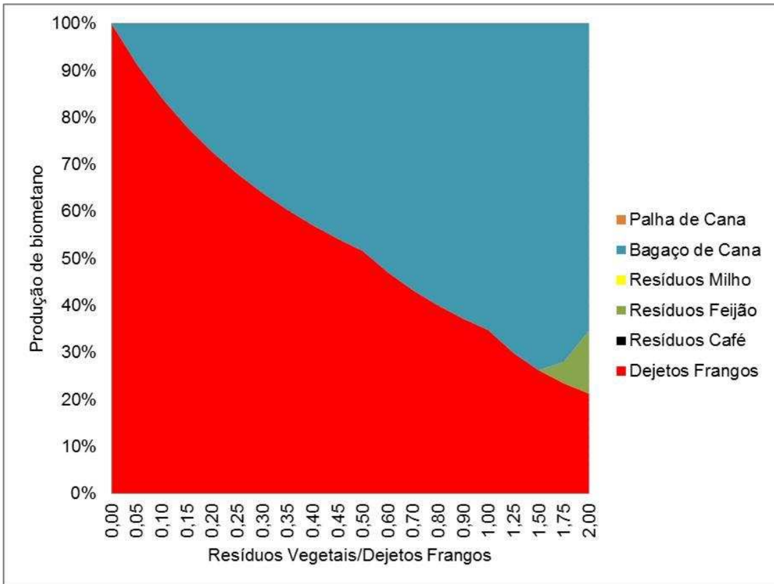
Figura 6.30 – Produção de metano por substrato para uma granja com 20.000 frangos no município de Juiz de Fora.
