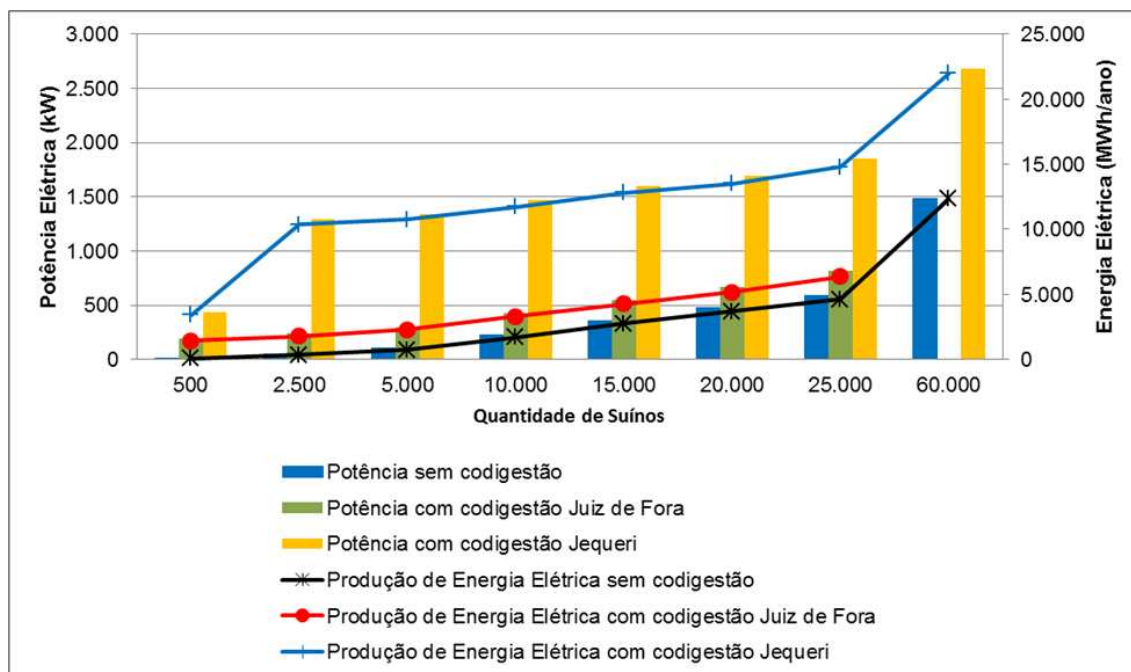
Figura 6.15 – Potência e energia elétrica gerada em granjas dos municípios de Juiz de Fora e Jequeri.
