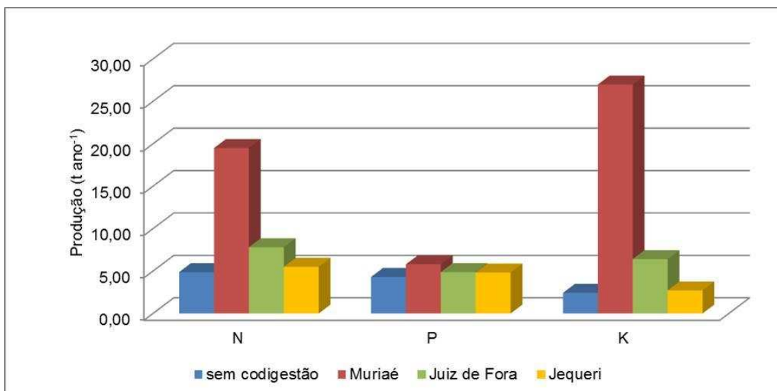
Figura 6.16 – Produção de biofertilizante em granja com 500 suínos nos municípios de Muriaé, Juiz de Fora e Jequeri.
