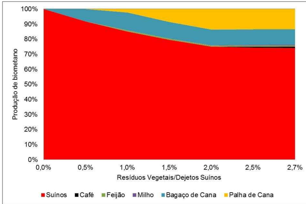
Figura 7.32 – Produção de biometano por substrato.
