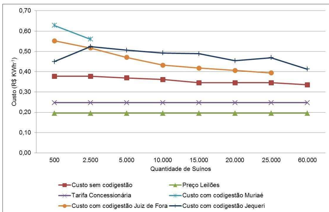
Figura 6.19 – Custo de produção de energia elétrica com codigestão de resíduos agropecuárias em granjas com 500, 2.500, 5.000, 10.000, 15.000, 20.000, 25.000 e 60.000 suínos nos municípios de Muriaé, Juiz de Fora e Jequeri.
