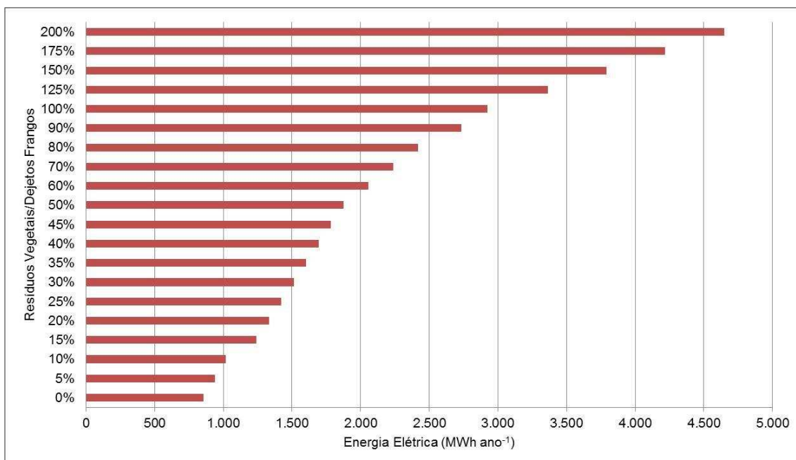
Figura 7.49 – Energia elétrica produzida.
