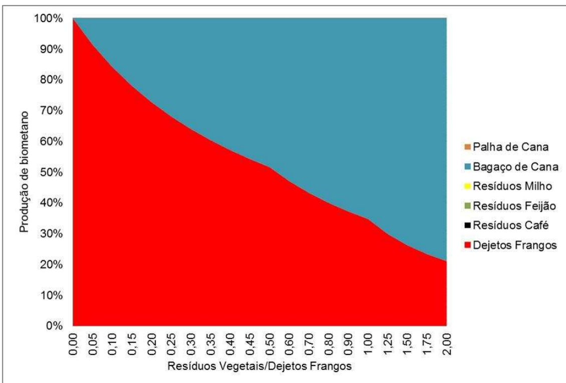
Figura 6.29 – Produção de metano por substrato para uma granja com 20.000 frangos no município de São Pedro dos Ferros.
