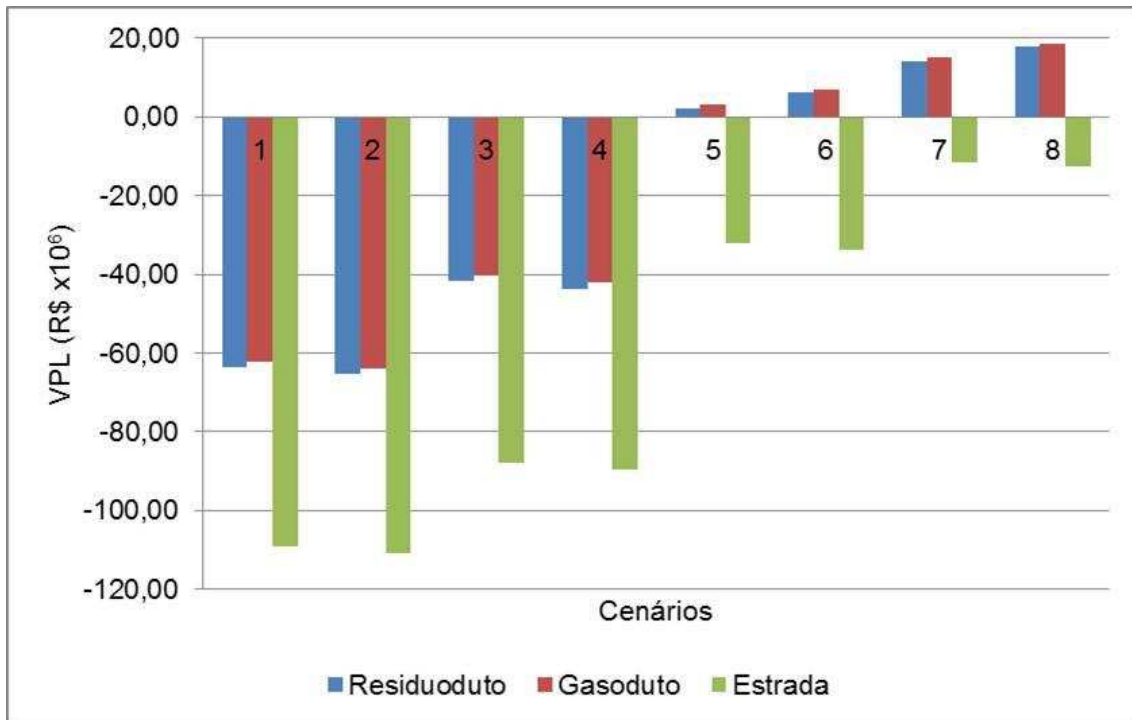
Figura 4.15 – VPL para os cenários sem codigestão.
