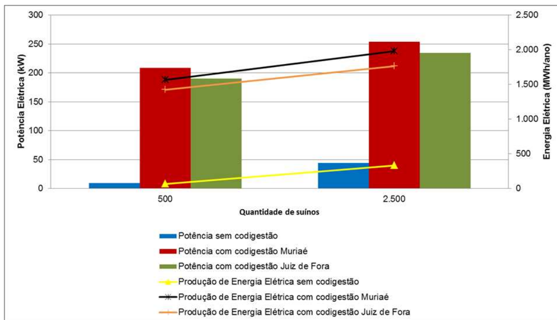
Figura 6.14 – Potência e energia elétrica gerada em granjas dos municípios de Muriaé e Juiz de Fora.
