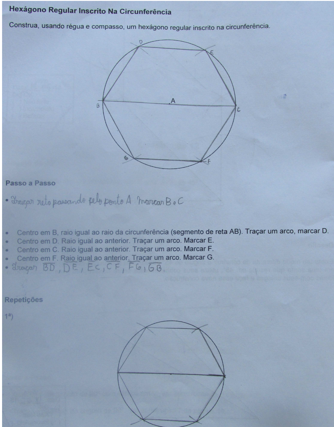
Figura A.4: Construção hexágono regular – Atividade 2
