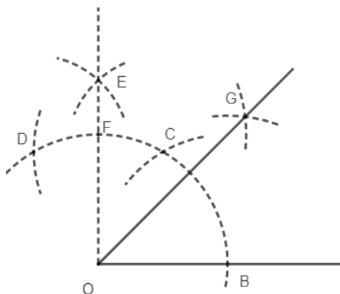
Figura 2.28: Ângulo de 45^\circ
