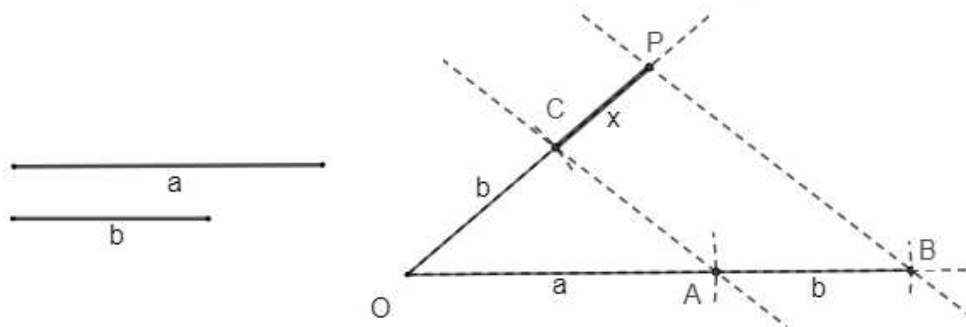
Figura 3.5: x é a 3ª proporcional entre a e b .
