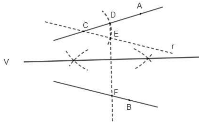
Figura 2.31: Bissetriz de um ângulo com vértice inacessível
