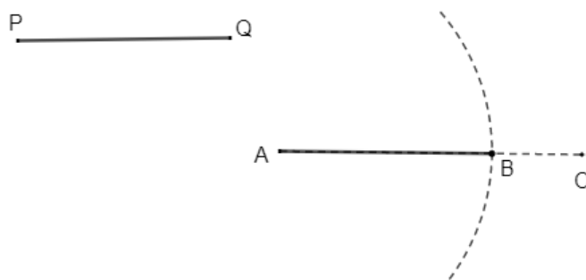
Figura 2.7: Transporte de segmento de reta
