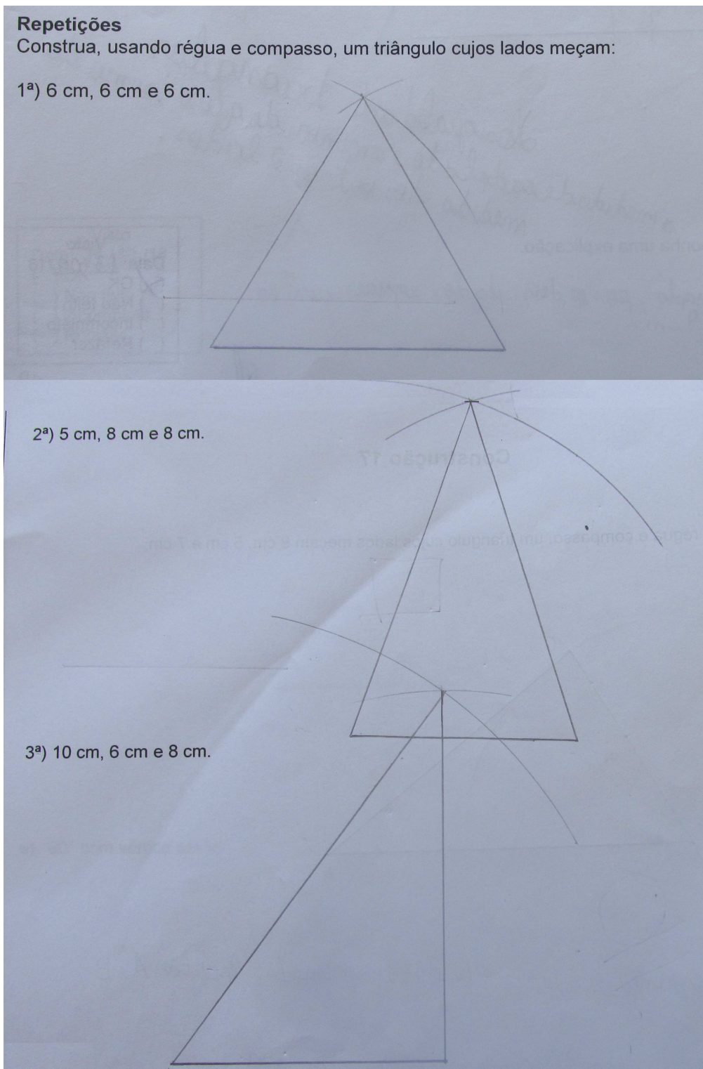
Figura A.2: Trabalho autônomo do estudante – Atividade 1
