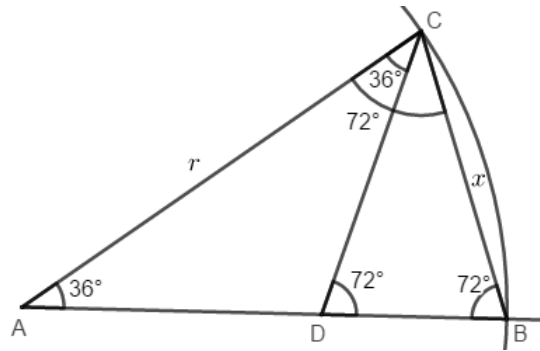
Figura 4.5: Triângulo isósceles ABC
