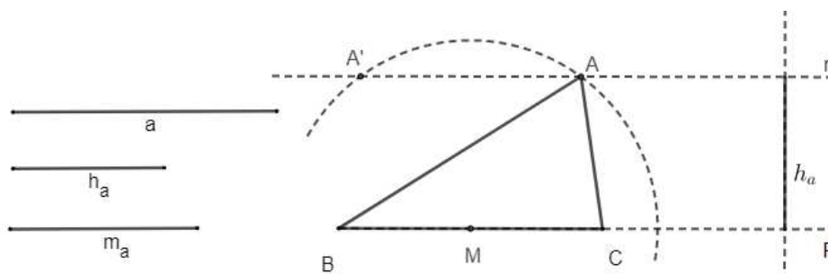
Figura 2.22: Triângulo conhecidos um lado, a altura e a mediana relativas a ele
