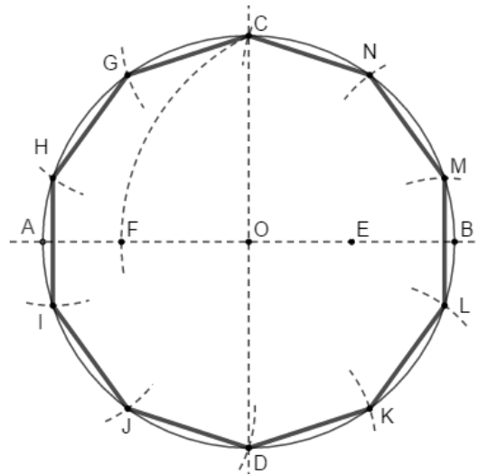
Figura 4.4: Decágono regular inscrito na circunferência
