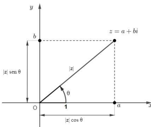
Figura 3.17: z = a + bi = |z|(\cos\theta + i\sin\theta)
