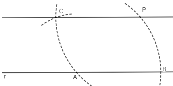
Figura 2.14: Retas paralelas II
