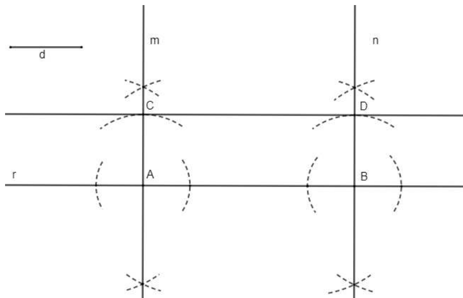
Figura 2.13: Retas Paralelas I
