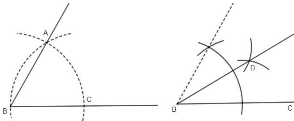
Figura 2.24: Ângulos de 60^\circ e 30^\circ
