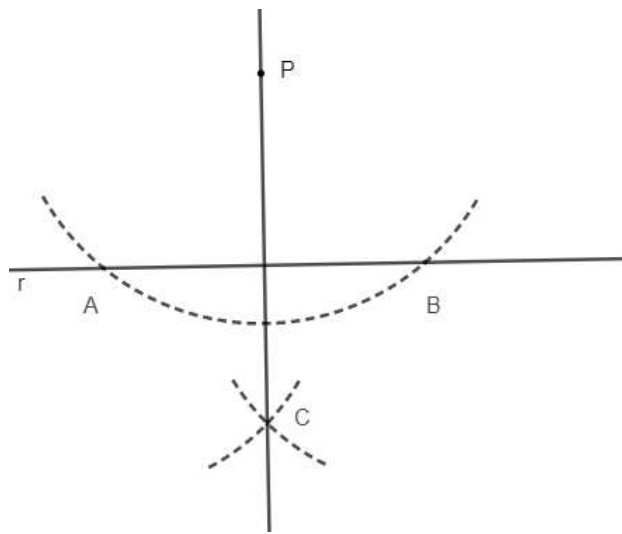
Figura 2.11: Reta Perpendicular à r passando por P , P \notin r .
