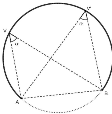
Figura 2.6: Arco capaz
