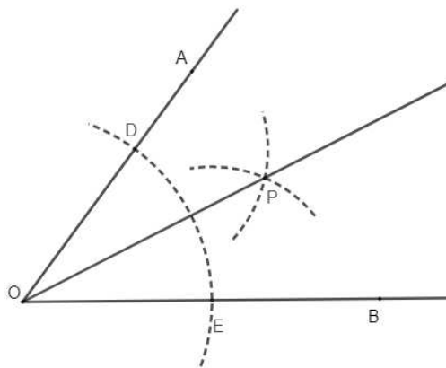
Figura 2.12: Bissetriz de um ângulo
