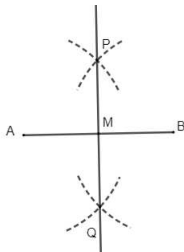
Figura 2.9: Reta mediatriz
