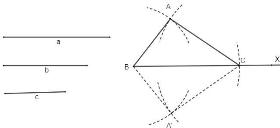
Figura 2.17: Triângulo conhecidas as medidas de seus lados
