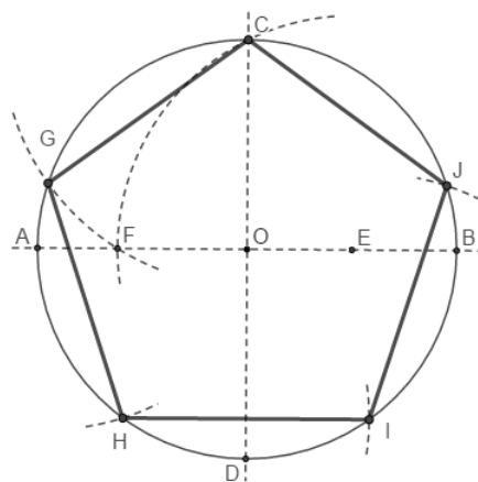
Figura 4.7: Pentágono regular
