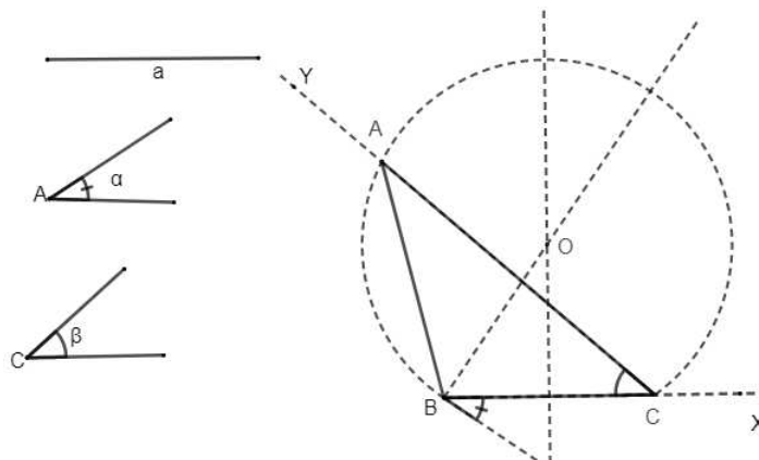
Figura 2.20: Triângulo conhecidas as medidas de um lado, um ângulo adjacente e um ângulo oposto
