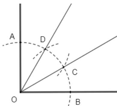
Figura 2.30: Dividir um ângulo reto em três parte congruentes
