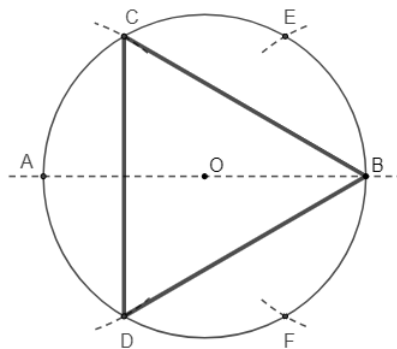
Figura 4.3: Triângulo equilátero inscrito na circunferência
