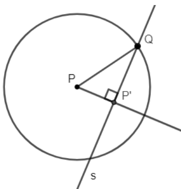
Figura 2.3: A reta s é secante à circunferência.
