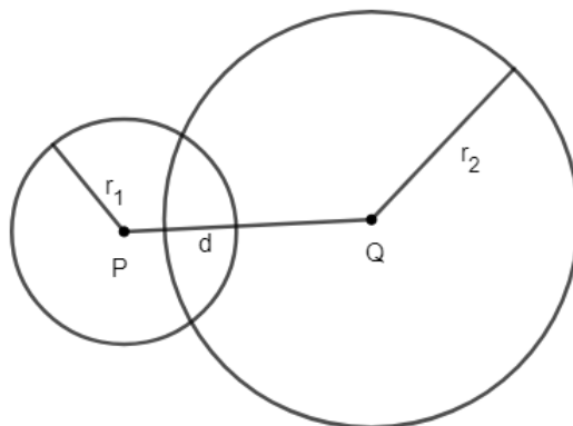
Figura 2.4: Circunferências secantes
