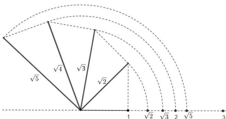
Figura 3.3: Segmentos iguais a \sqrt{2} , \sqrt{3} , ... etc.
