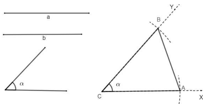
Figura 2.18: Triângulo conhecidas as medidas de dois lados e do ângulo entre eles
