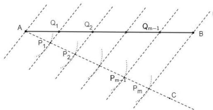
Figura 3.9: Segmento dividido em m partes iguais.
