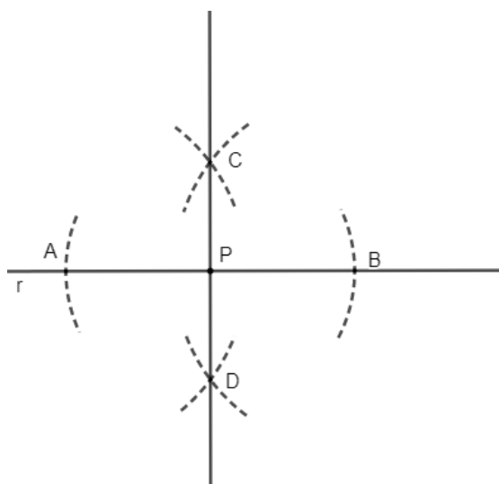
Figura 2.10: Reta perpendicular à r passando por P , P \in r .
