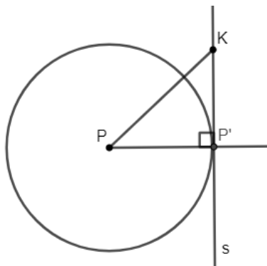
Figura 2.2: A reta s é tangente à circunferência.
