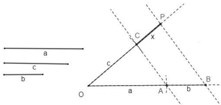
Figura 3.4: x é a 4ª proporcional de a , b e c .
