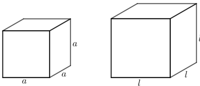
Figura 3.18: V_1 = a^3, V_2 = l^3, V_2 = 2 \cdot V_1
