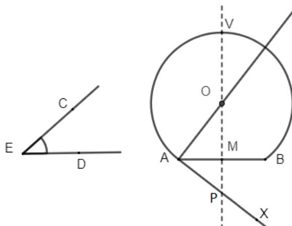
Figura 2.15: \widehat{AVB} é o arco capaz de C\hat{E}D
