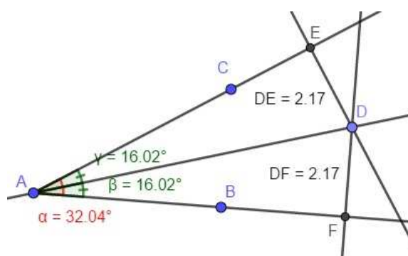
Figura 5.2: Atividade 3 - Bissetriz 1ª parte
