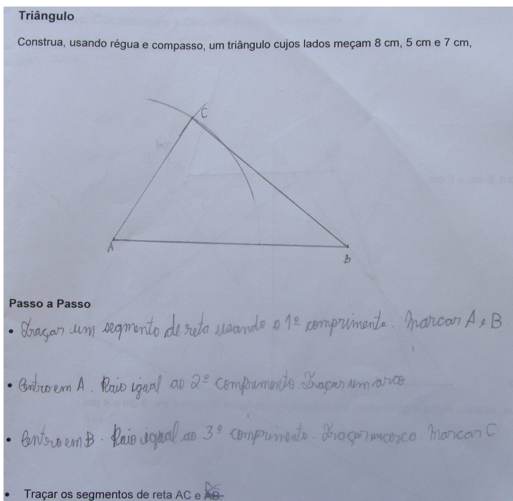
Figura A.1: Construção do triângulo e passo a passo – Atividade 1
