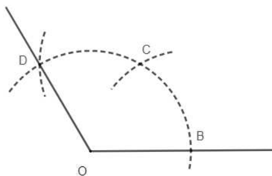
Figura 2.26: Ângulo de 120^\circ
