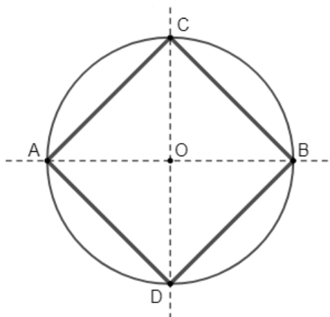
Figura 4.1: Quadrado inscrito na circunferência
