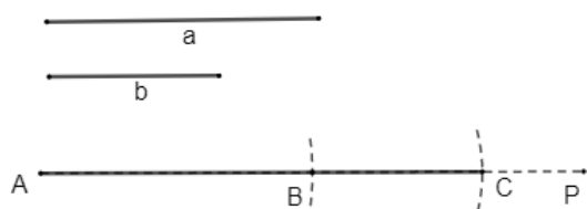
Figura 3.1: Soma dos segmentos de medidas a e b .
