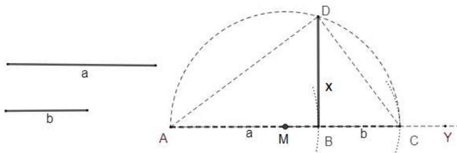
Figura 3.6: x = \sqrt{ab} .
