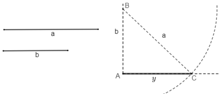
Figura 3.15: y = \sqrt{a^2 - b^2}
