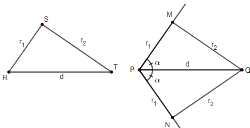
Figura 2.5: Triângulos congruentes
