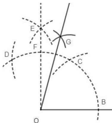
Figura 2.29: Ângulo de 75^\circ
