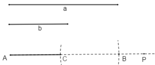
Figura 3.2: Diferença entre segmentos de medidas a e b .
