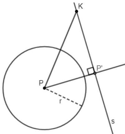
Figura 2.1: P' é externo à circunferência
