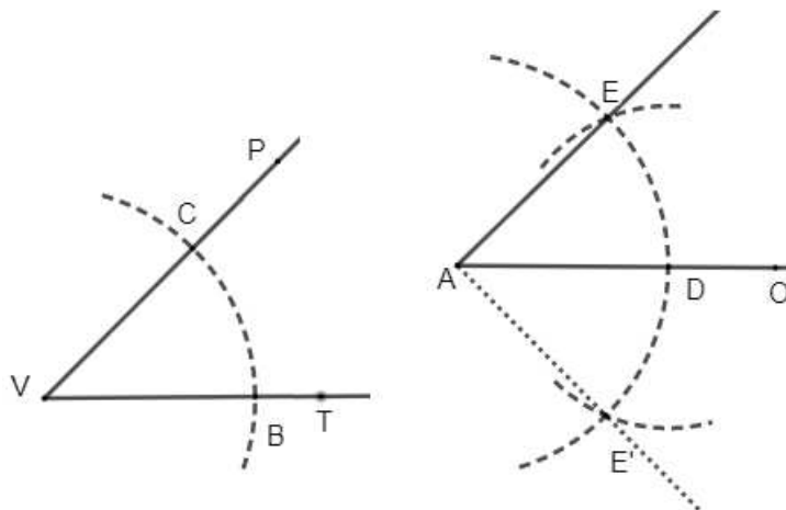
Figura 2.8: Transporte de ângulo
