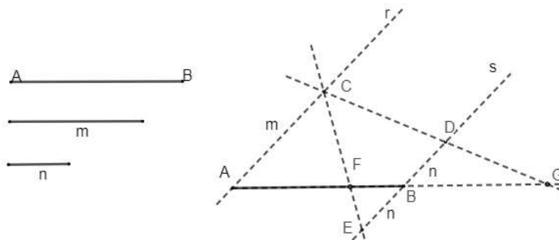
Figura 3.11: Divisão harmônica.
