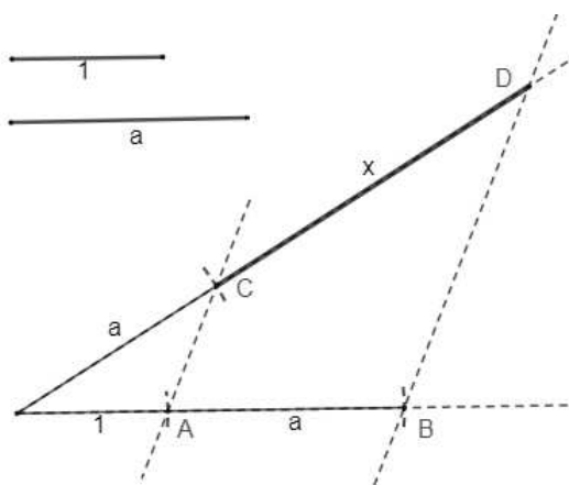
Figura 3.7: x = a^2 .
