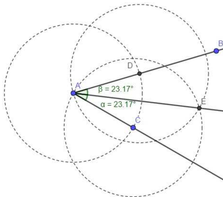
Figura 5.3: Atividade 3 - Bissetriz 2ª parte
