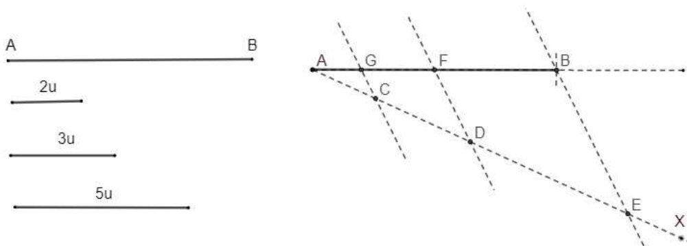
Figura 3.10: Segmento dividido em partes proporcionais a 2, 3 e 5.
