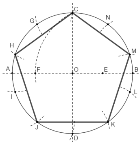
Figura 4.6: Pentágono regular inscrito na circunferência
