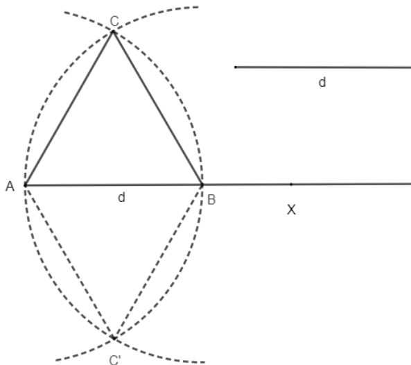
Figura 2.16: Triângulo equilátero
