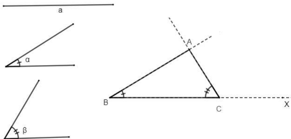
Figura 2.19: Triângulo conhecidas as medidas de dois ângulos e do lado adjacente a eles
