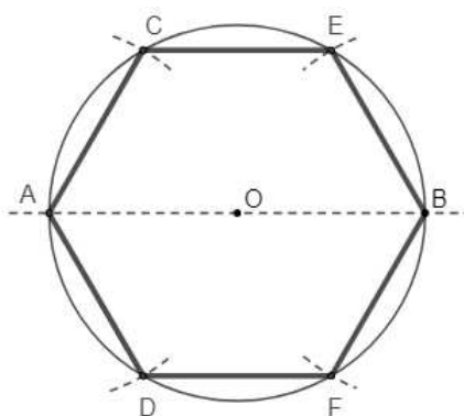
Figura 4.2: Hexágono regular inscrito na circunferência
