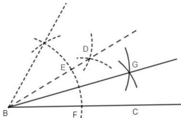
Figura 2.25: Ângulo de 15^\circ
