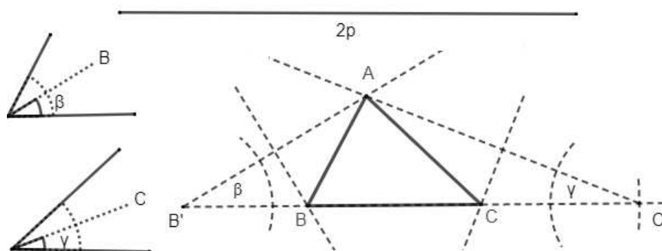
Figura 2.23: Triângulo conhecidos seu perímetro e dois de seus ângulos
