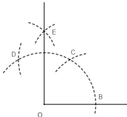
Figura 2.27: Ângulo de 90^\circ
