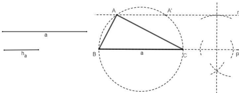
Figura 2.21: Triângulo retângulo conhecidas a hipotenusa e a altura relativa a ela
