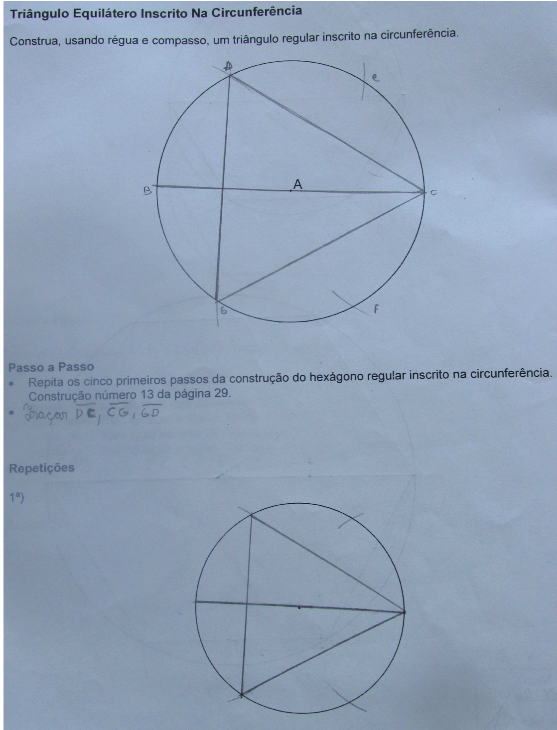
Figura A.5: Construção triângulo equilátero – Atividade 2
