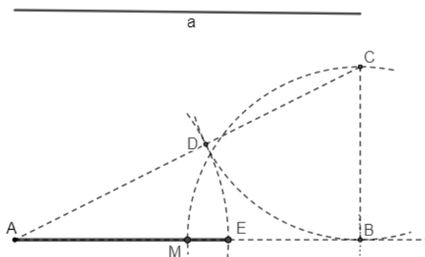
Figura 3.13: Seção áurea.
