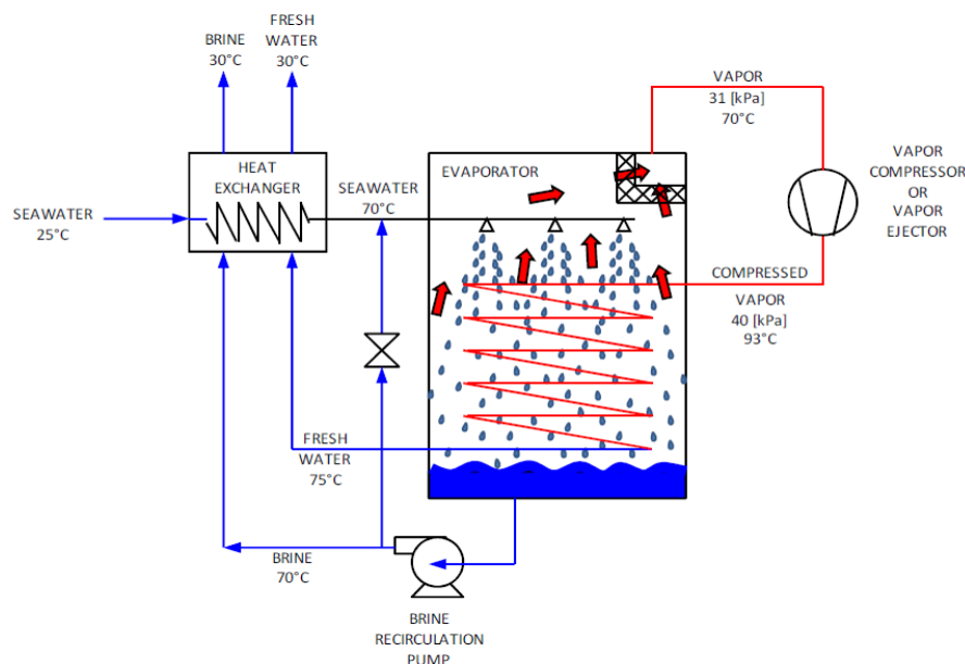
Figura 4: Diagrama de um Sistema de Dessalinização por Compressão de Vapor Mecânica - VC (BARRAZA, 2011).
