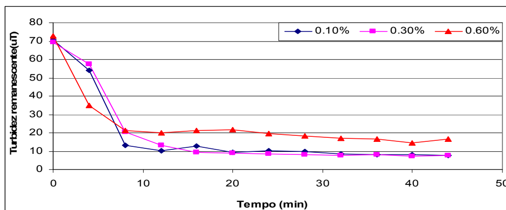
Figura 6.6: Ensaio de clarificação da ALF da ETA UFV, turbidez remanescente x tempo de sedimentação, coleta a 7 cm de altura, dose do polímero aniônico de 2 mg . L -1 tempo de mistura de 5 minutos e concentração de 0,1%, 0,3% e 0,6%.
