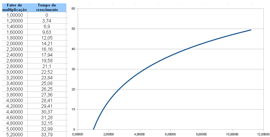
Figura 3.23: Gráfico do tempo em função da “população”.
