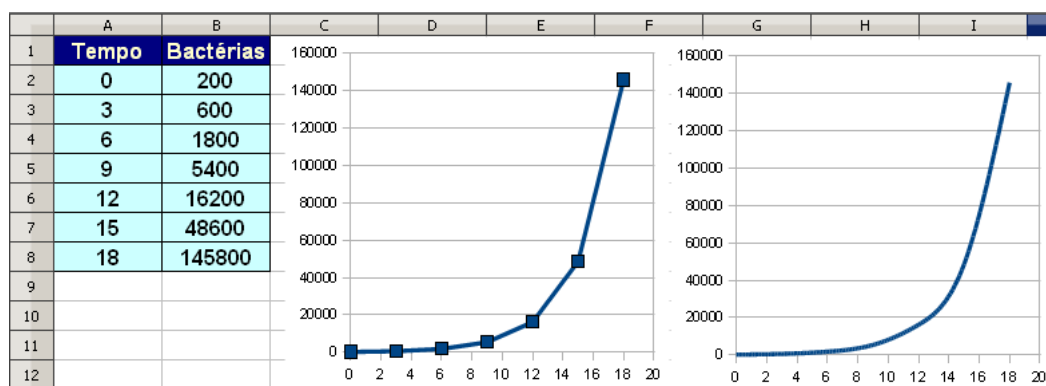
Figura 4.2: Gráficos da progressão geométrica e da suposta função.
