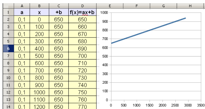
Figura 3.4: Gráfico de f(x) = 0,1x + 650 para 0 \leq x \leq 2900 .
