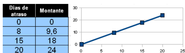
Figura 5.6: Tabela e gráfico do problema.
