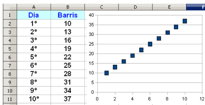
Figura 4.1: Tabela e gráfico da progressão aritmética.
