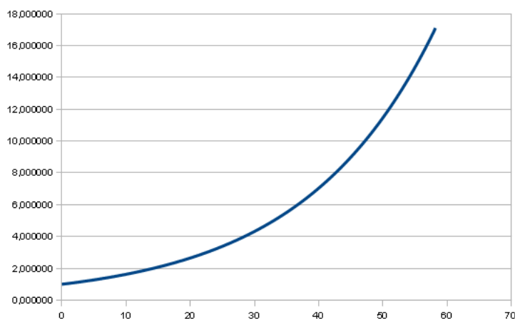
Figura 3.21: Gráfico da população de peixes em função do tempo.
