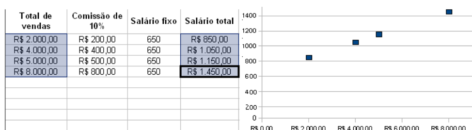
Figura 3.2: Tabela e Gráfico XY (Dispersão), somente pontos, para a coluna Salário total em função do Total de vendas.
