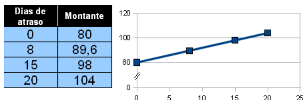
Figura 5.7: Tabela e gráfico do montante pago em função dos dias de atraso.
