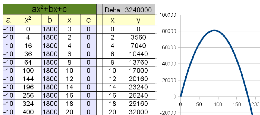
Figura 3.9: Construção do gráfico da função quadrática.
