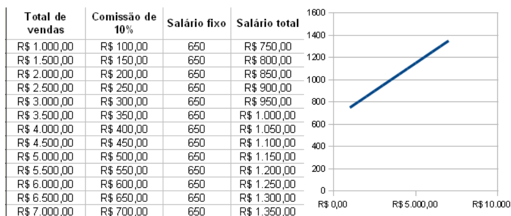
Figura 3.3: Tabela e gráfico somente linhas para o Salário total em função do total de vendas..
