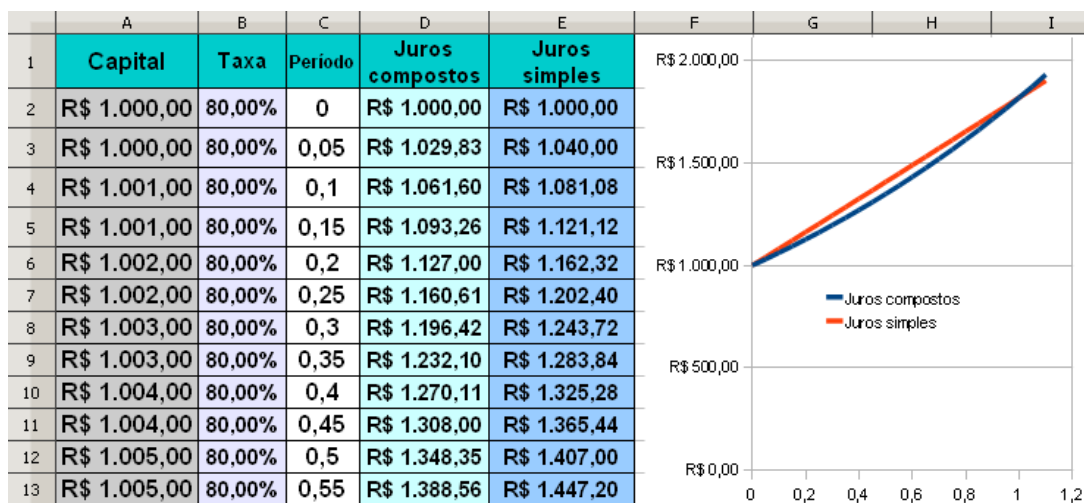
Figura 5.16: Comparação entre os montantes gerados no regime de capitalização simples e composta para um tempo menor que a unidade.
