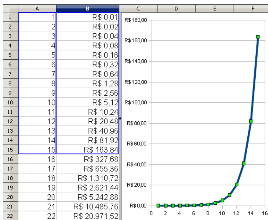
Figura 3.14: Gráfico da função do tipo exponencial para o problema do comerciante rico, representando os ganhos diários do 1º ao 15º dia.
