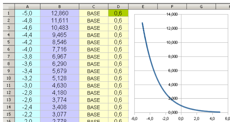
Figura 3.17: Tabela e gráfico dinâmico ao se alterar a base da função exponencial.
