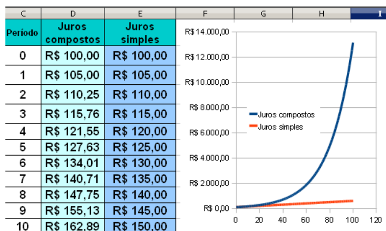
Figura 5.15: Tabela e gráficos de comparação dos montantes nos regimes de capitalização simples e composta.
