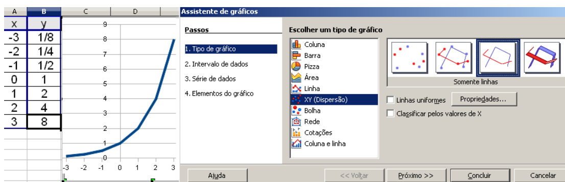
Figura 2.26: Usando o Assistente de gráfico para construção de gráfico de uma função exponencial a partir dos dados na tabela.
