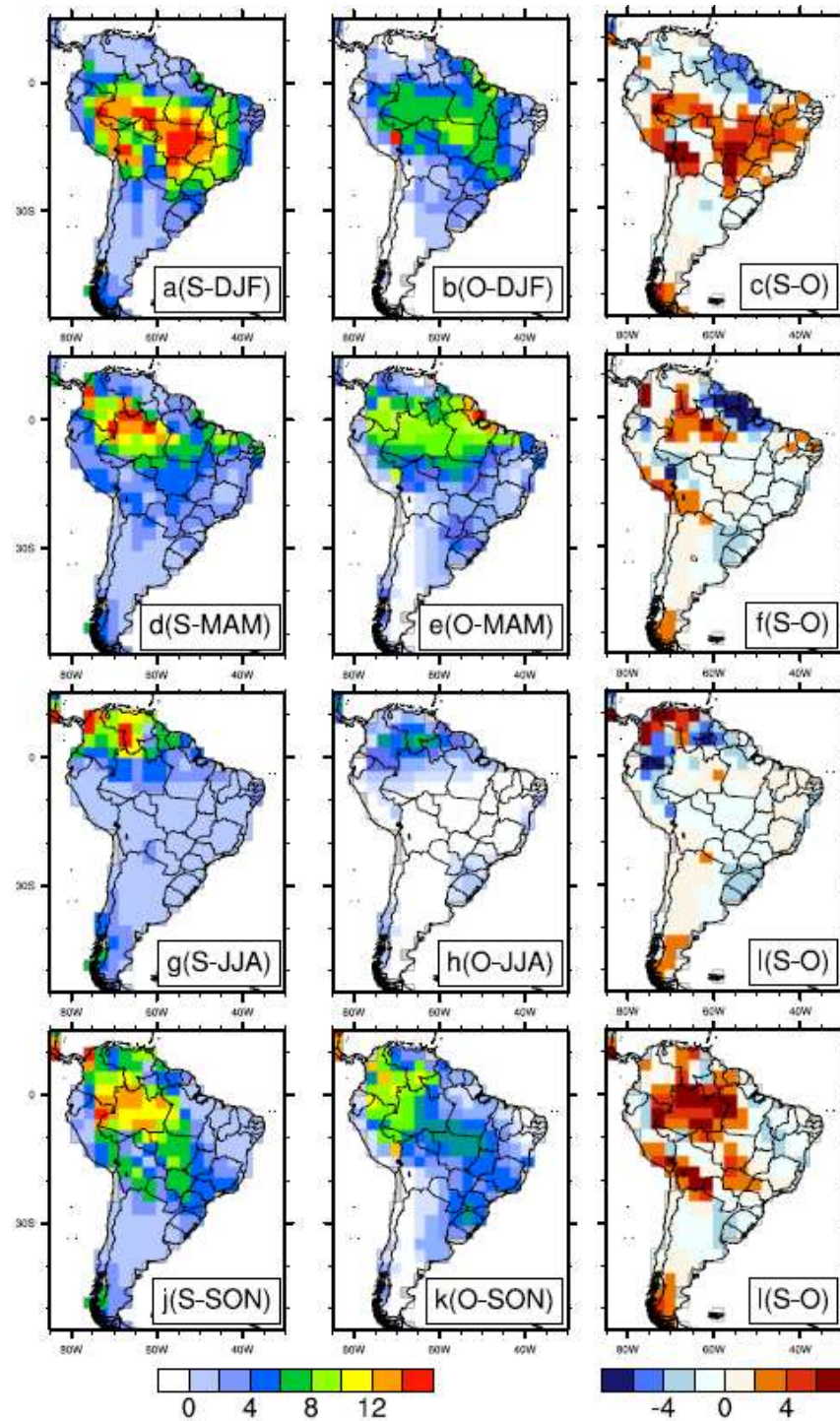
Figura 5. Resultados dos dados simulados (S), observados (O) e o erro de simulação (S-O) da precipitação sazonal média mensal (mm/dia) no período de 1961-1990.
