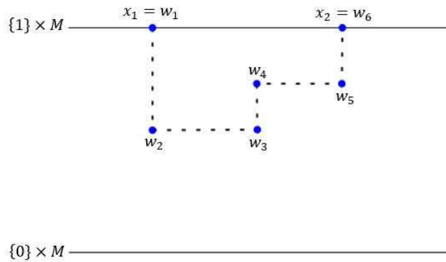
Figura 1.6: Cadeia entre x_1 e x_2 .
