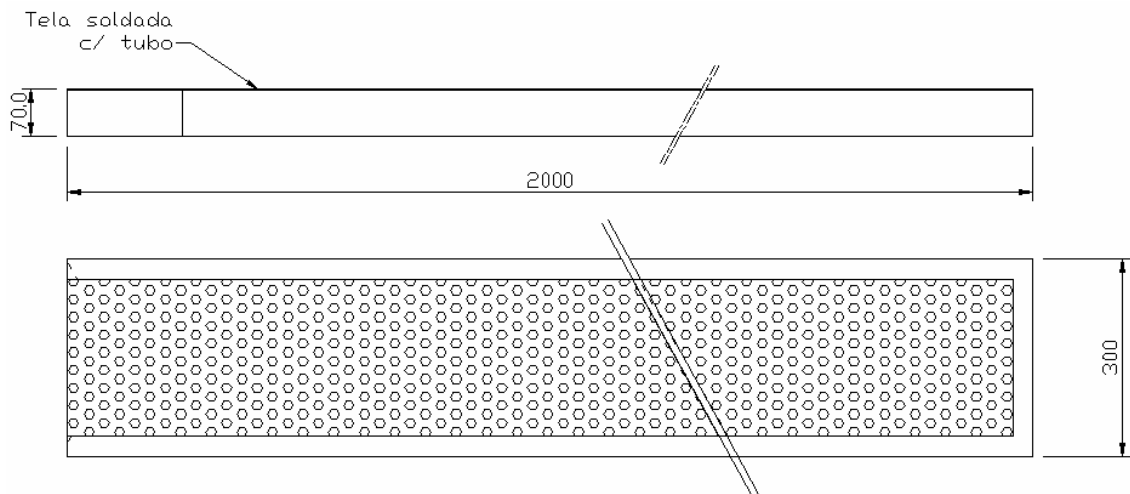
Figura 8 - Detalhe da peneira inferior da abanadora.
