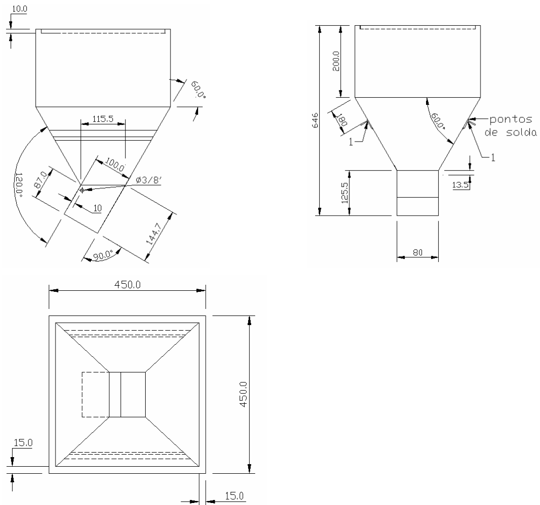
Figura 3 - Detalhe da moega de alimentação da abanadora.
