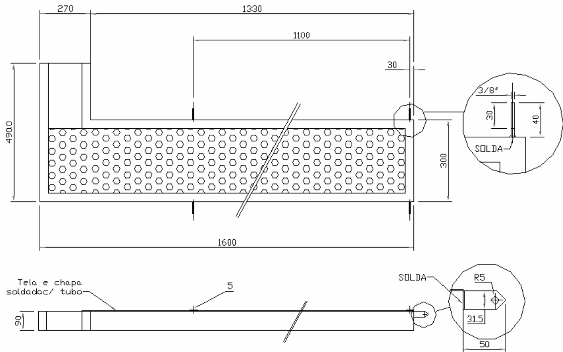
Figura 7 - Detalhe da peneira superior da abanadora.
