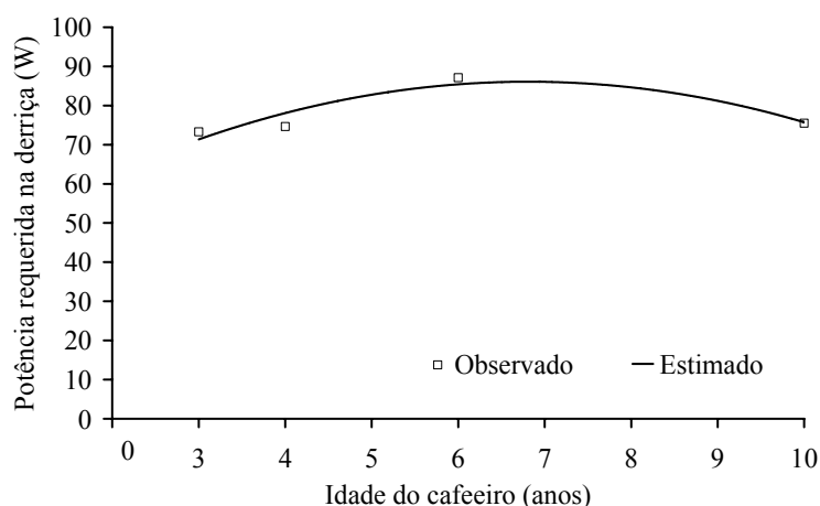
Figura 11 - Potência elétrica requerida na derriça em função da idade de cafeeiros Catuaí e Catucaí.
