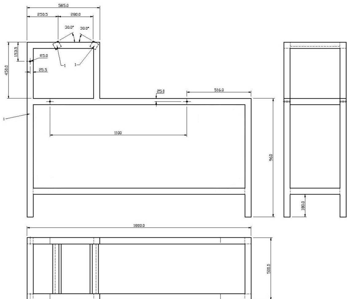
Figura 2 - Detalhe da estrutura da abanadora (chassi).
