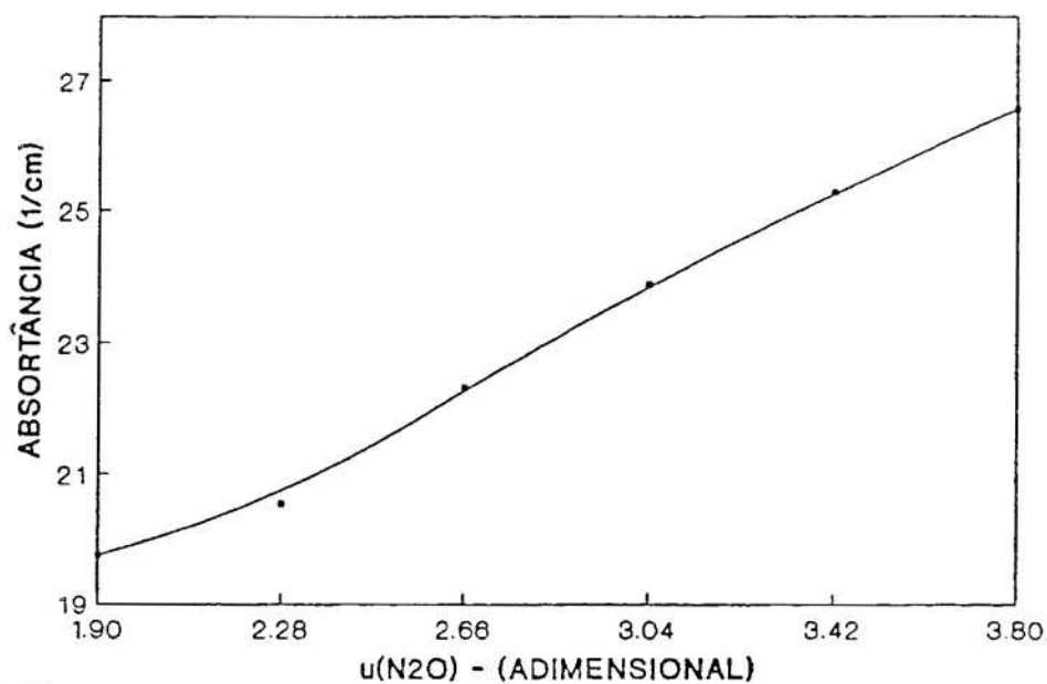
FIGURA 1B - Absortância Atmosférica na Banda de 7,8 \mu\text{m} do \text{N}_2\text{O} , em Função do Parâmetro de Espessura Ótica ( u ), para a Atmosfera-Padrão USA (1962).
