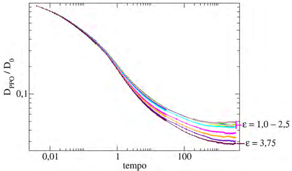
Figura 7.17: Coeficiente de difusão das unidades PPO dependendo do tempo para vários valores de \epsilon . Variação de \epsilon = 1,0 a \epsilon = 3,75 .
