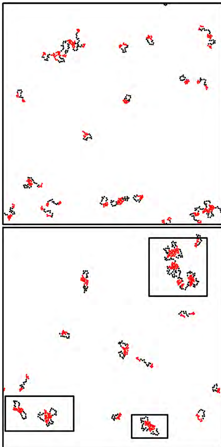
Figura 7.10: Imagem das estruturas formadas em \epsilon = 3,0 (acima) e \epsilon = 3,75 (abaixo). Em destaque estruturas micelares isoladas e agregadas.
