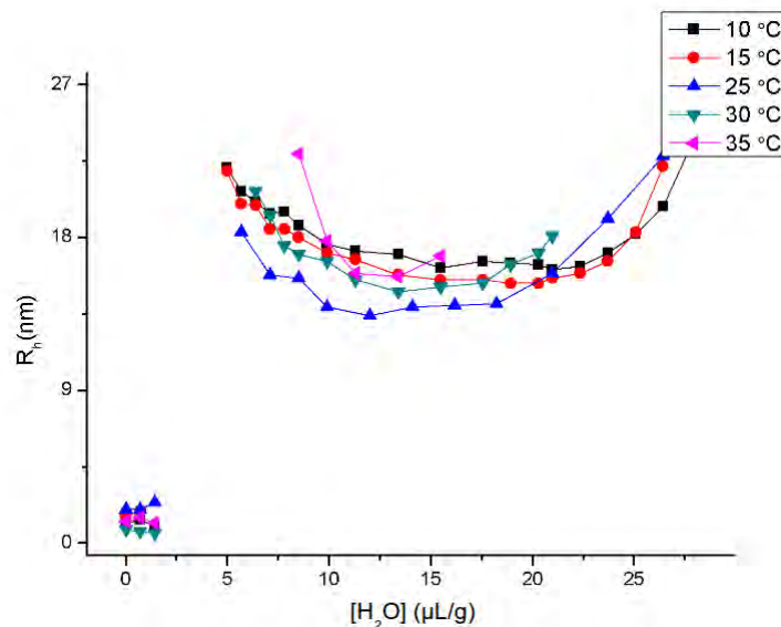
Figura 6.16: Raio hidrodinâmico aparente por volume de água adicionado em temperaturas diferentes. Não observou-se variações significativas dos tamanhos das estruturas.
