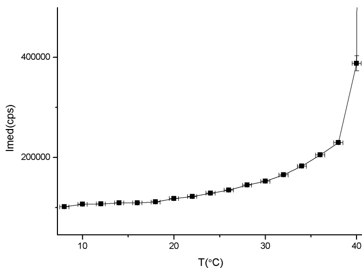
Figura 6.15: Intensidade média espalhada com variação de temperatura. Separação de fases observada também por volta de 38°C. A variação de intensidade antes do ponto de separação pode estar ligado à mudanças de índices de refração não consideradas.
