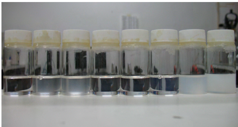
Figura 6.13: Algumas das amostras utilizadas nos experimentos de variação de temperatura. Da esquerda para direita as amostras apresentam concentrações de água: 2,14; 2,85; 3,56; 6,39; 11,30; 31,81 e 37,14 \mu\text{L/g} . As concentrações são dadas em \mu\text{L} de água por grama de solução. A foto foi tirada em temperatura ambiente de \approx 28^\circ\text{C} .
