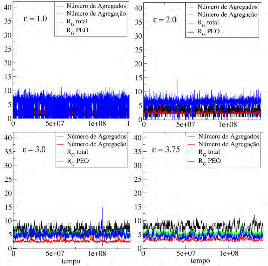
Figura 7.8: Mesmo gráfico do anterior desconsiderando-se as cadeias livres nas médias.
