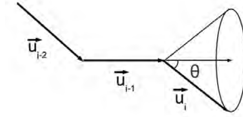
Figura 2.2: Modelo com dependência angular entre as ligações.
