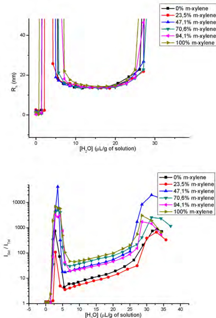
Figura 6.7: Medidas de R_h (cima) e intensidade média espalhada (normalizada) por concentração de água adicionada, com variação das proporções p -xileno e m -xileno. Nenhuma diferença relevante foi observada.
