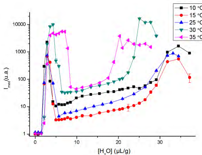
Figura 6.17: Intensidade média espalhada por volume de água adicionado em temperaturas diferentes. A dependência exponencial com a concentração foi observado para todas as amostras.
