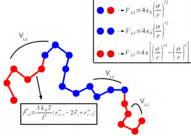
Figura 7.3: Interações Lennard-Jones para diferentes tipos de partículas. As interações também são as mesmas para cadeias diferentes.
