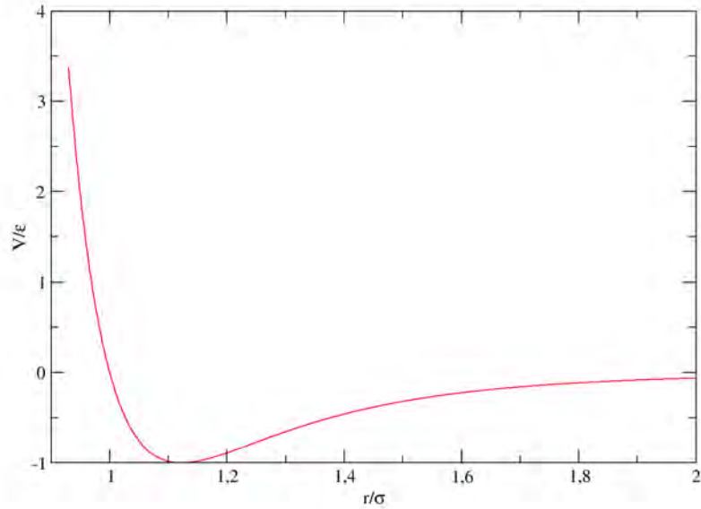
Figura 7.1: Potencial de Lennard-Jones (uma dimensão). Vemos que o gráfico apresenta um mínimo de potencial que é a distância de equilíbrio para as partículas.
