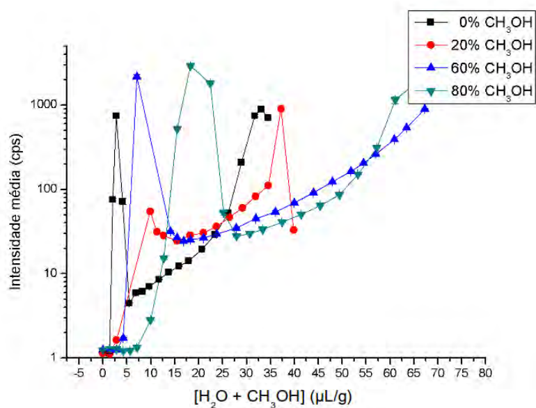
Figura 6.9: Medidas de intensidade média espalhada variando com quantidade de solução para soluções com diferentes proporções de água e metanol.
