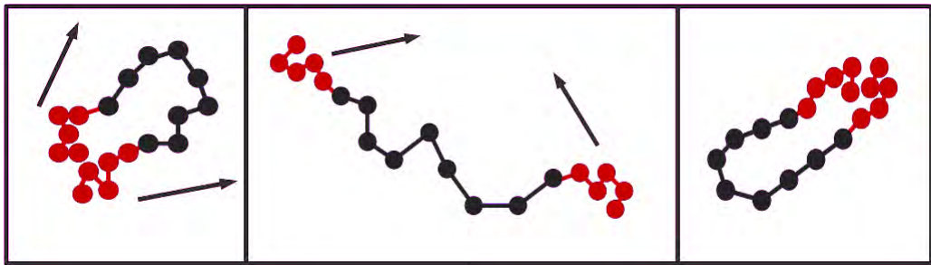
Figura 7.15: Esquema explicando o aumento do coeficiente de difusão do PEO para tempos da ordem de 10^2 .
