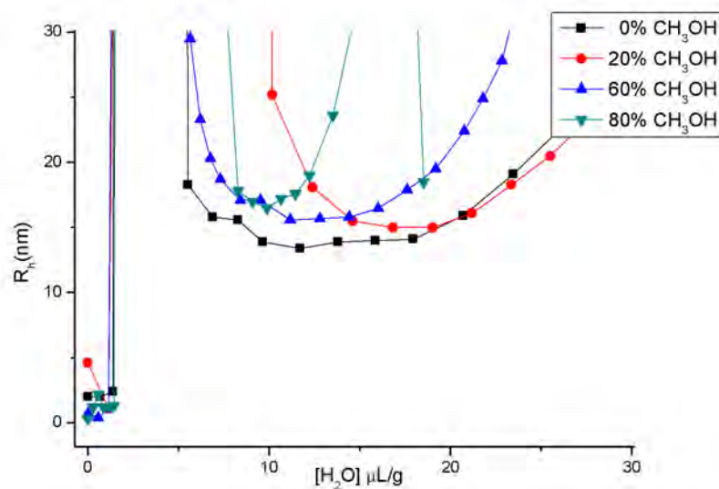
Figura 6.10: Medidas de raio hidrodinâmico variando com quantidade de solução para soluções com diferentes proporções de água e metanol. Gráficos relativos somente à quantidade de água.
