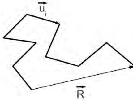
Figura 2.1: Cadeia livremente ligada e o vetor ponta-a-ponta.
