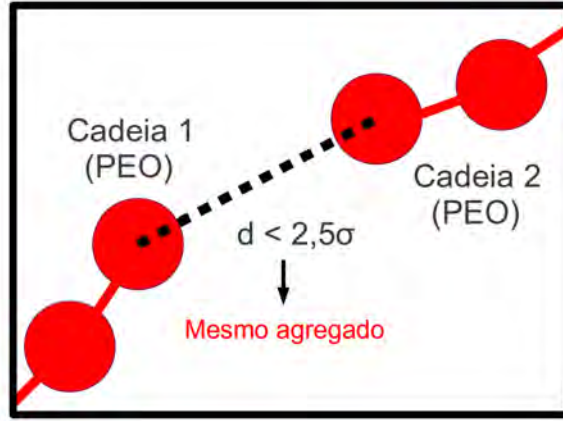
Figura 7.4: Critério adotado para considerarmos duas cadeias diferentes parte de um mesmo agregado.
