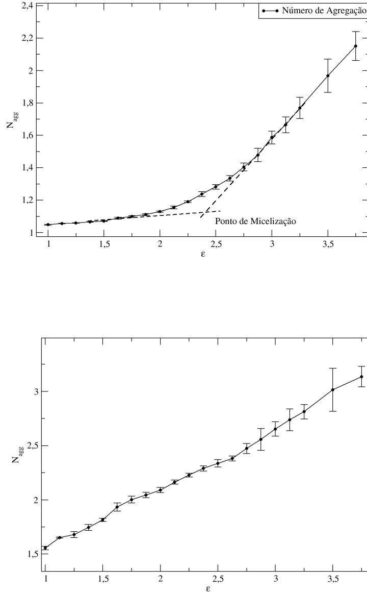
Figura 7.11: Número de agregação com a variação do parâmetro \epsilon . Considerando cadeias livres (acima) e desconsiderando cadeias livres (abaixo). Os comportamentos das curvas mostram-se significativamente diferentes.
