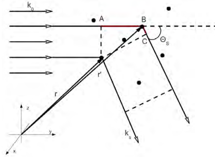
Figura 5.1: Esquema representativo do espalhamento elástico de luz em direção de espalhamento \Theta_s .
