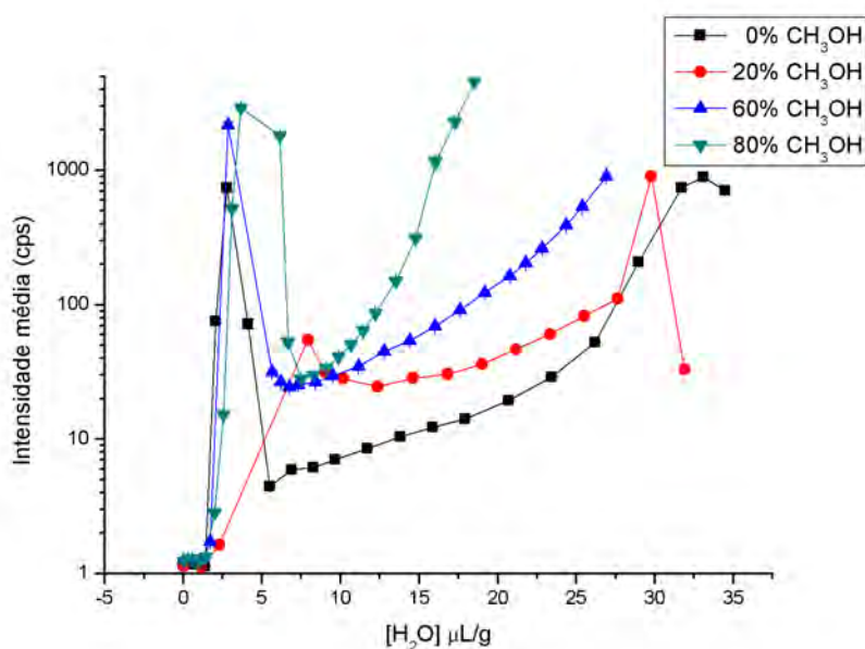
Figura 6.11: Medidas de intensidade média espalhada variando com quantidade de solução para soluções com diferentes proporções de água e metanol. Gráficos relativos somente à quantidade de água.
