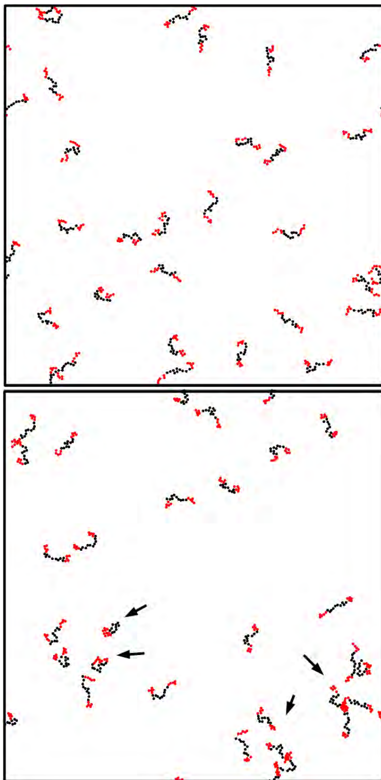
Figura 7.9: Imagem das estruturas formadas em \epsilon = 1,0 (acima) e \epsilon = 2,0 (abaixo). Os monômeros vermelhos são do tipo PEO e os pretos do tipo PPO. As setas mostram estruturas no formato de ferradura e algumas formando agregados abertos.
