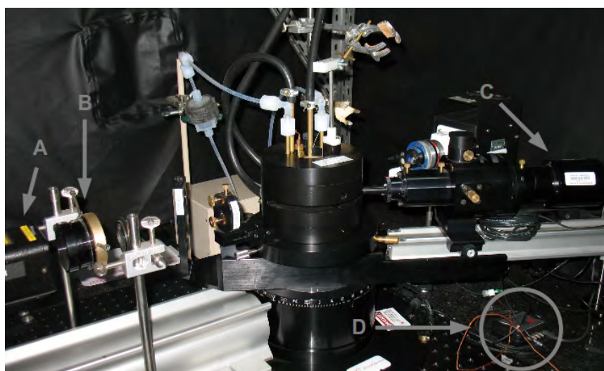
Figura 6.1: Equipamento de espalhamento utilizado nos experimentos. A) Parte do laser; B) sistema de polarizadores; C) detector e D) correlacionador.
