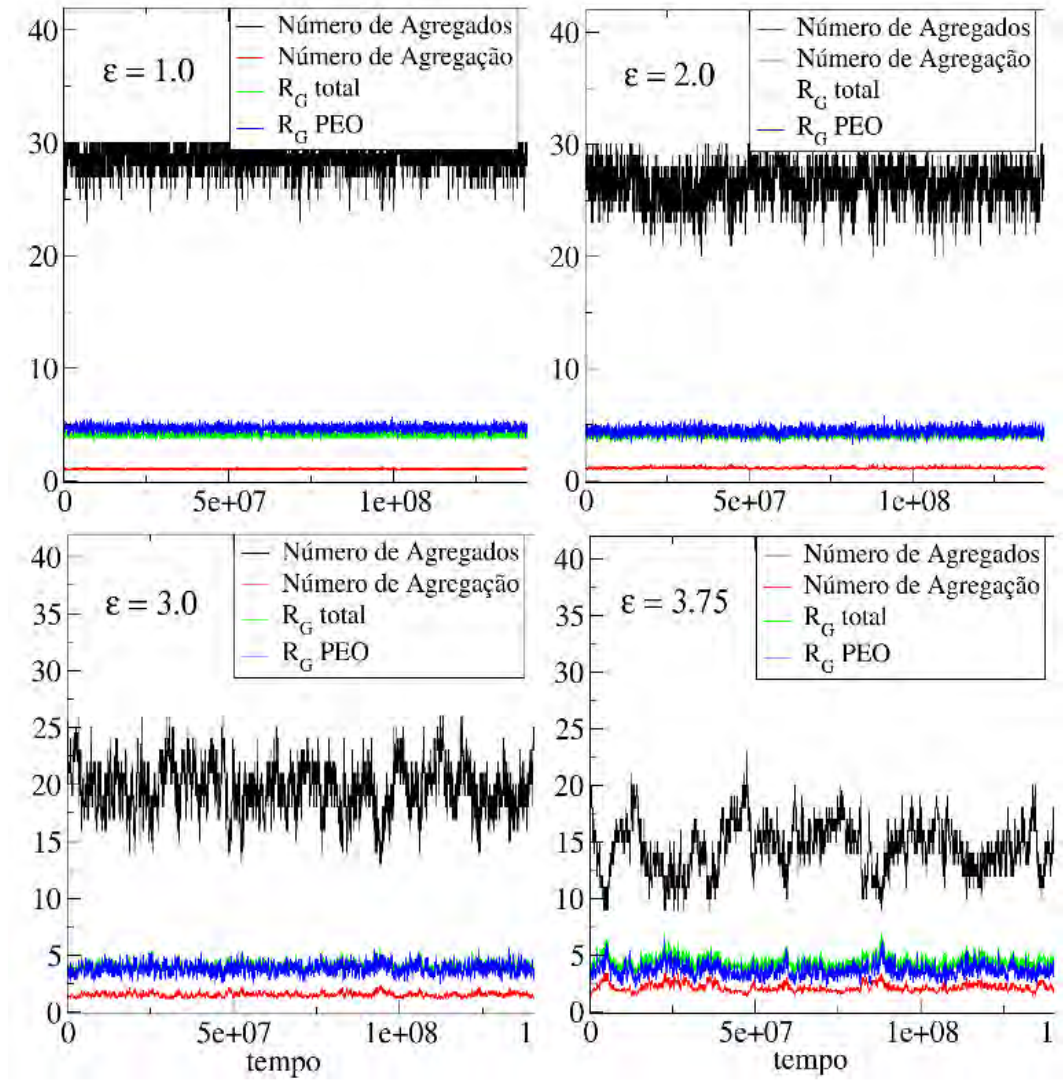
Figura 7.7: Cálculo dos valores de número de agregados, número de agregação, raio de giração total e raio de giração dos monômeros PEO considerando-se as cadeias livres nas médias.
