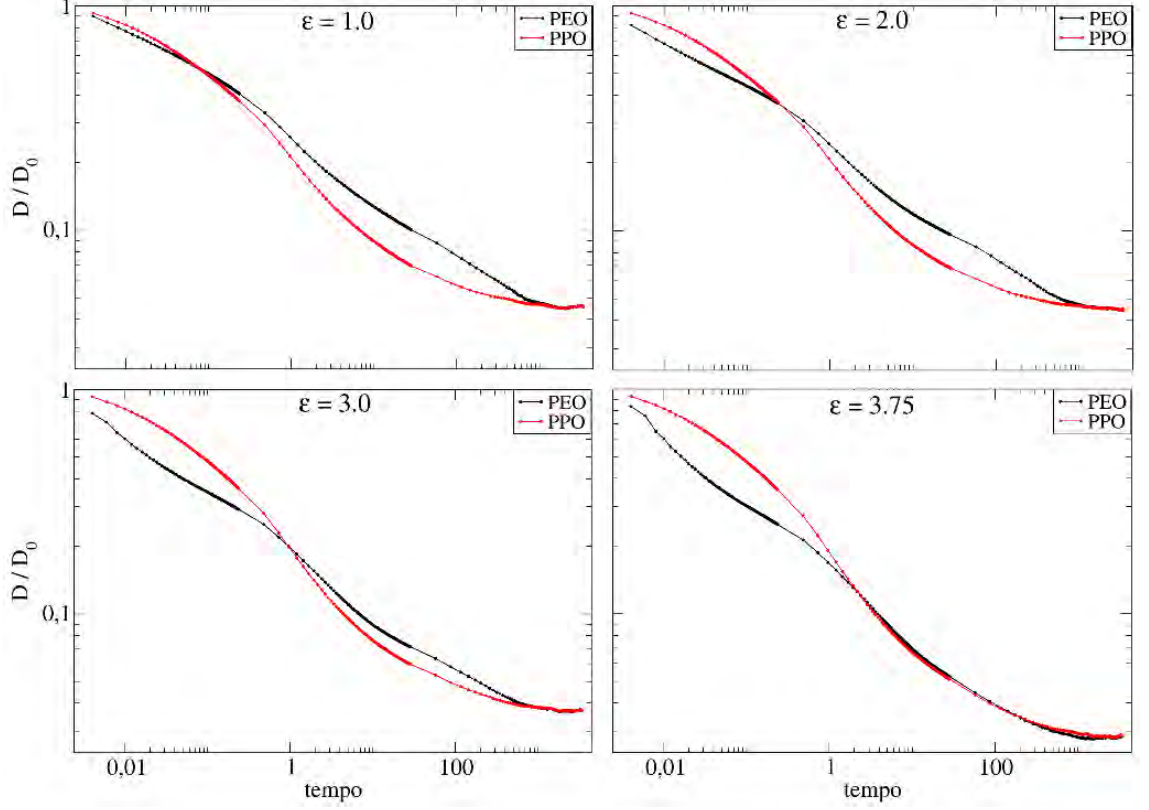
Figura 7.14: Coeficientes de difusão das cadeias tipo PEO e tipo PPO para diferentes \epsilon 's.
