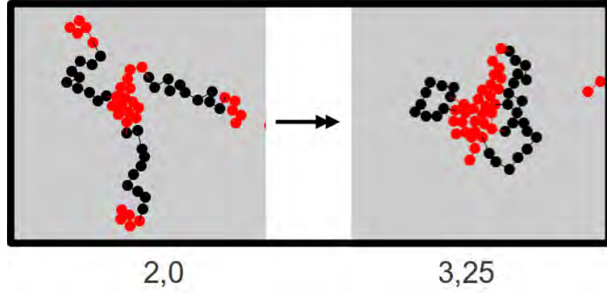
Figura 7.13: Processo de compactação das estruturas à medida que se aumenta a magnitude da interação.
