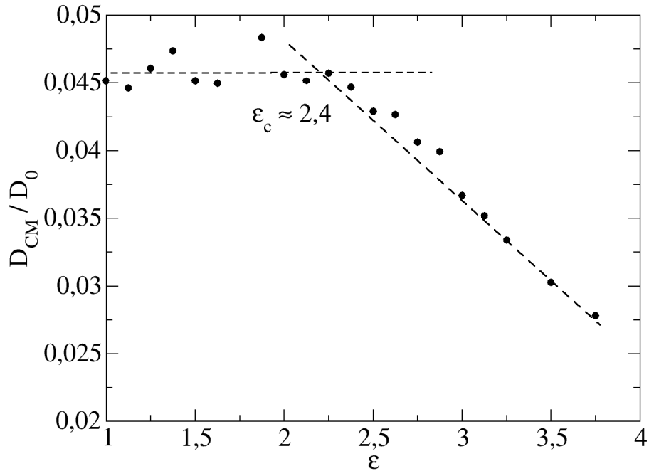
Figura 7.18: Coeficiente de difusão do centro de massa dos agregados variando com \epsilon . Novamente temos o \epsilon crítico próximo a 2,4.
