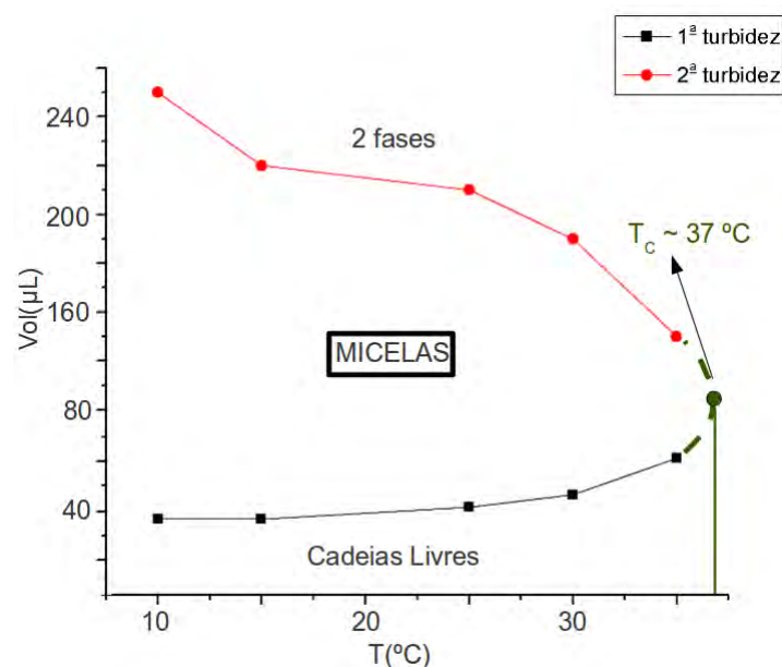
Figura 6.18: Curvas com volumes extremos de água para a formação das micelas. Abaixo da primeira curva e acima da segunda não há estruturas micelares. Temperatura crítica próximo a 37^\circ\text{C} .
