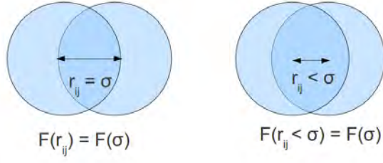
Figura 7.2: Esquema do corte para a interação de Lennard-Jones.
