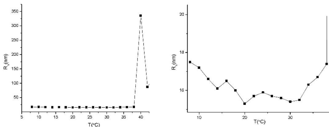
Figura 6.14: Raio hidrodinâmico aparente das estruturas em função da temperatura. Na direita uma ampliação do gráfico para a melhor visualização da mudança do raio. A separação de fases ocorre para uma temperatura próxima a 38°C.
