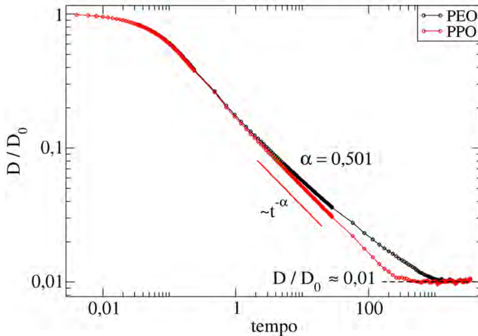
Figura 7.5: Coeficiente de difusão dos blocos EO e PO para uma cadeia livre de 100 unidades. Os resultados observados são esperados pelo modelo de Rouse para cadeias livres.
