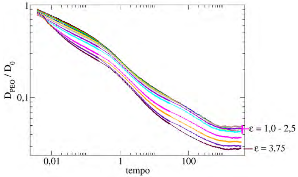
Figura 7.16: Coeficiente de difusão das unidades PEO dependendo do tempo para vários valores de \epsilon . Variação de \epsilon = 1,0 a \epsilon = 3,75 .
