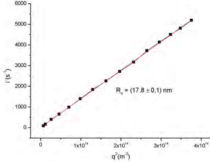
Figura 6.2: Gráfico de \Gamma por q^2 . Relação linear entre essas grandezas com o coeficiente de difusão como coeficiente angular.
