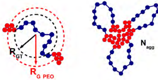
Figura 7.6: Esquema com as medidas de número de agregação e raios de giração total e somente das unidades das extremidades. Na figura o número de agregação da micela é 3.
