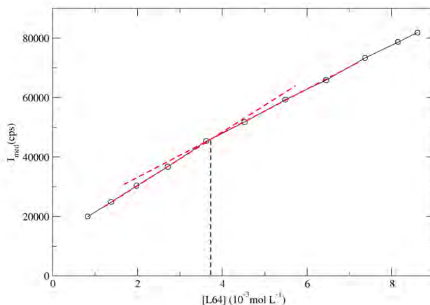
Figura 6.3: Intensidade de luz espalhada (não normalizada) com a variação da concentração de L64. Observamos uma mudança de regime próximo a 4 mM.
