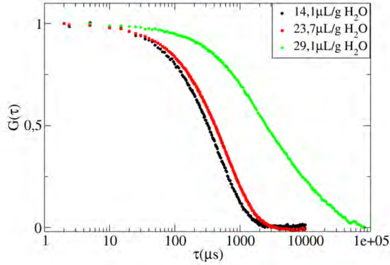
Figura 6.4: Funções de correlação normalizadas para 14,1, 23,7 e 29,1 \mu L/g de água.
