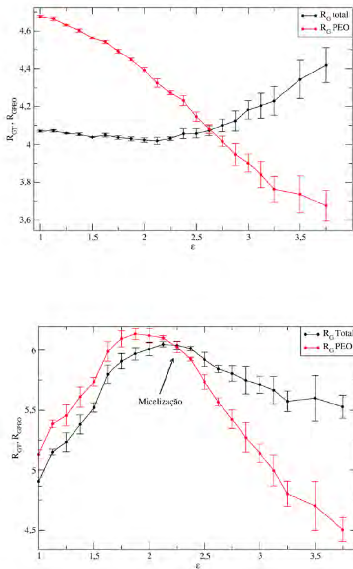
Figura 7.12: Raios de giração de toda a cadeia e somente dos monômeros do tipo PEO (extremidade). Considerando-se cadeias livres (acima) e desconsiderando-se as mesmas (abaixo).
