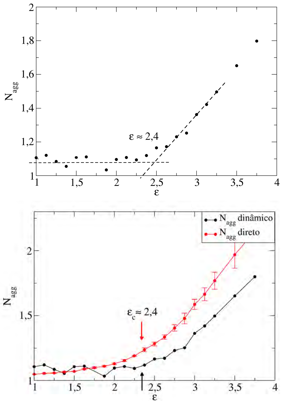
Figura 7.19: Número de agregação médio das estruturas variando com \epsilon . Superior: medidas via coeficiente de difusão. Inferior: comparação entre a medida via coeficiente de difusão e a medida direta.
