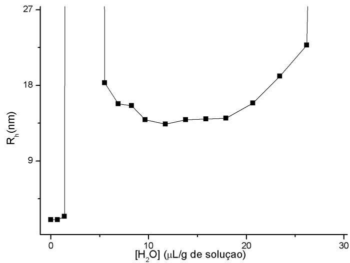
Figura 6.5: Dependência de R_h aparente com a concentração.
