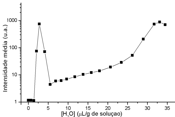
Figura 6.6: Medida de intensidade média espalhada por concentração de água adicionada.
