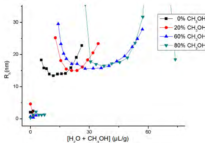
Figura 6.8: Medidas de raio hidrodinâmico variando com quantidade de solução para soluções com diferentes proporções de água e metanol.
