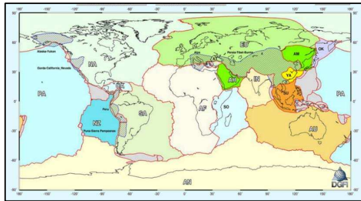
Figura 12 - Placas tectônicas e zonas de deformação segundo o modelo APKIM2005.
