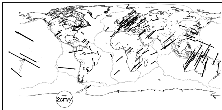
Figura 6 - Vetores velocidades das estações utilizadas na estimação dos vetores de Euler.
