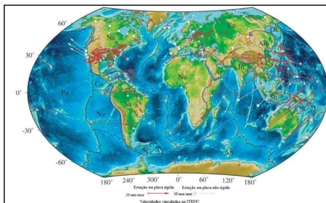
Figura 18 - Velocidades horizontais no ITRF97 segundo o modelo REVEL2000. Fonte: Sella, Dixon e Mao (2002).
