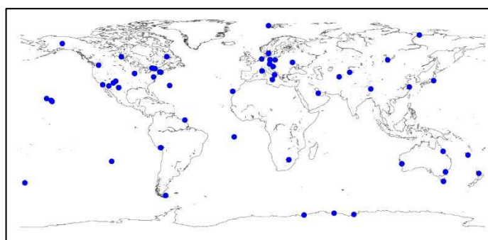
Figura 3 - Estações empregados na estimativa dos parâmetros de transformação de ITRF2005 para ITRF2000.
