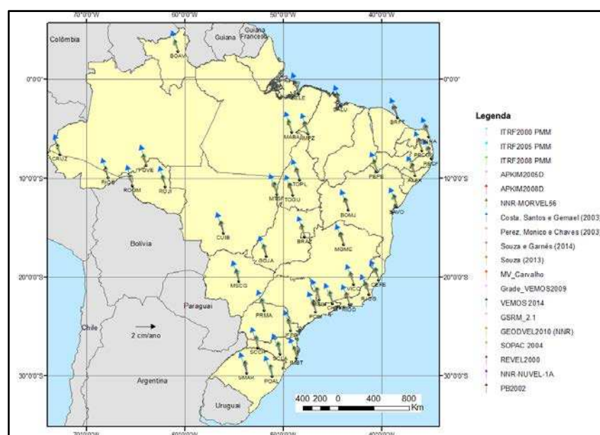
Figura 26 - Velocidades das estações obtidas com 19 modelos de movimento da placa SOAM.
