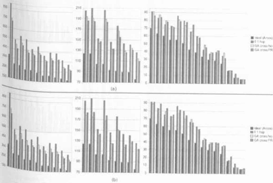
Figura 5.10. Algoritmo Genético: (a) Grupo Grande, a heurística GA crossover por PR ficou 61,54% acima do número mínimo possível de arcos; (b) Grupo Pequeno, a heurística GA cross nó ficou 53,99% acima do número mínimo possível de arcos.
