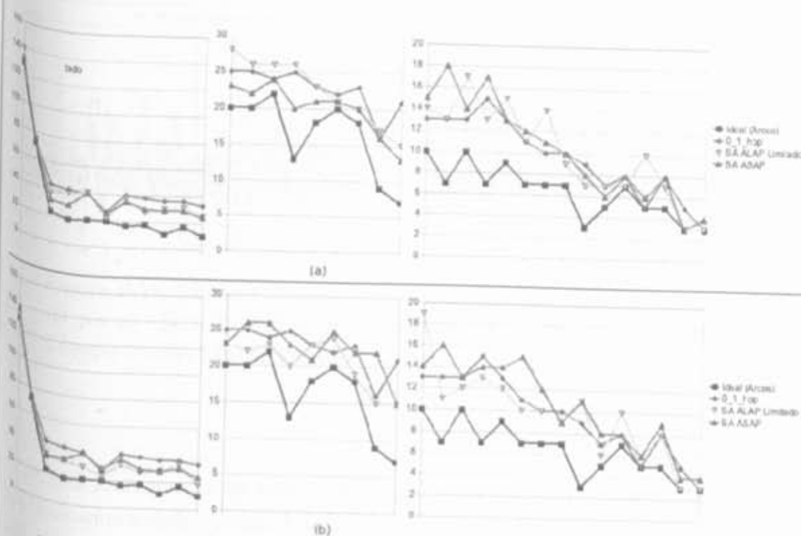
Figura B.16. Simulated Annealing: (a) Grupo Grande, a heurística SA ASAP ficou 36,45% acima do número mínimo possível de arcos do caminho crítico; (b) Grupo Pequeno, a heurística SA ALAP limitado ficou 31,94% acima do número mínimo possível de arcos do caminho crítico.
