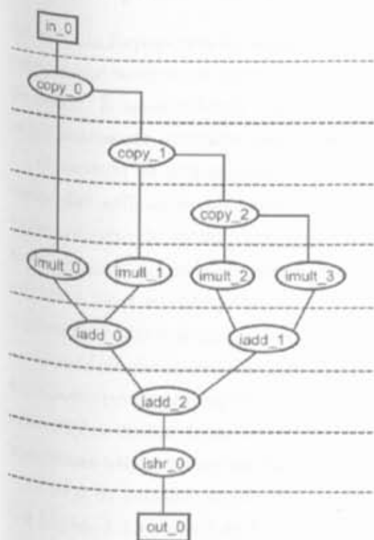
Figura 4.5. Algoritmo ALAP aplicado ao fluxo de dados do FIR 4.
