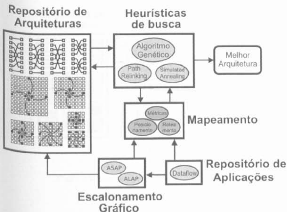
Figura 4.1. Gerador de Arquiteturas
