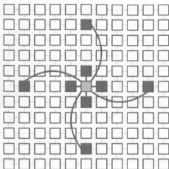
Figura 3.2. Saltos 0_3_hop.
