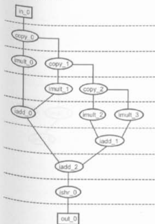
Figura 4.4. Algoritmo ASAP aplicado ao fluxo de dados do FIR 4.
