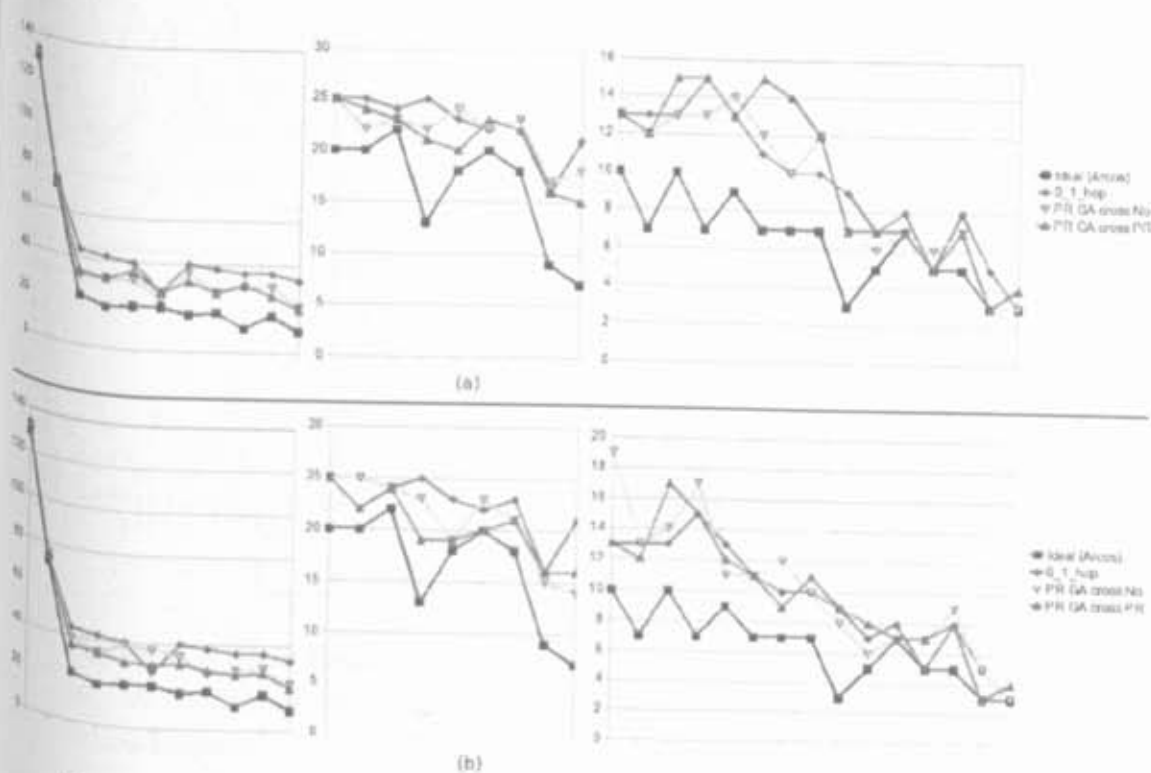
Figura B.8. Path Relinking: (a) Grupo Grande, a heurística PR GA crossover não ficou 34,62% acima do número mínimo possível de arcos do caminho crítico; (b) Grupo Pequeno, a heurística PR GA crossover PR ficou 33,44% acima do número mínimo possível de arcos do caminho crítico.
