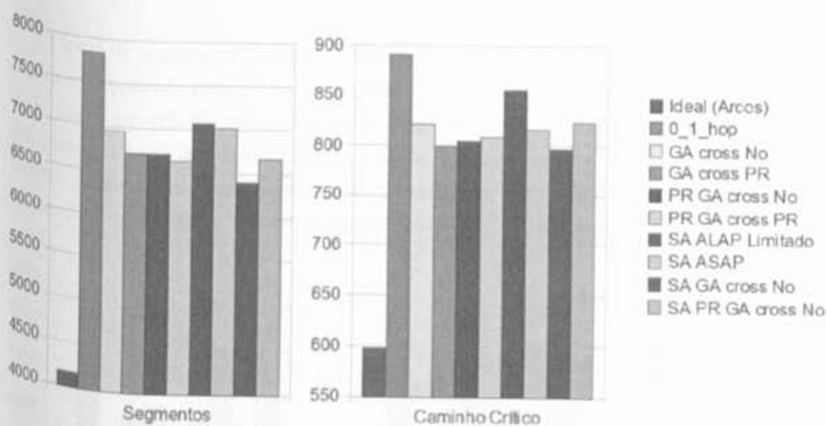
Figura 5.14. Gráficos com as variações do número total de segmentos e do número de segmentos dos caminhos críticos.
