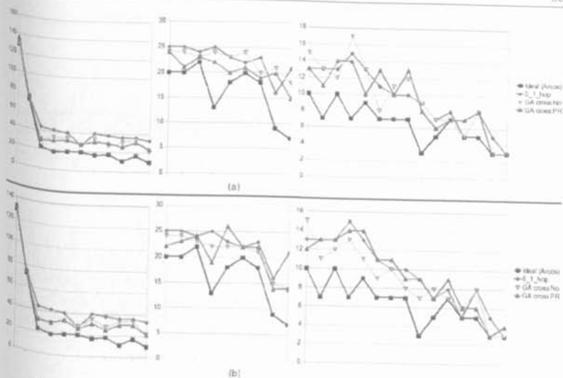
Figura B.1. Algoritmo Genético: (a) Grupo Grande, a heurística GA crossover PR ficou 33,61% acima do número mínimo possível de arcos do caminho crítico; (b) Grupo Pequeno, a heurística GA crossover PR ficou 34,62% acima do número mínimo possível de arcos do caminho crítico.
