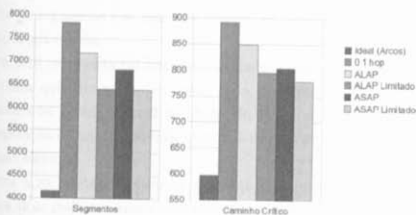
Figura 5.18. Gráficos com as variações do número total de segmentos e do número de segmentos dos caminhos críticos.
