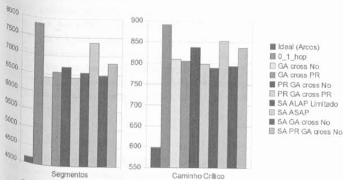
Figura 5.15. Gráficos com as variações do número total de segmentos e do número de segmentos dos caminhos críticos.
