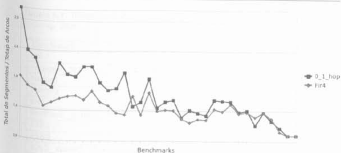
Figura 5.3. Gráfico de comparação entre 0_1_hop e a melhor arquitetura obtida para o FIR 4.
