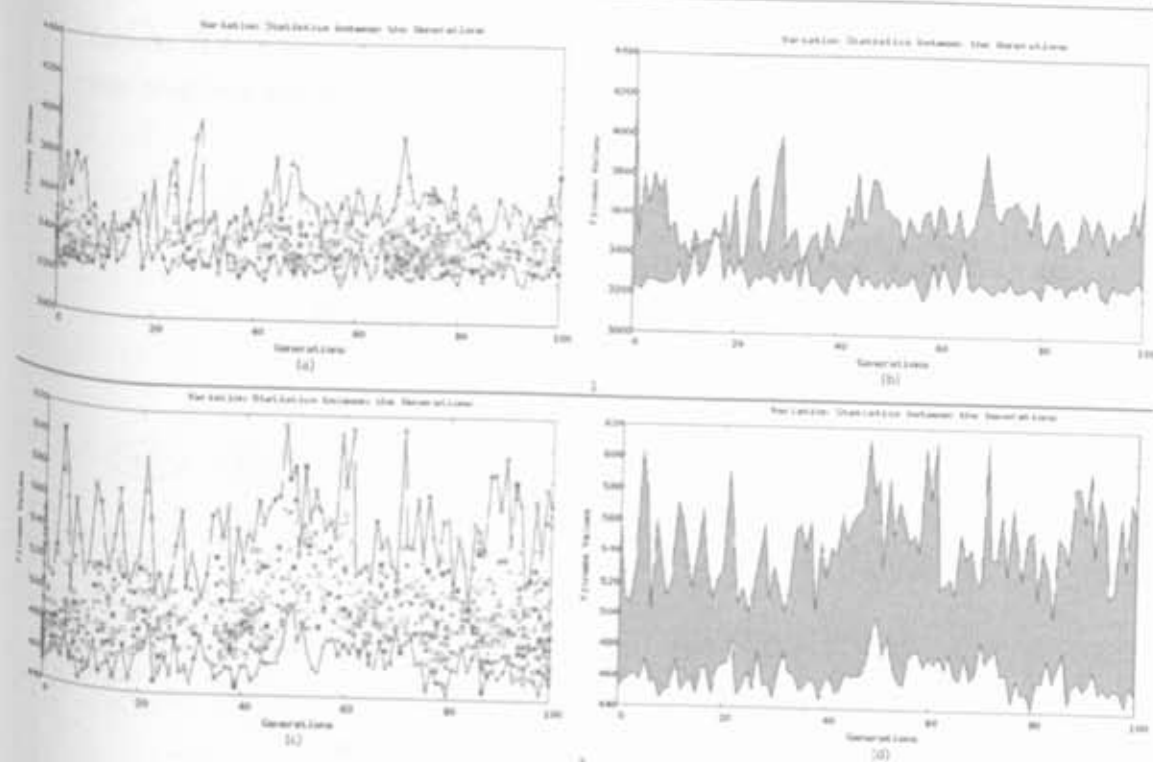
Figura B.2. Algoritmo Genético com crossover por nó – (a) e (c) Gráficos de Concentração; (b) e (d) Gráficos Estatísticos: 1 Grupo Grande; 2 Grupo Pequeno.
