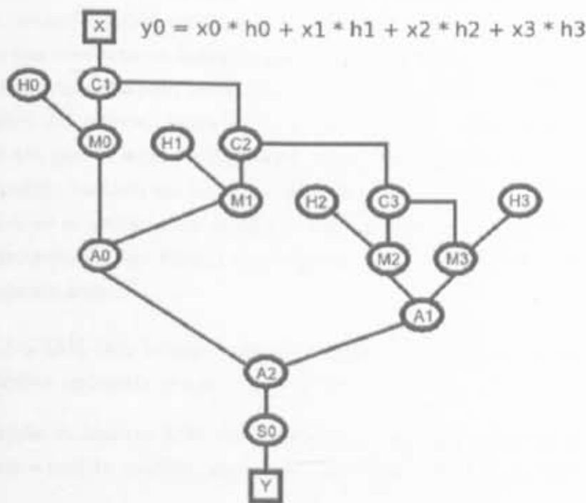
Figura 3.1. Grafo FIR de ordem 4.
