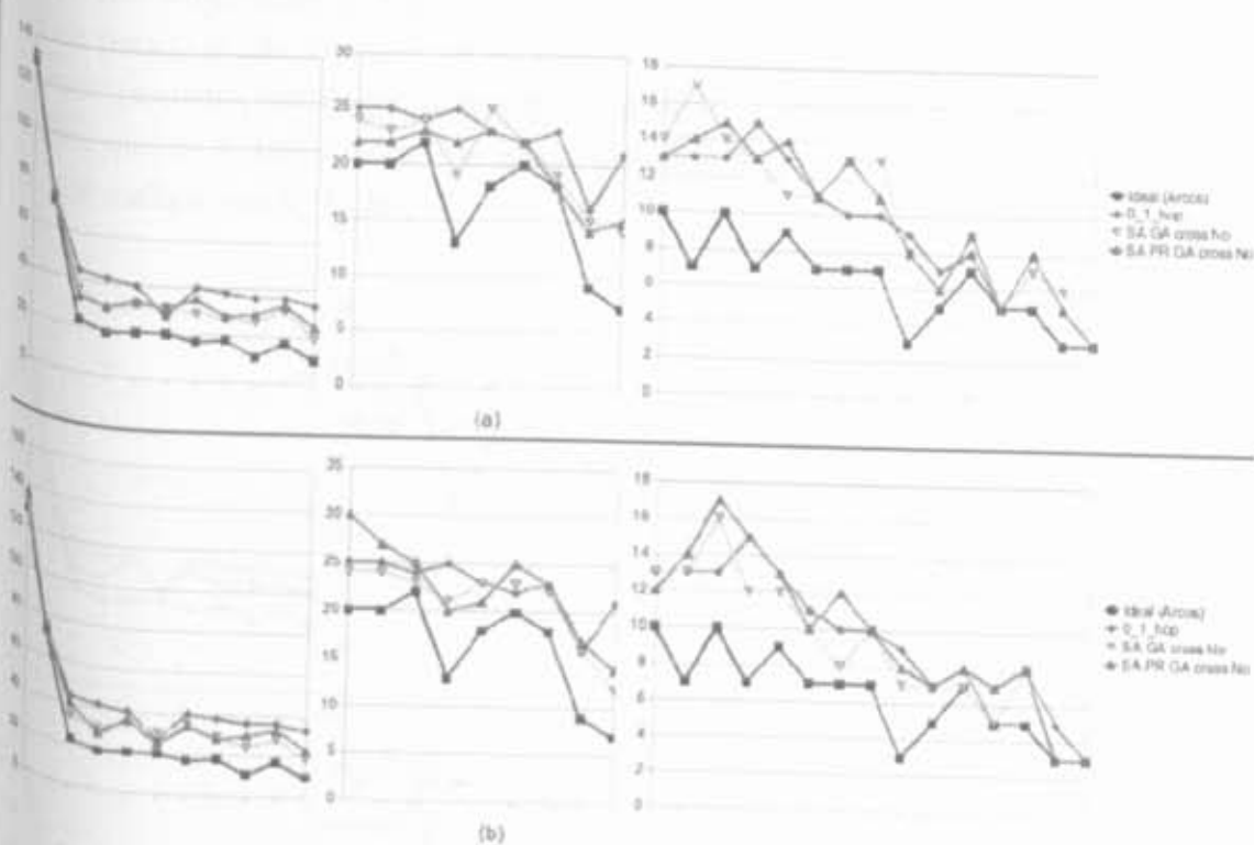
Figura B.15. Simulated Annealing: (a) Grupo Grande, a heurística SA GA crossover não ficou 33,28% acima do número mínimo possível de arcos do caminho crítico; (b) Grupo Pequeno, a heurística SA GA crossover não ficou 32,78% acima do número mínimo possível de arcos do caminho crítico.
