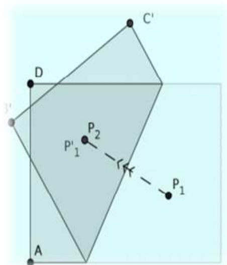
Figura 2.3: Axioma 2
