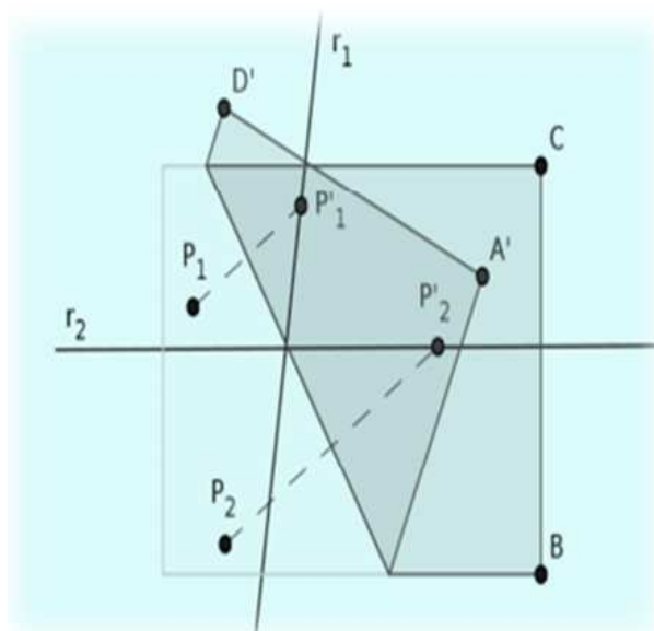
Figura 2.7: Axioma 6
