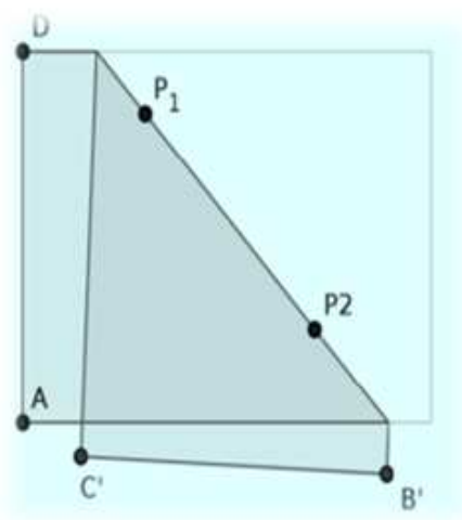
Figura 2.2: Axioma 1
