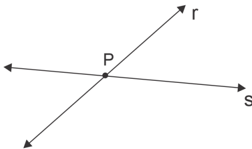
Figura 3.10: Retas Concorrentes
