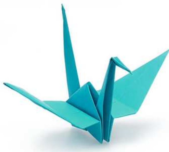
Figura 2.1: Tsuru
