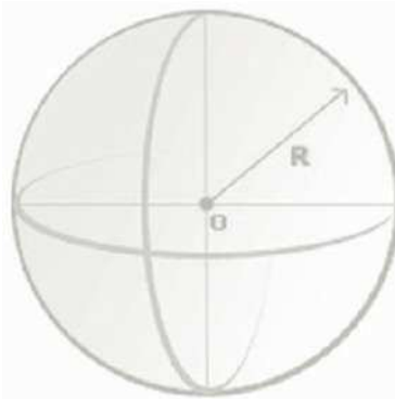
Figura 3.7: Superfície Esférica
