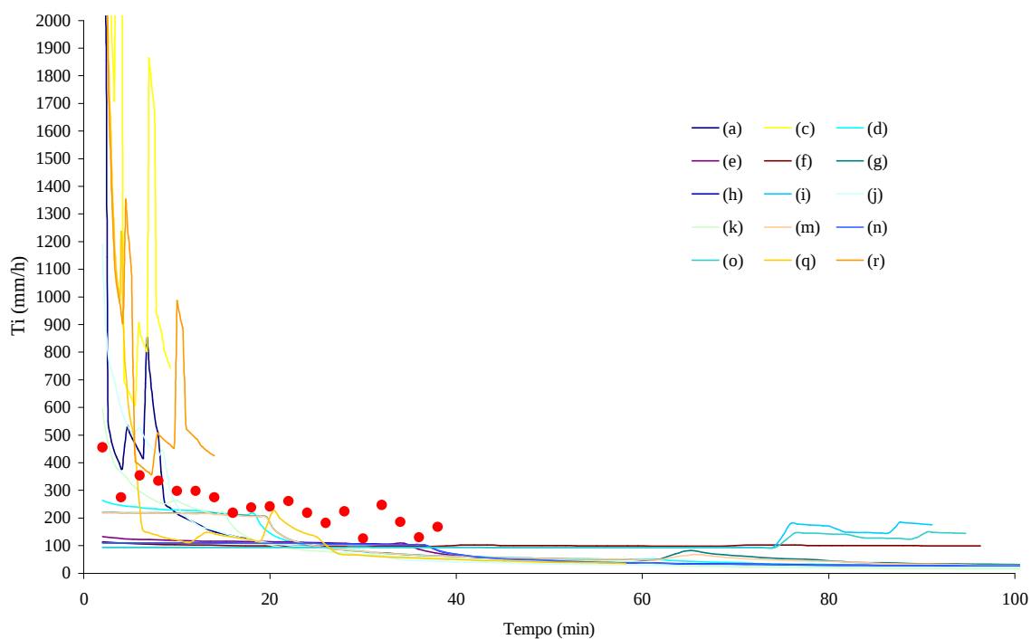
Figura 5D – Taxa de infiltração medida e simulada para a coluna 5, sendo \theta_w igual a 0,84 \theta_s para os três horizontes.
