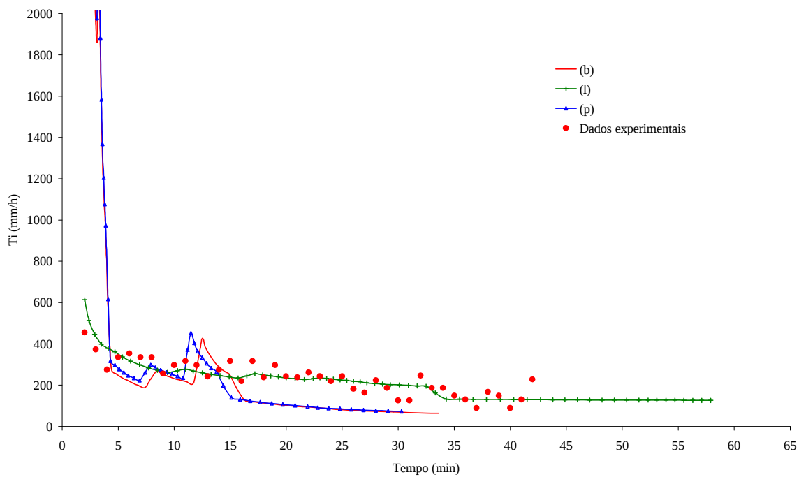
Figura 23 – Taxa de infiltração medida e simulada para a coluna 5, sendo \theta_w igual a 0,84 \theta_s para os três horizontes.
