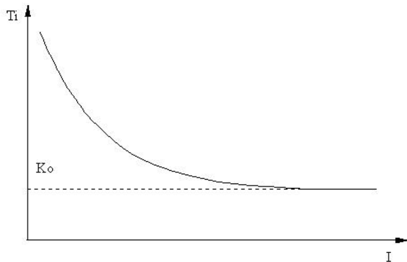
Figura 5 – Curva representativa da taxa de infiltração em função da infiltração acumulada obtida a partir da equação de Green-Ampt.
