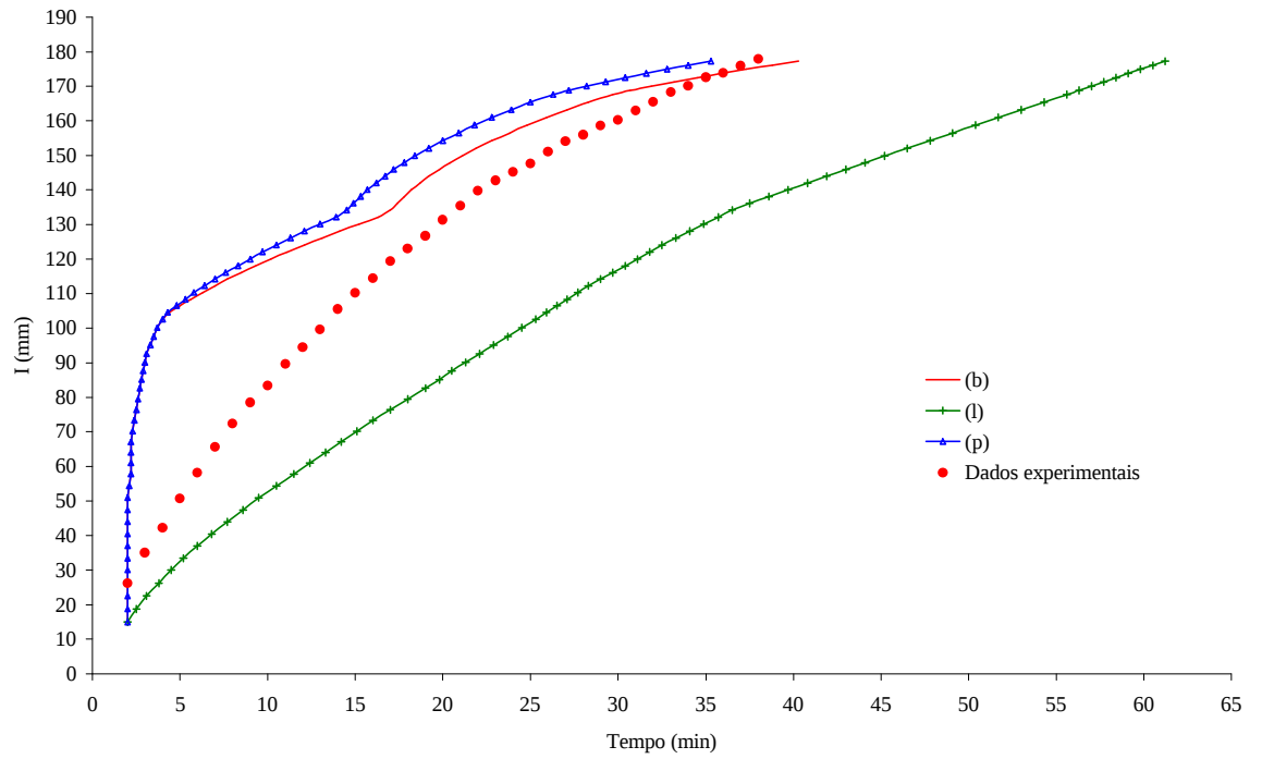
Figura 26 – Infiltração acumulada medida e simulada para a coluna 3, sendo \theta_w igual a 0,86 \theta_s para os três horizontes.
