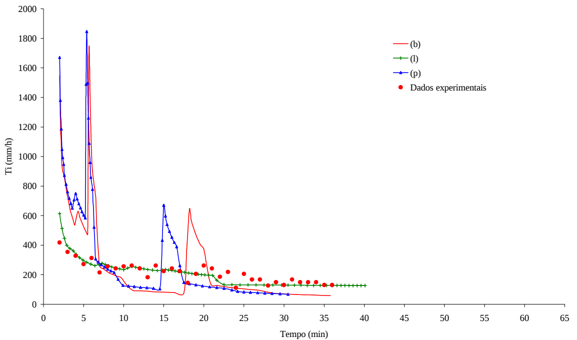
Figura 19 – Taxa de infiltração medida e simulada para a coluna 1, sendo \theta_w igual a 0,81 \theta_s para os três horizontes.
