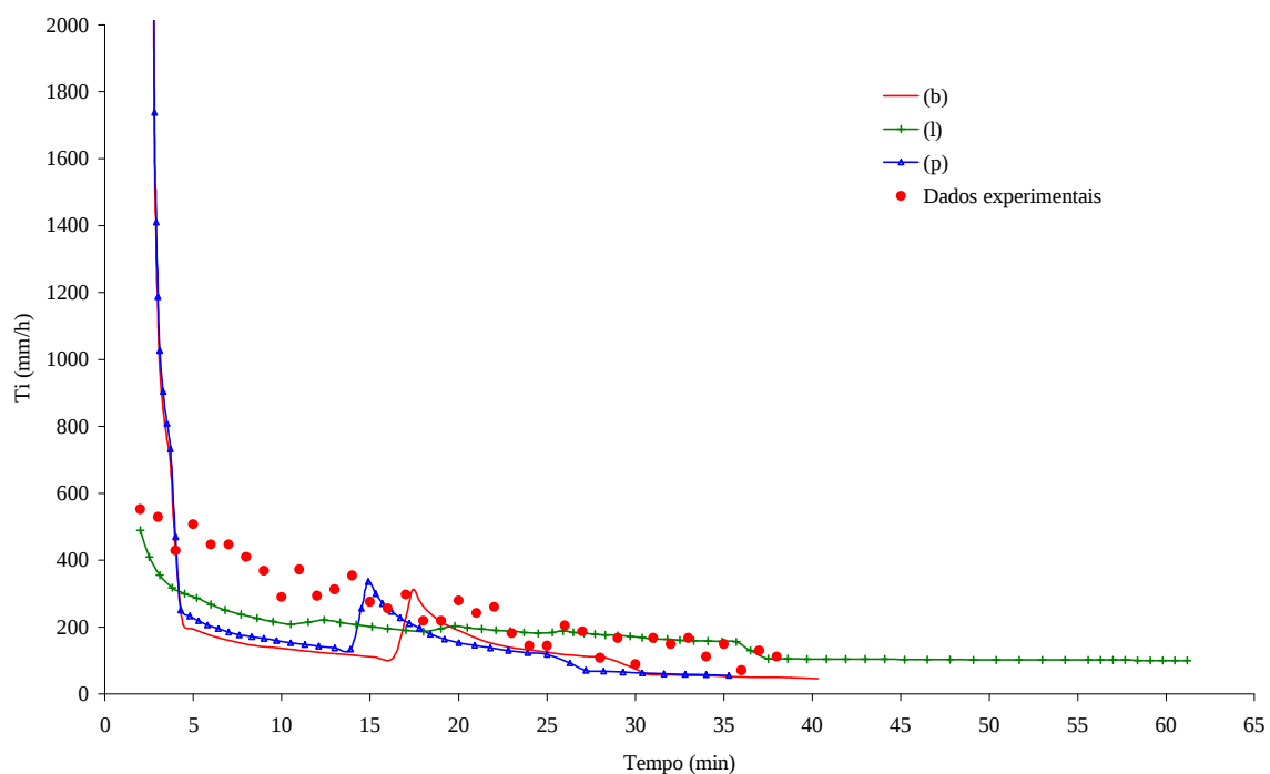
Figura 21 – Taxa de infiltração medida e simulada para a coluna 3, sendo \theta_w igual a 0,86 \theta_s para os três horizontes.
