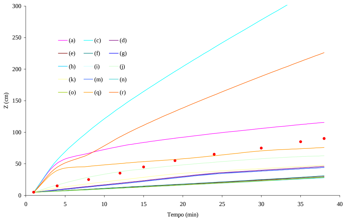
Figura 14D – Profundidade da frente de umedecimento ( z ) medida e simulada para a coluna 4, sendo \theta_w igual a 0,86 \theta_s para os três horizontes.
