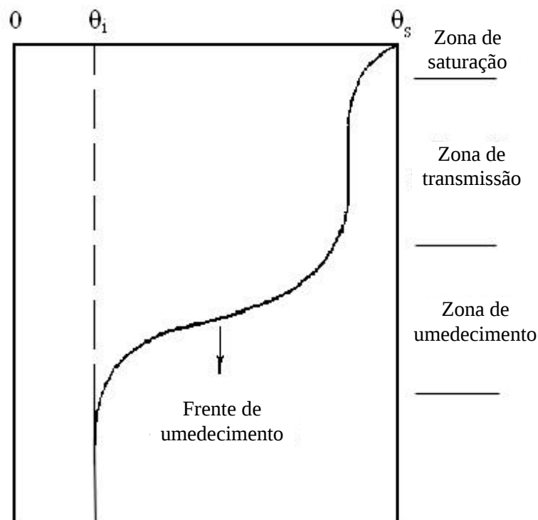
Figura 1 – Esquema representativo da variação do conteúdo de umidade no perfil do solo durante a infiltração.
