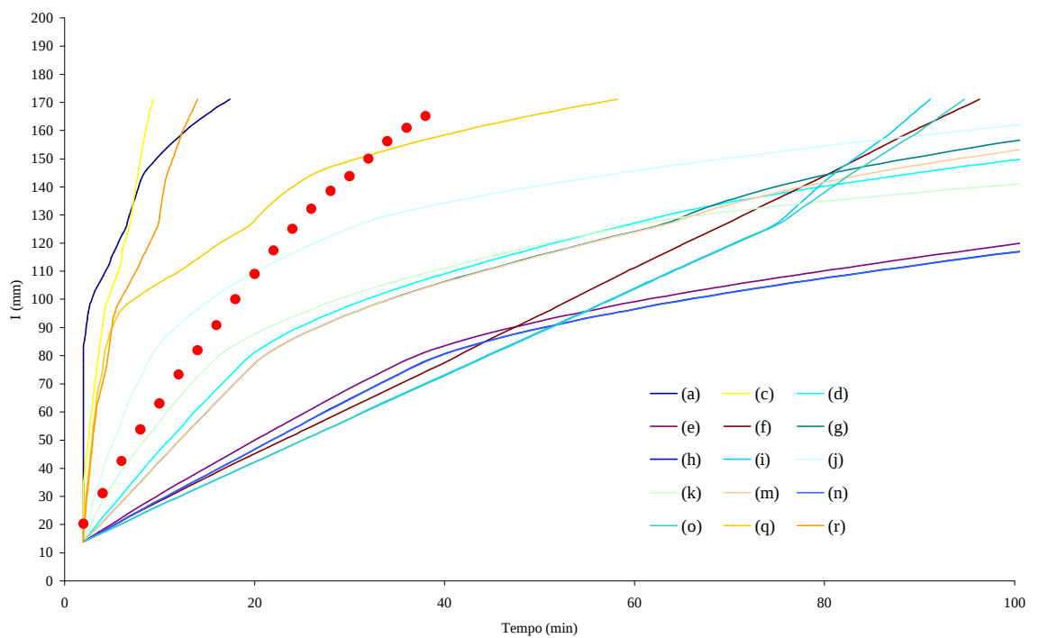
Figura 10D – Infiltração acumulada medida e simulada para a coluna 5, sendo \theta_w igual a 0,84 \theta_s para os três horizontes.
