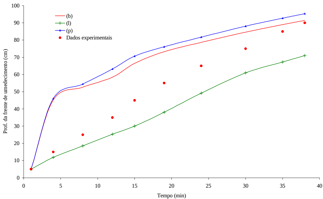
Figura 32 – Profundidade da frente de umedecimento medida e simulada para a coluna 4, sendo \theta_w igual a 0,86 \theta_s para os três horizontes.
