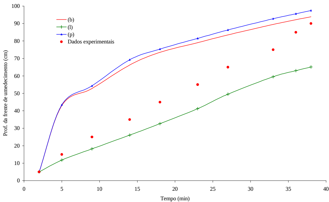
Figura 33 – Profundidade da frente de umedecimento medida e simulada para a coluna 5, sendo \theta_w igual a 0,84 \theta_s para os três horizontes.
