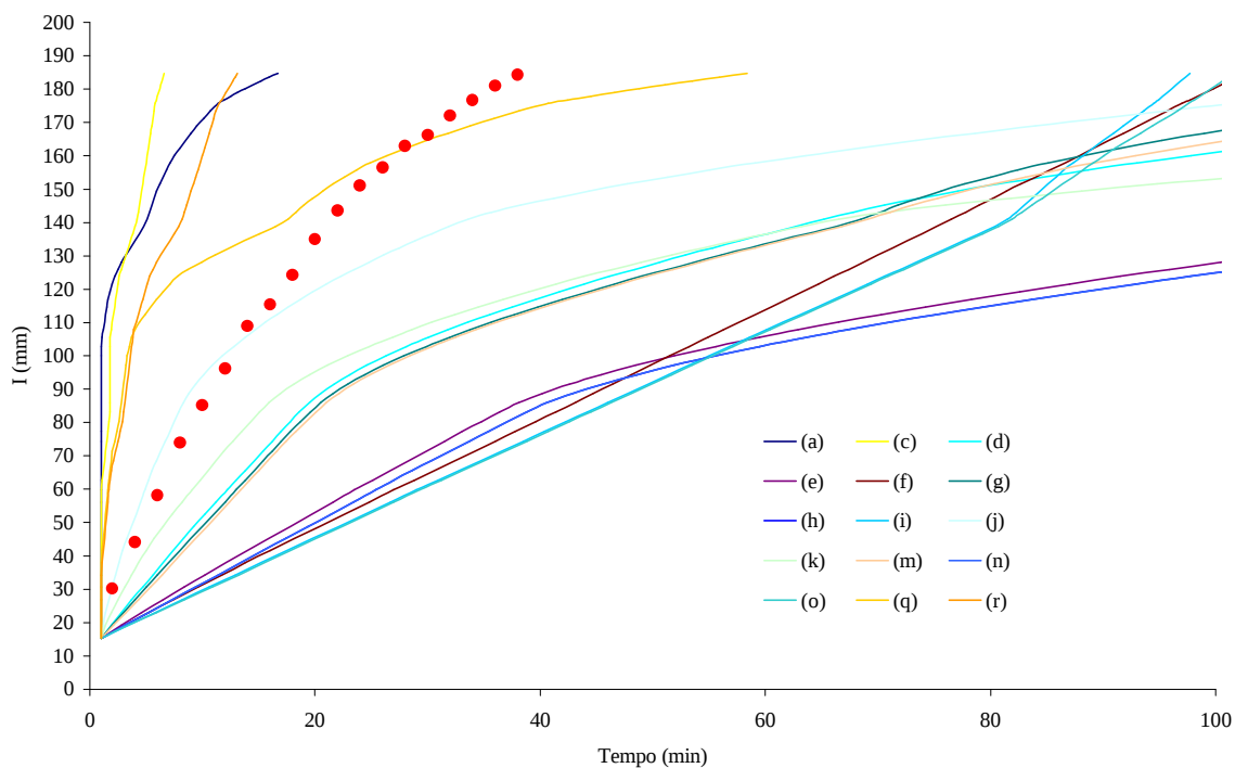
Figura 7D – Infiltração acumulada medida e simulada para a coluna 2, sendo \theta_w igual a 0,86 \theta_s para os três horizontes.
