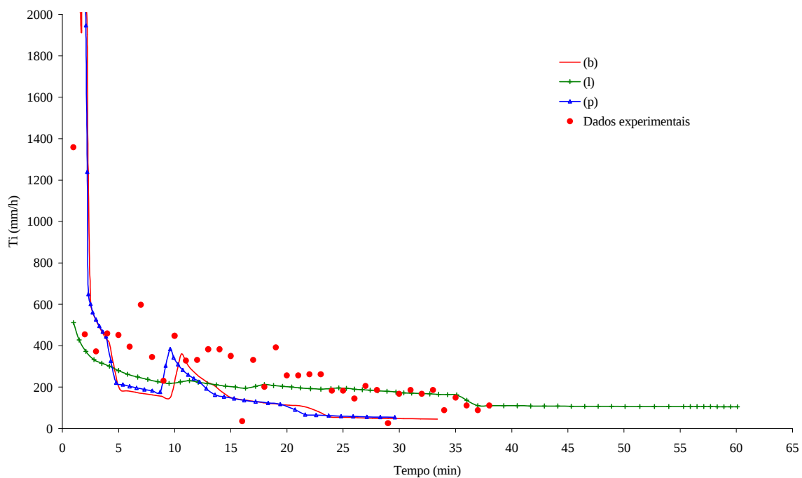
Figura 20 – Taxa de infiltração medida e simulada para a coluna 2, sendo \theta_w igual a 0,86 \theta_s para os três horizontes.
