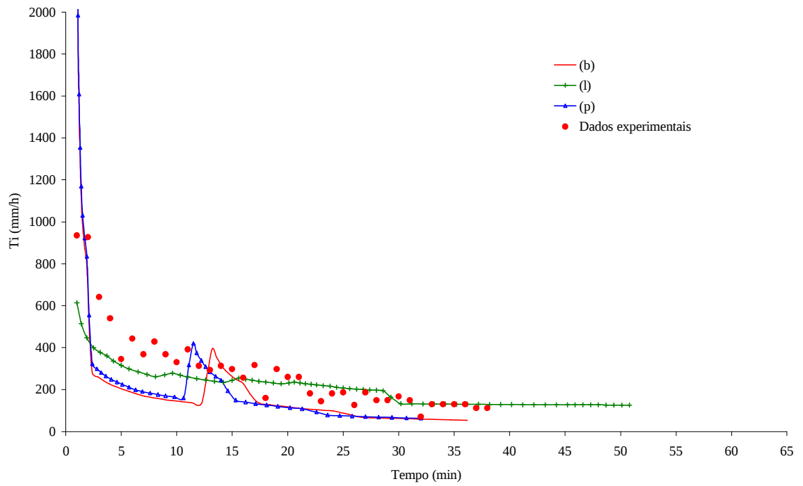
Figura 22 – Taxa de infiltração medida e simulada para a coluna 4, sendo \theta_w igual a 0,86 \theta_s para os três horizontes.
