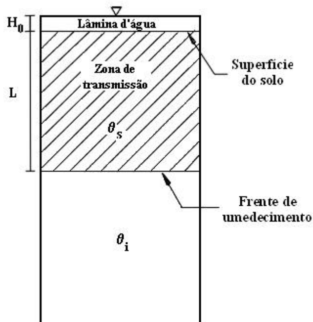
Figura 4 – Esquema representativo da infiltração conforme pressuposições feitas por Green-Ampt, destacando-se as umidades de saturação ( \theta_s ) e inicial ( \theta_i ).
