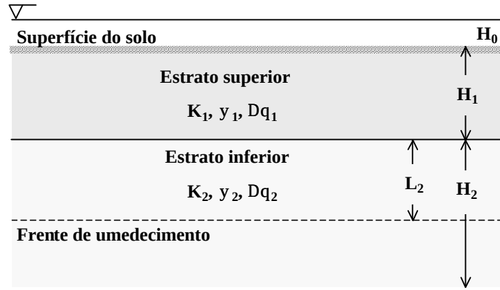
Figura 7 – Parâmetros do modelo de Green-Ampt para solos com dois estratos.
