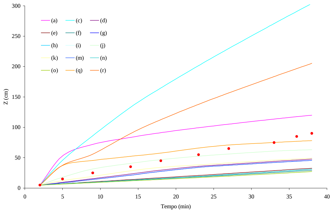
Figura 15D – Profundidade da frente de umedecimento ( z ) medida e simulada para a coluna 5, sendo \theta_w igual a 0,84 \theta_s para os três horizontes.
