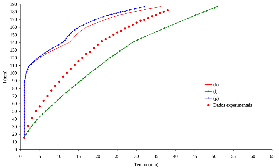
Figura 27 – Infiltração acumulada medida e simulada para a coluna 4, sendo \theta_w igual a 0,86 \theta_s para os três horizontes.
