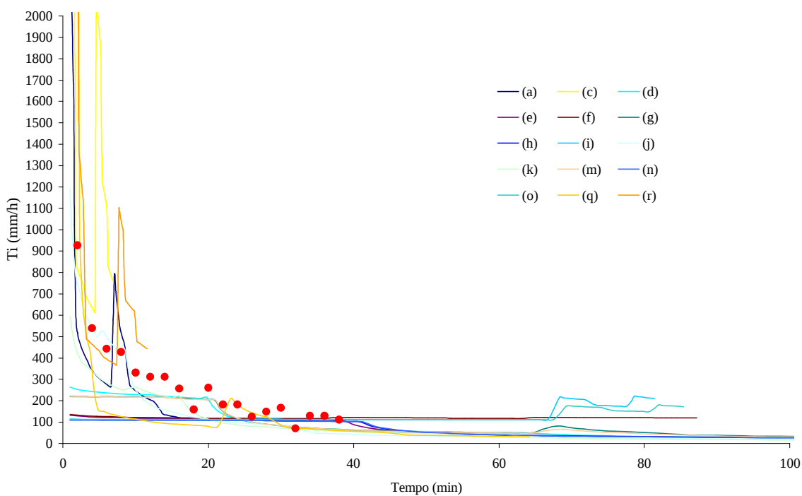
Figura 4D – Taxa de infiltração medida e simulada para a coluna 4, sendo \theta_w igual a 0,86 \theta_s para os três horizontes.
