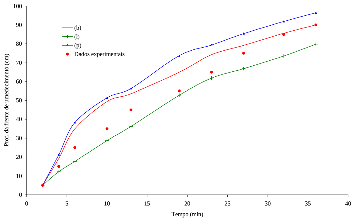
Figura 29 – Profundidade da frente de umedecimento medida e simulada para a coluna 1, sendo \theta_w igual a 0,81 \theta_s para os três horizontes.
