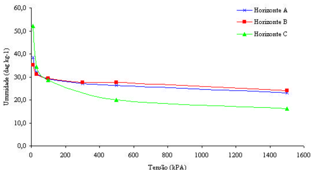
Figura 10 – Curva de retenção de água no solo para os três horizontes.
