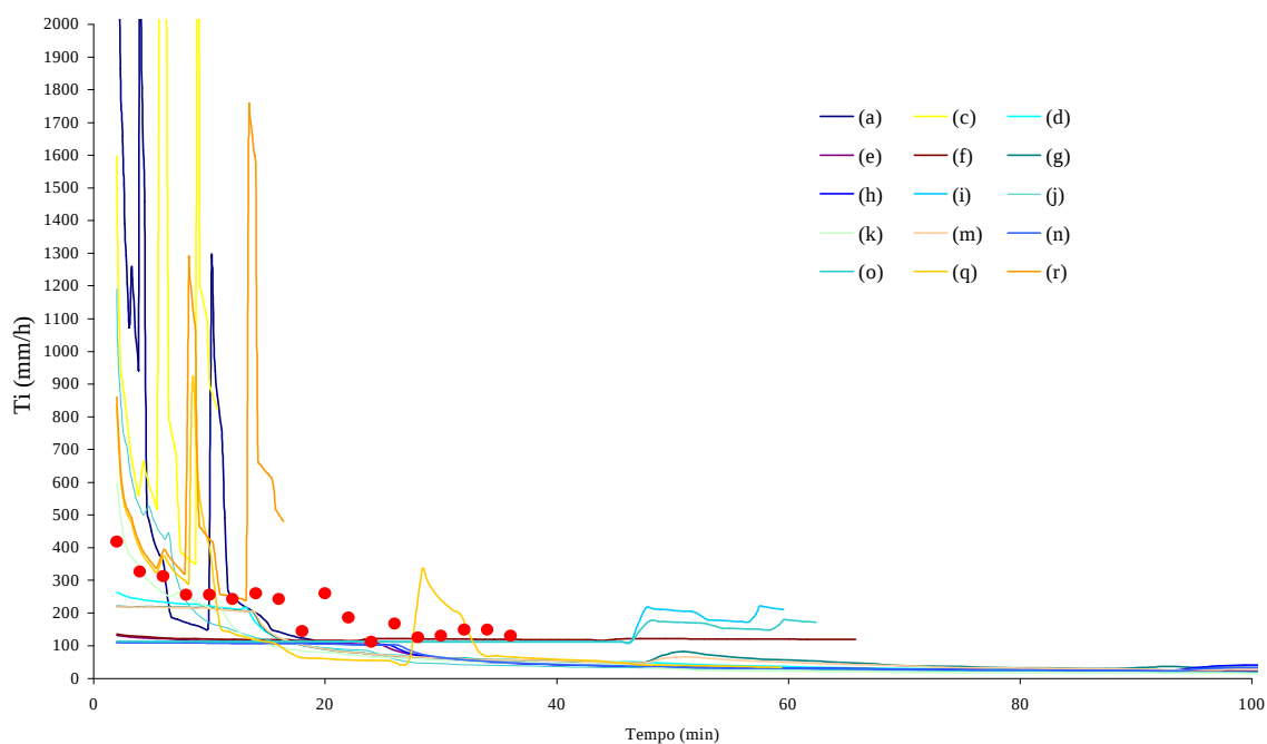
Figura 1D – Taxa de infiltração medida e simulada para a coluna 1, sendo \theta_w igual a 0,81 \theta_s para os três horizontes.
