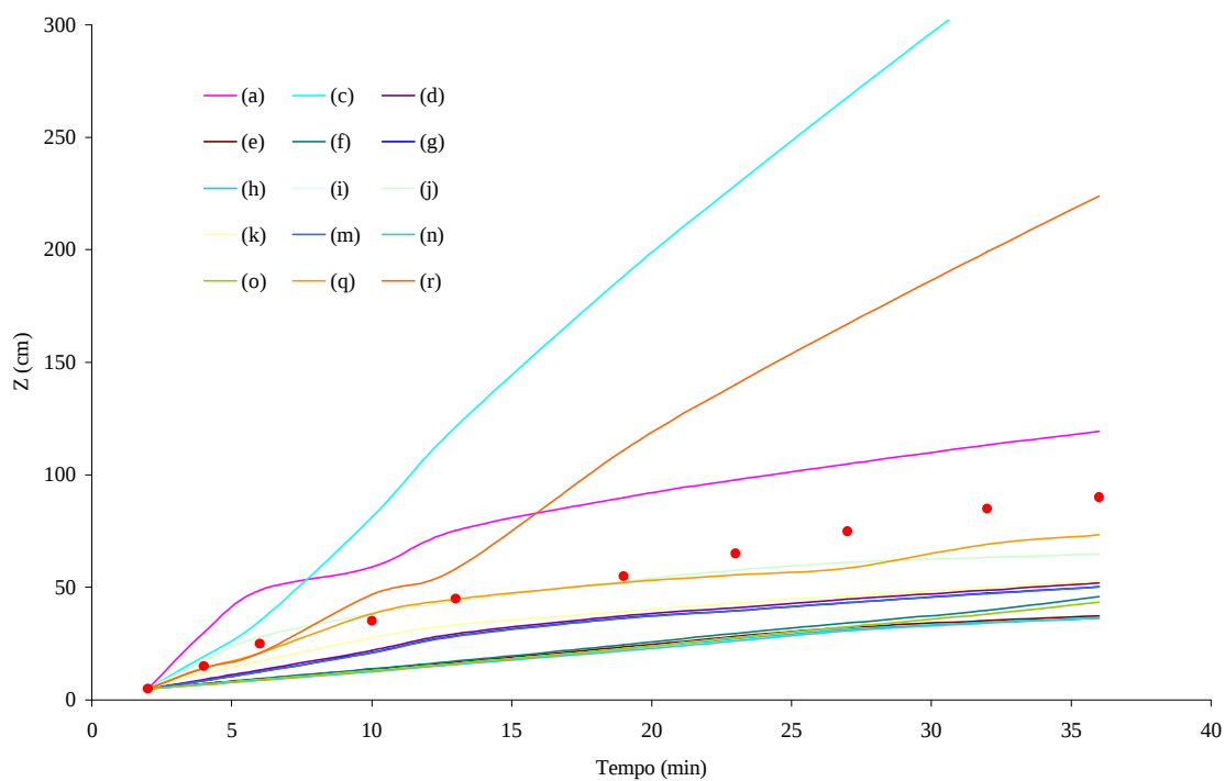
Figura 11D – Profundidade da frente de umedecimento ( z ) medida e simulada para a coluna 1, sendo \theta_w igual a 0,81 \theta_s para os três horizontes.
