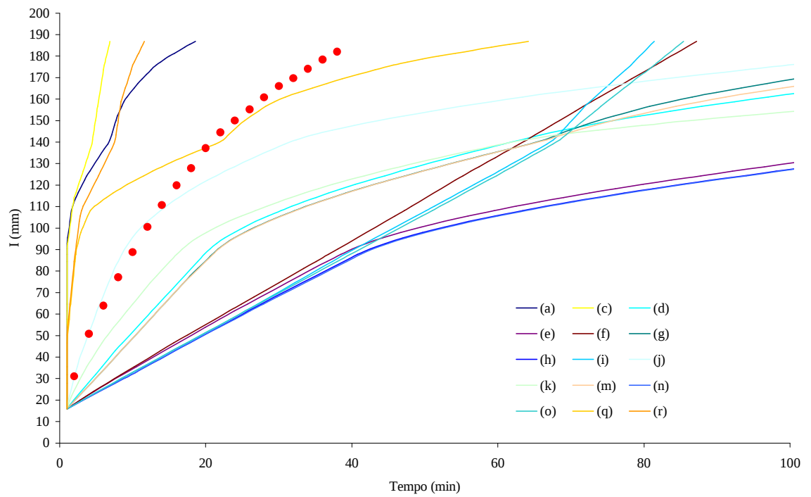
Figura 9D – Infiltração acumulada medida e simulada para a coluna 4, sendo \theta_w igual a 0,86 \theta_s para os três horizontes.
