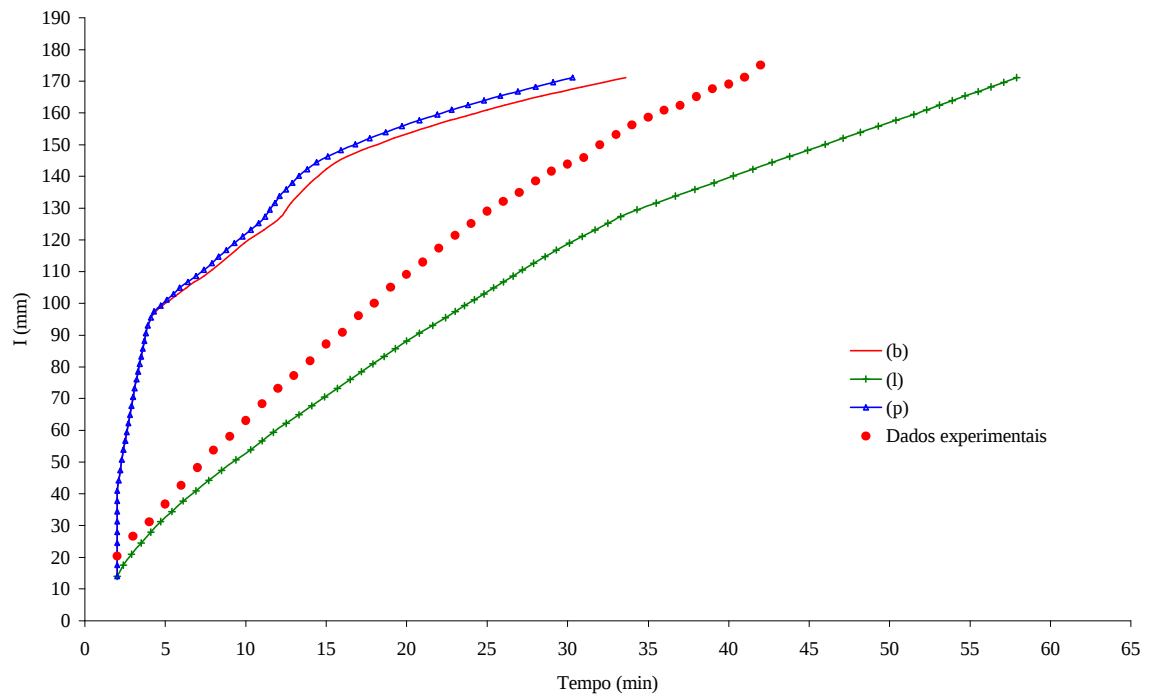
Figura 28 – Infiltração acumulada medida e simulada para a coluna 5, sendo \theta_w igual a 0,84 \theta_s para os três horizontes.
