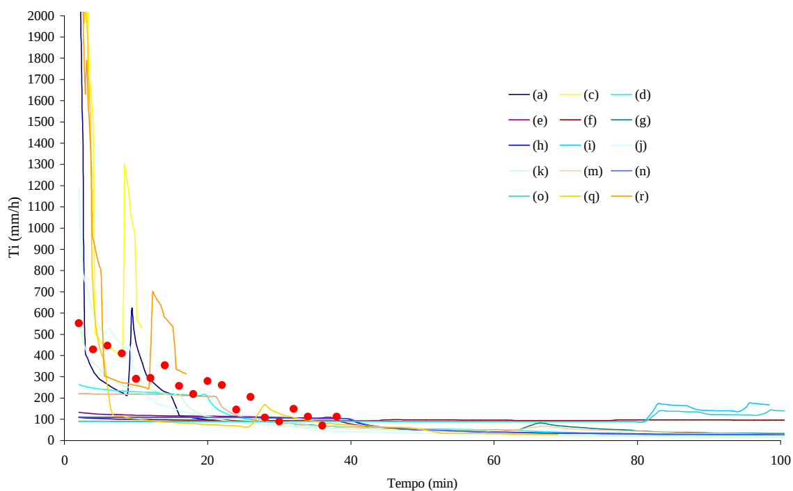
Figura 3D – Taxa de infiltração medida e simulada para a coluna 3, sendo \theta_w igual a 0,86 \theta_s para os três horizontes.
