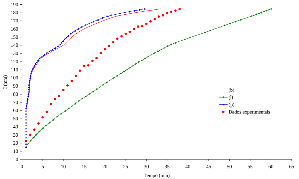
Figura 25 – Infiltração acumulada medida e simulada para a coluna 2, sendo \theta_w igual a 0,86 \theta_s para os três horizontes.
