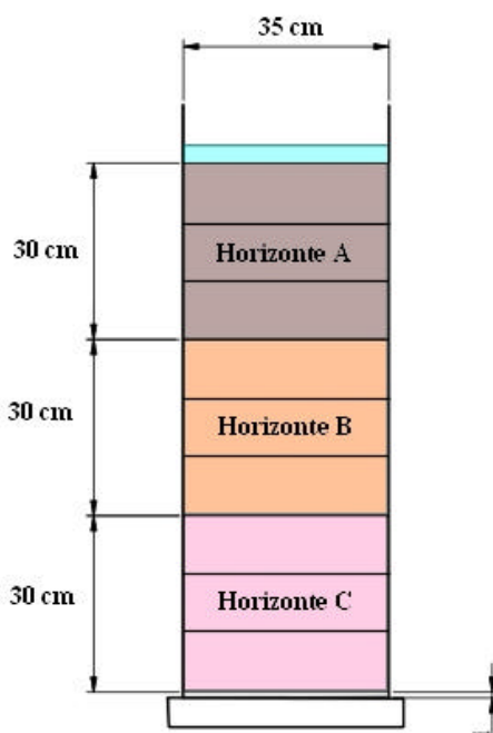
Figura 11 – Esquema representativo da disposição final das camadas de solo dentro das colunas.
