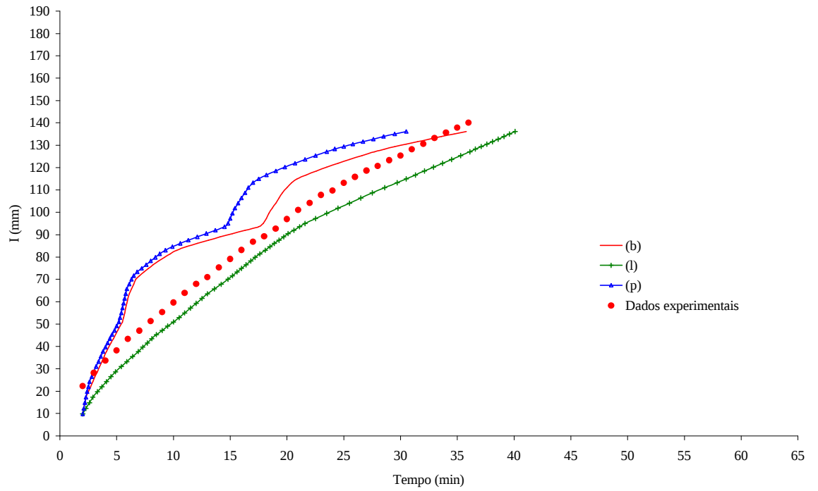
Figura 24 – Infiltração acumulada medida e simulada para a coluna 1, sendo \theta_w igual a 0,81 \theta_s para os três horizontes.
