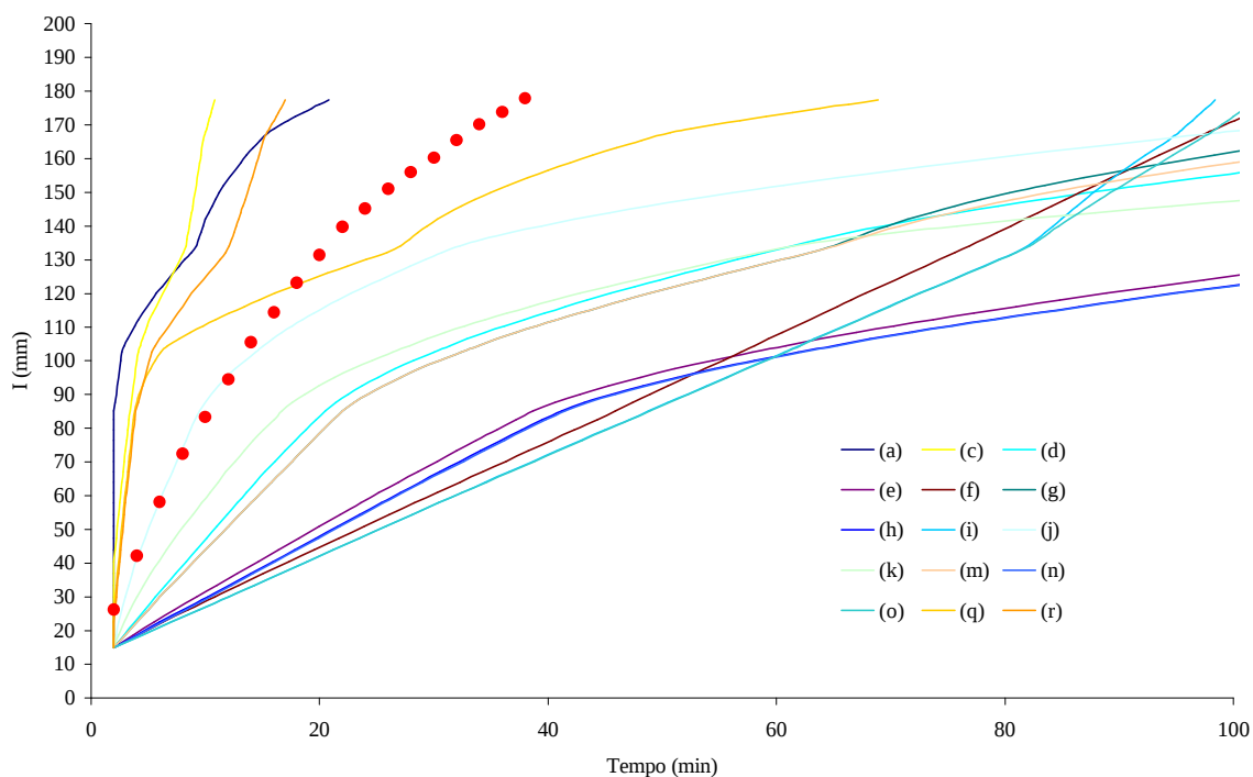
Figura 8D – Infiltração acumulada medida e simulada para a coluna 3, sendo \theta_w igual a 0,86 \theta_s para os três horizontes.
