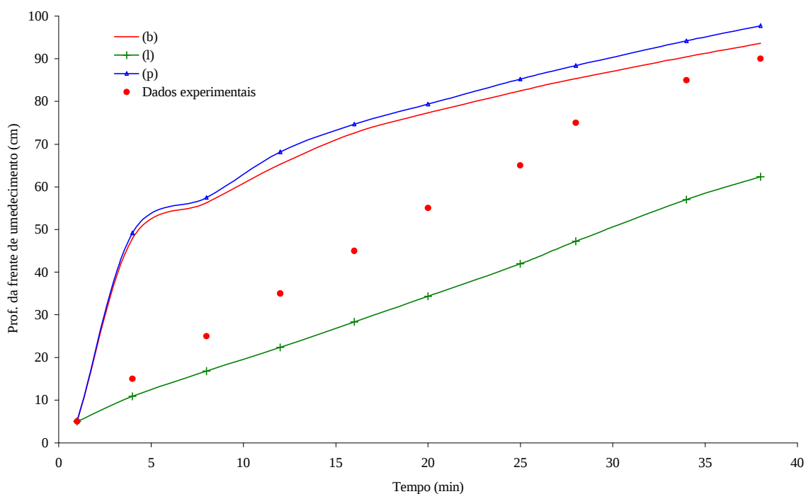
Figura 30 – Profundidade da frente de umedecimento medida e simulada para a coluna 2, sendo \theta_w igual a 0,86 \theta_s para os três horizontes.
