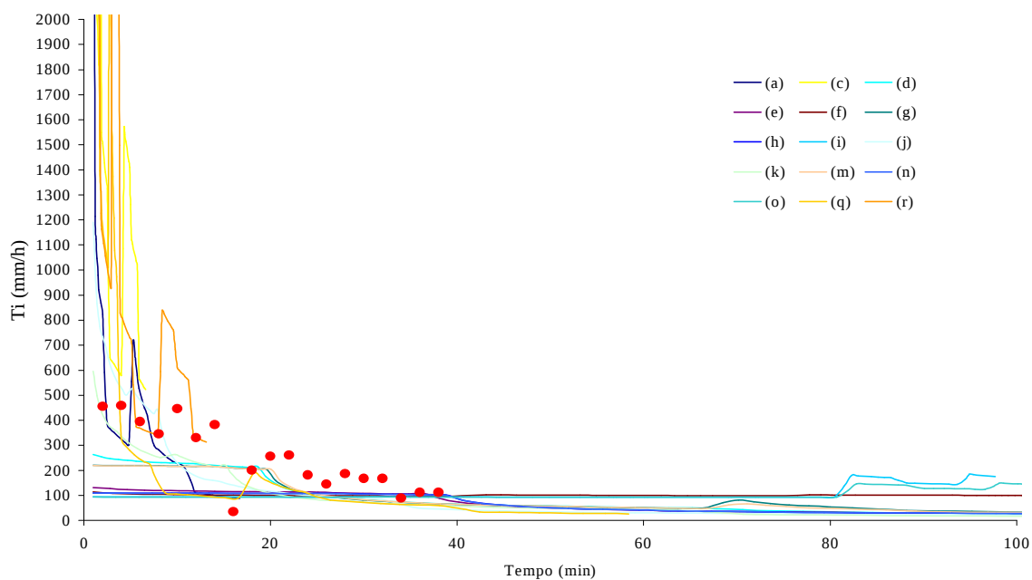
Figura 2D – Taxa de infiltração medida e simulada para a coluna 2, sendo \theta_w igual a 0,86 \theta_s para os três horizontes.
