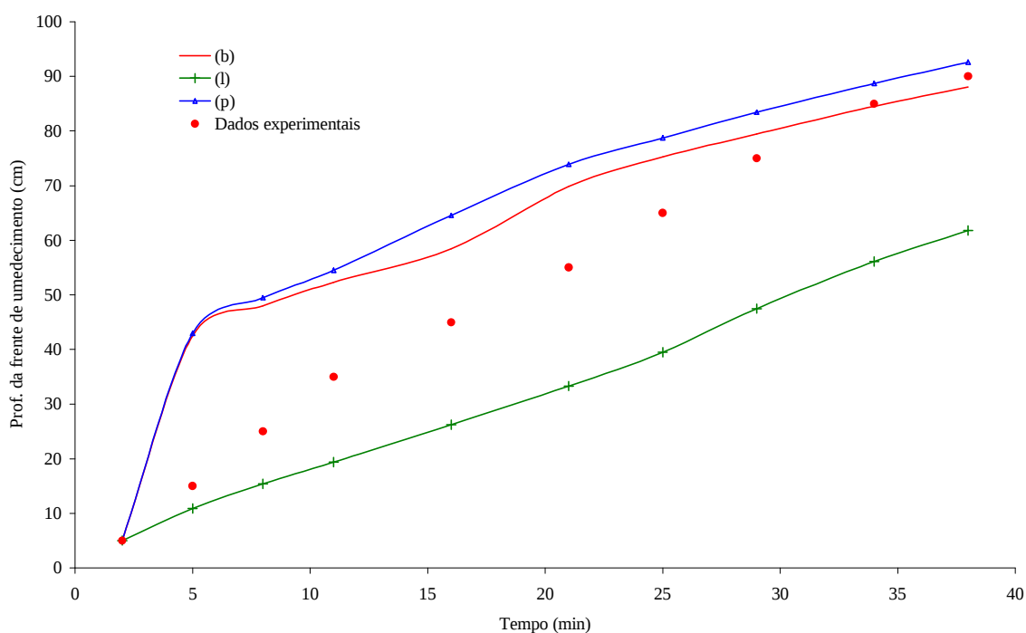
Figura 31 – Profundidade da frente de umedecimento medida e simulada para a coluna 3, sendo \theta_w igual a 0,86 \theta_s para os três horizontes.
