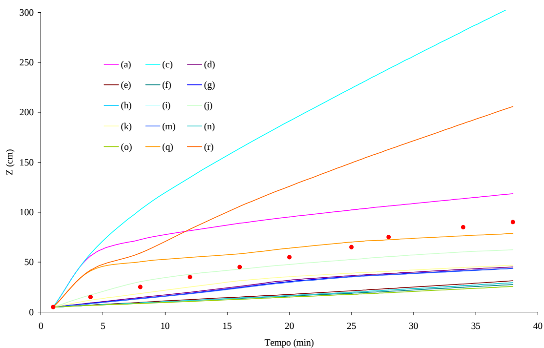
Figura 12D – Profundidade da frente de umedecimento ( z ) medida e simulada para a coluna 2, sendo \theta_w igual a 0,86 \theta_s para os três horizontes.
