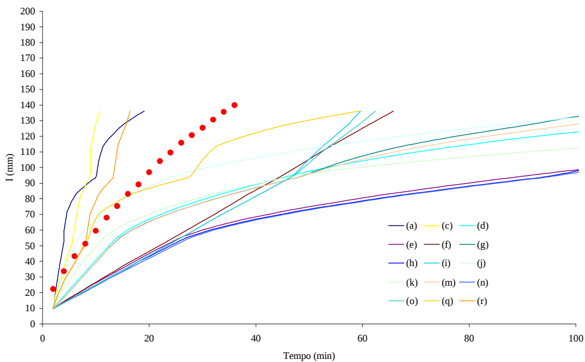
Figura 6D – Infiltração acumulada medida e simulada para a coluna 1, sendo \theta_w igual a 0,81 \theta_s para os três horizontes.
