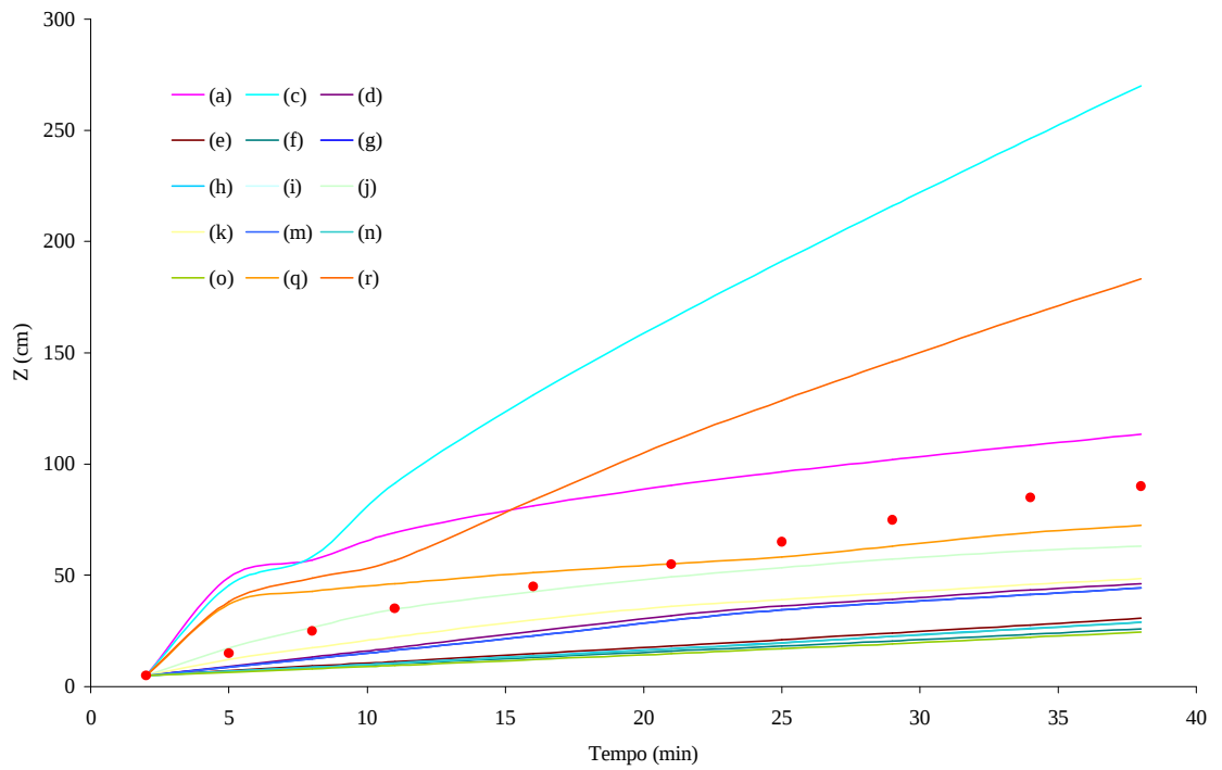
Figura 13D – Profundidade da frente de umedecimento ( z ) medida e simulada para a coluna 3, sendo \theta_w igual a 0,86 \theta_s para os três horizontes.
