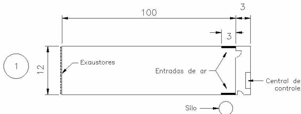
FIGURA 2. Croqui - detalhe das entradas de ar e da posição dos exaustores na instalação semi-climatizada com ventilação por pressão negativa.
