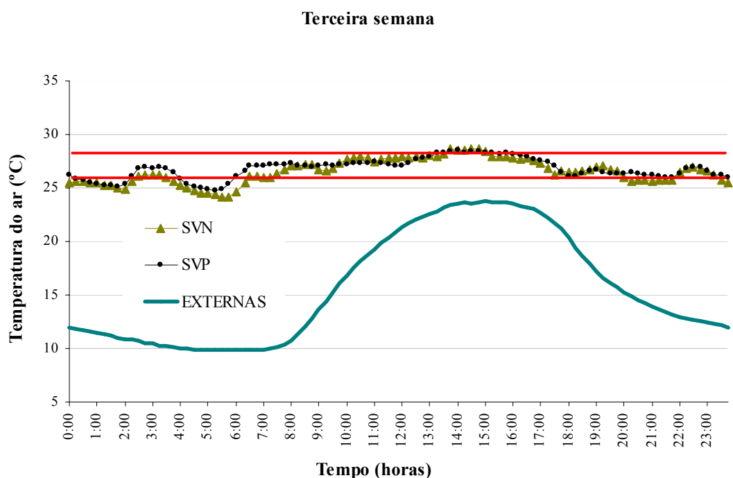
FIGURA 7. Médias de temperatura do ar no ambiente interno e externo, em função dos horários na terceira semana, correspondentes aos tratamentos SVN e SVP.
