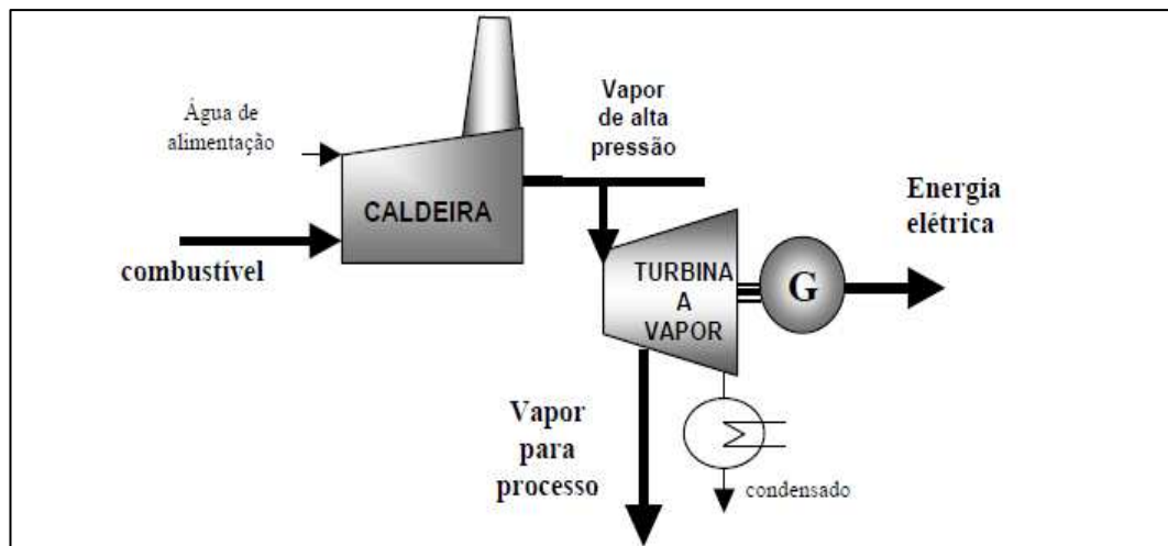
Figura 5: Representação da cogeração com ciclo Rankine. Fonte: Brasil (2005).
