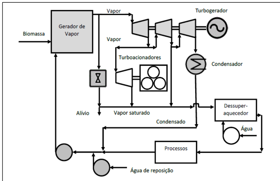
Figura 6: Ciclo vapor com condensação e extração em cogeração e na geração elétrica. Fonte: Tolmasquim (2016).
