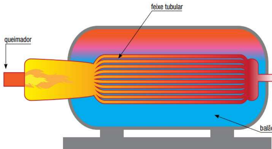
Figura 7: Representação esquemática de caldeira flamotubular.
