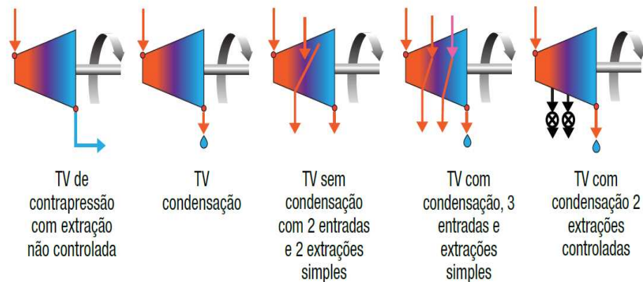
Figura 9: Representação esquemática de tipos de turbinas a vapor.
