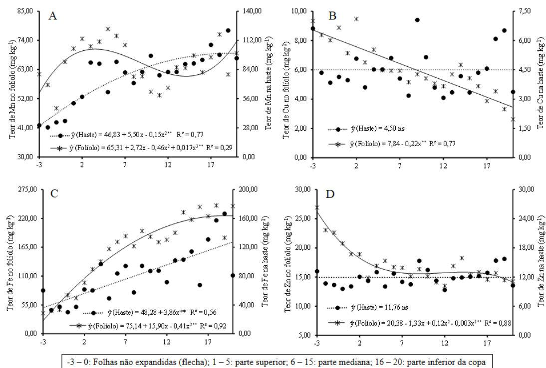
Figura 3 – Teores de micronutrientes nos folíolos e haste foliar em diferentes posições do ápice para a base da copa de plantas de macaúba adultas e produtivas. ns, *, ** = não significativo, significativo a 5 e 1 % pelo teste t.
