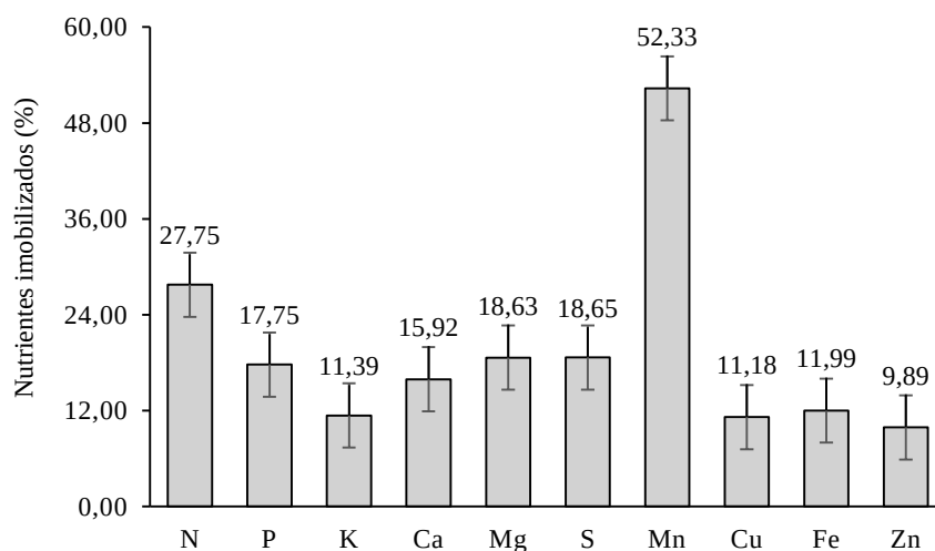
Figura 3 – Partição de macro e micronutrientes em partes senescidas de plantas de macaúba adultas e produtivas. Dados: as barras no gráfico representam o erro padrão da média.
