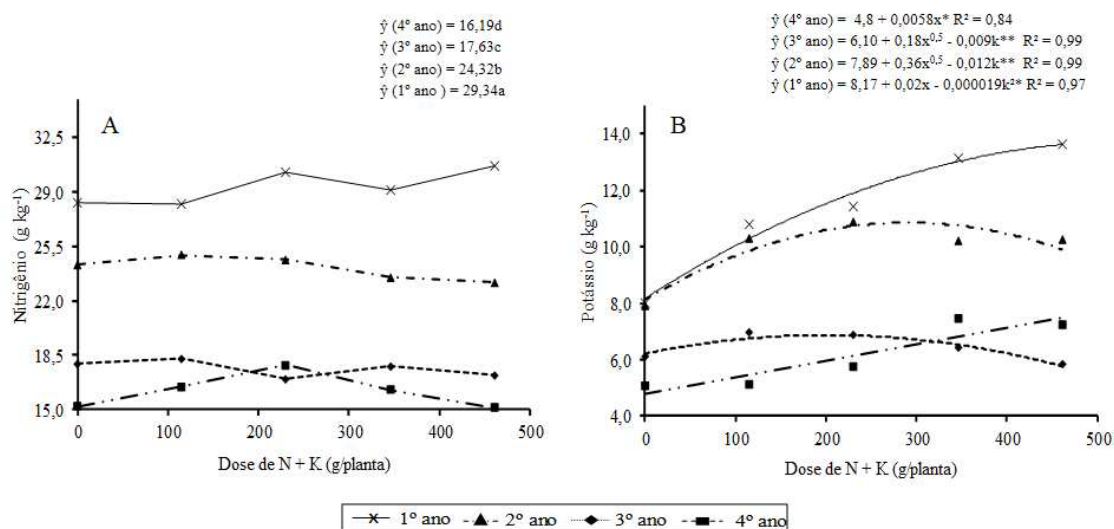
Figura 3 – Teores foliares de N (A) e K (B) em função das doses de NK e do ano de avaliação. Dados: * e ** Significativo a 5 e 1 % de probabilidade, respectivamente.
