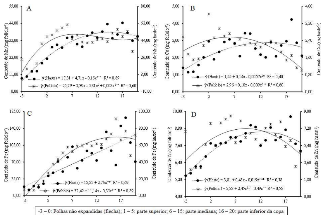
Figura 5 – Conteúdos de micronutrientes nos folículos e haste foliar em diferentes posições do ápice para a base da copa das plantas de macaúba adultas e produtivas. *, ** = significativo a 5 e 1 % pelo teste t.
