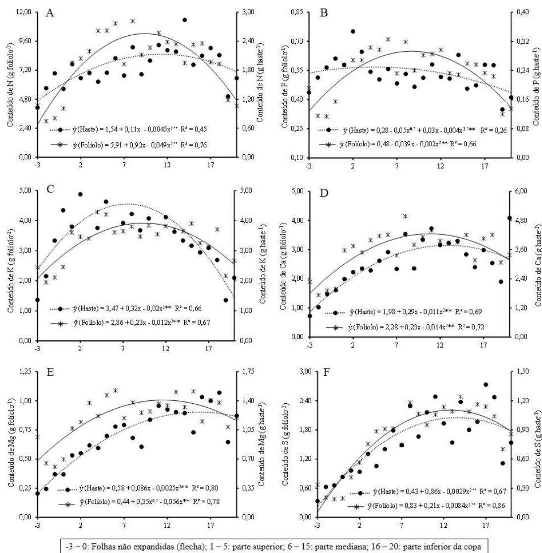
Figura 4 – Conteúdos de macronutrientes nos folíolos e haste foliar em diferentes posições do ápice para a base da copa das plantas de macaúba adultas e produtivas. *, ** = significativo a 5 e 1 % pelo teste t.
