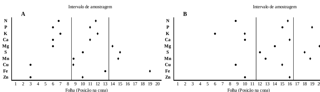
Figura 6 – Intervalo de folhas para amostragem dentro da faixa de maior estabilidade dos conteúdos de macro e micronutrientes nos folíolos (A) e na haste foliar (B) da macaúba.
