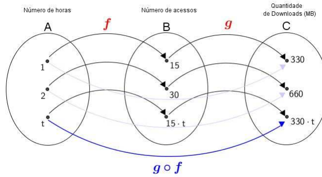
Figura 1.16: Função Composta
