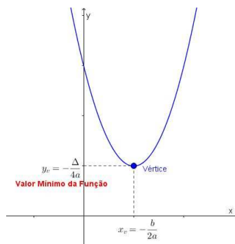
Figura 3.3: Valor Mínimo
