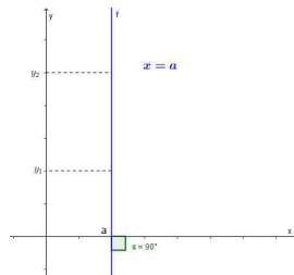
Figura 2.4: \alpha = 90^\circ
