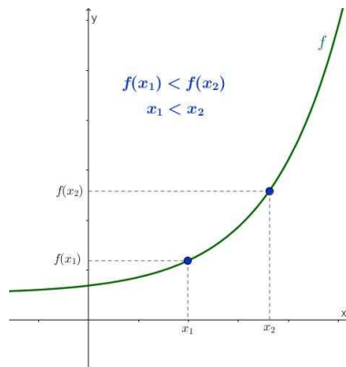
Figura 4.3: a > 1
