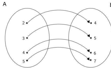
Figura 1.15: Exemplo de Bijecção
