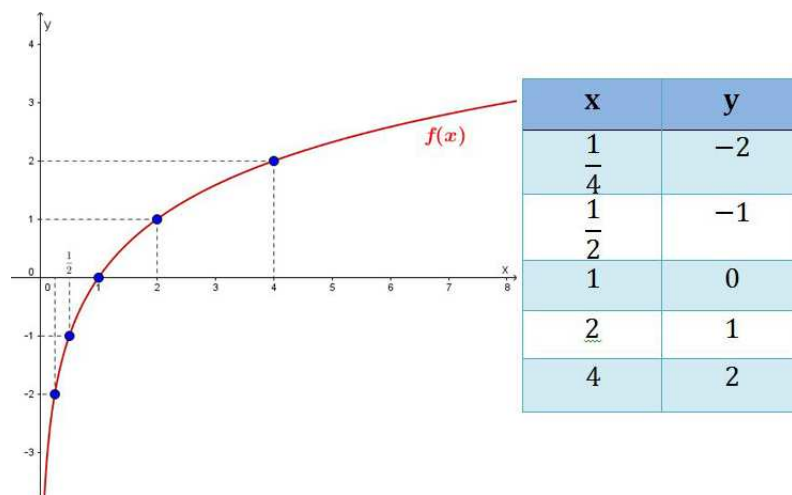
Figura 4.5: Função Crescente f
