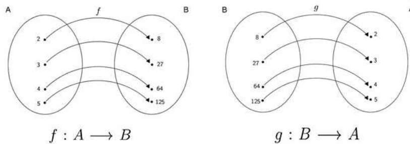
Figura 1.17: Função Inversa
