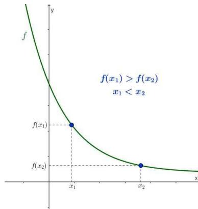
Figura 4.4: a < 1
