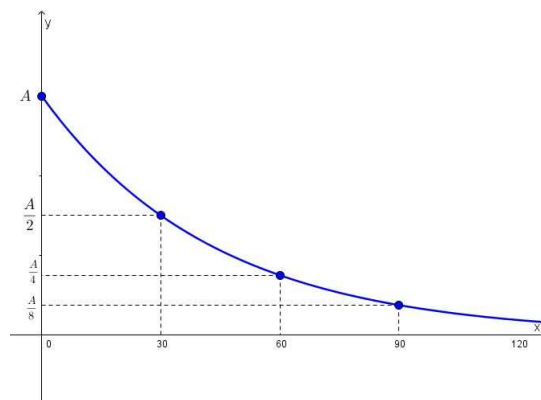
Figura 4.11: Meia vida do Césio-137
