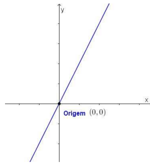
Figura 2.5: Função Linear \longrightarrow f(x) = ax
