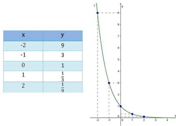
Figura 4.2: Função Decrescente
