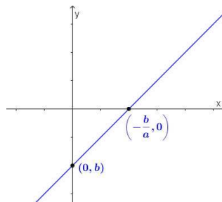
Figura 2.6: Pontos de interseção da Função Afim
