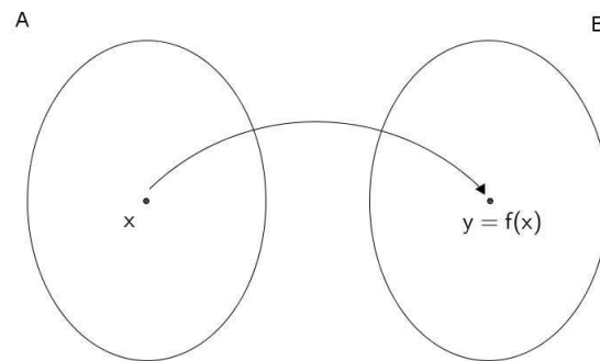
Figura 1.1: Representação por Diagramas
