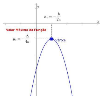
Figura 3.4: Valor Máximo
