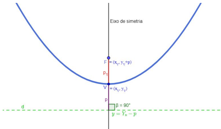
Figura 4.2: Parábola como LG e seus elementos.
