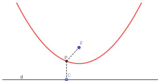
Figura 2.13: Parábola como LG.
