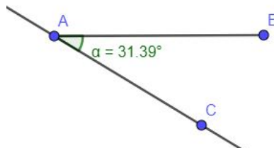
Figura 2.8: Segundo passo para construção do arco capaz. Fonte: Elaborado pela autora.
