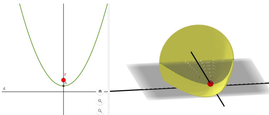
Figura 4.16: Parábola rotacionada com respectivos foco e diretriz.
