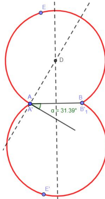
Figura 2.6: Simetria do arco capaz. Fonte: Elaborado pela autora.
