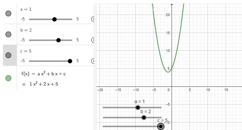
Figura 4.6: Variações dos coeficientes e respectiva representação gráfica.
