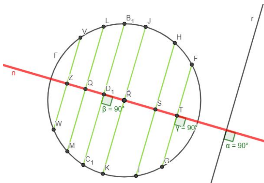
Figura 3.7: LG dos pontos médios das cordas de \Gamma .
