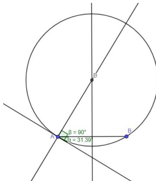
Figura 2.10: Quarto passo para construção do arco capaz. Fonte: Elaborado pela autora.
