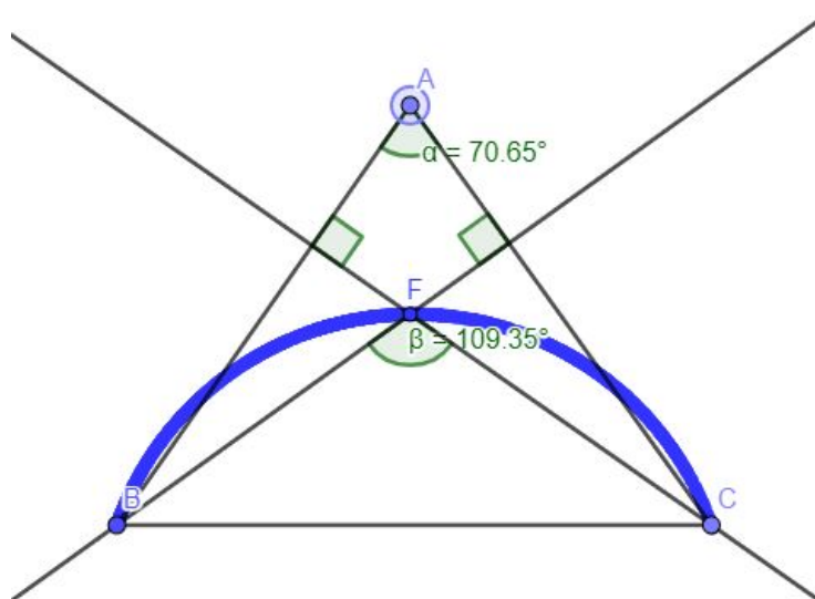
Figura 3.3: Novo arco capaz gerado a partir do triângulo.
