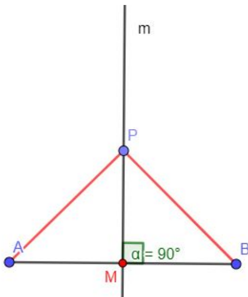
Figura 2.4: Mediatriz como LG
