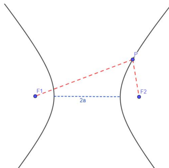
Figura 2.20: Hipérbole como LG. Fonte: Elaborado pela autora.
