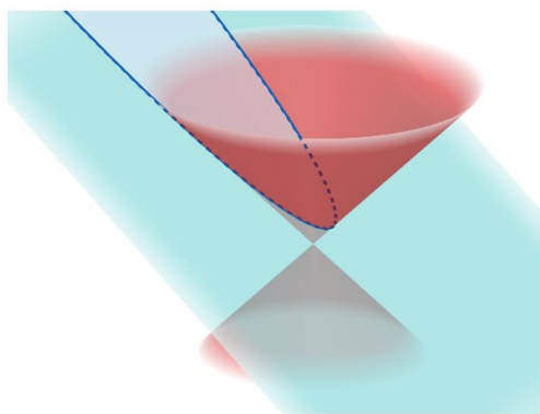
Figura 4.5: Construção da parábola pela intersecção de um plano com um cone duplo de revolução.
