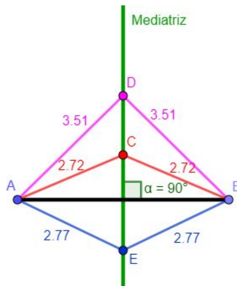
Figura 2.3: Mediatriz: equidistância de seus pontos aos extremos do segmento. Fonte: Elaborado pela autora.
