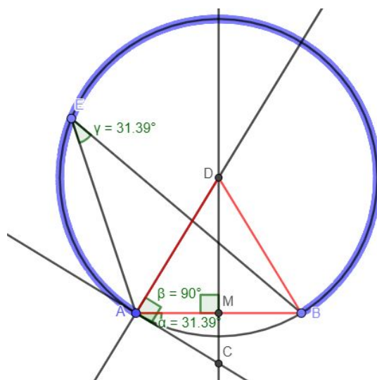
Figura 2.12: Sexto passo para construção do arco capaz. Fonte: Elaborado pela autora.
