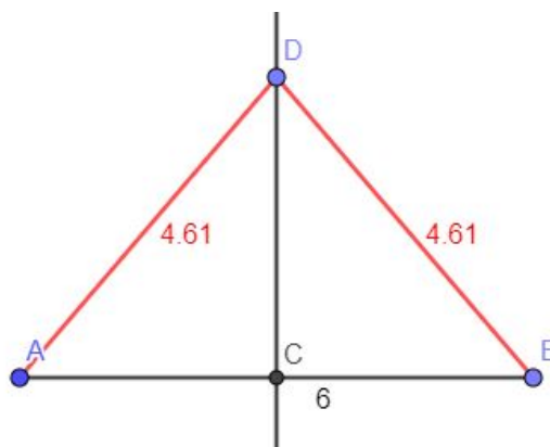
Figura 4.1: Mediatriz de um segmento
