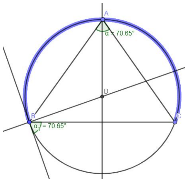
Figura 3.2: Construção do triângulo a partir do arco capaz.
