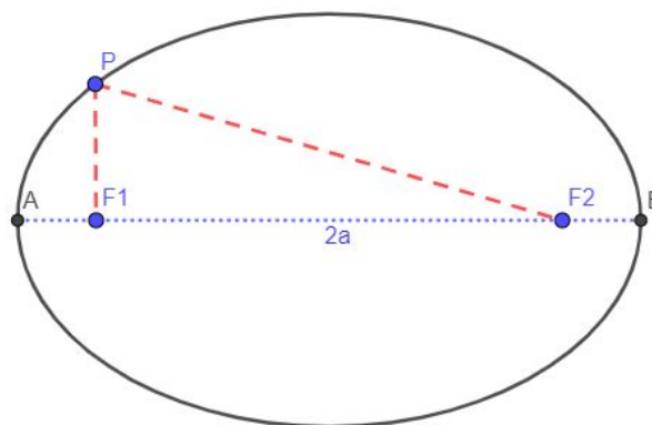
Figura 2.18: Elipse como LG
