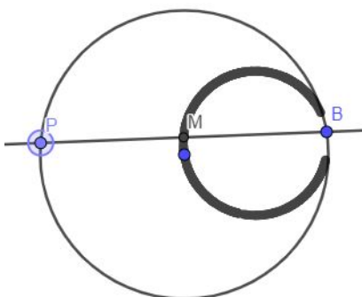
Figura 3.9: Ponto P pertencente à circunferência.
