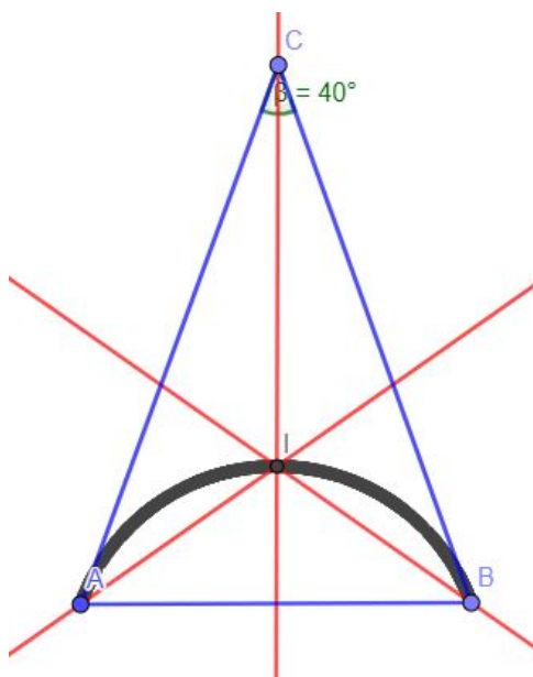
Figura 3.12: Exemplo 6: arco capaz do ângulo de 110^\circ .
