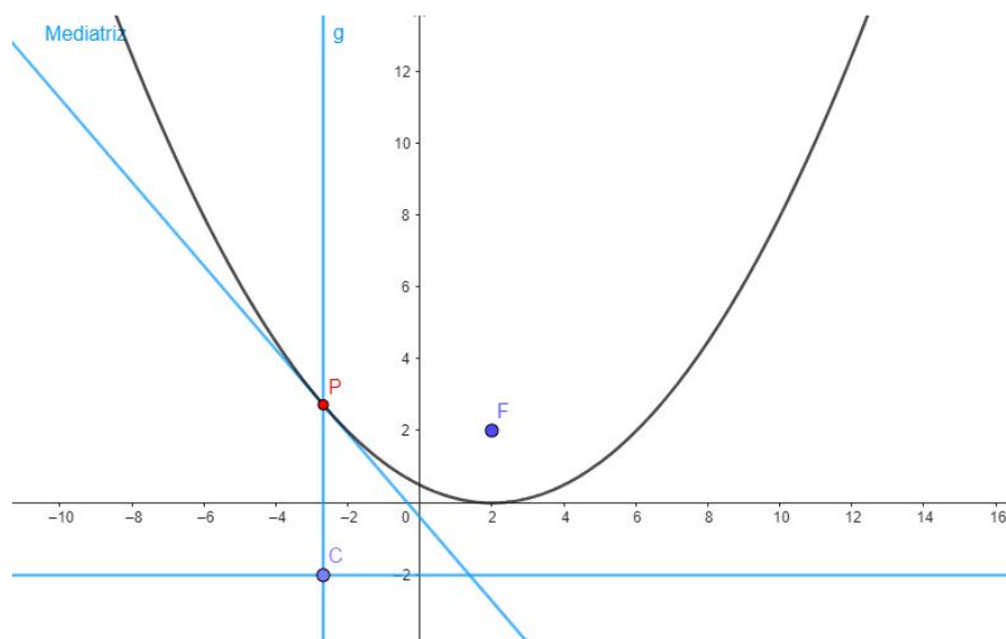
Figura 4.4: Construção da parábola como LG.
