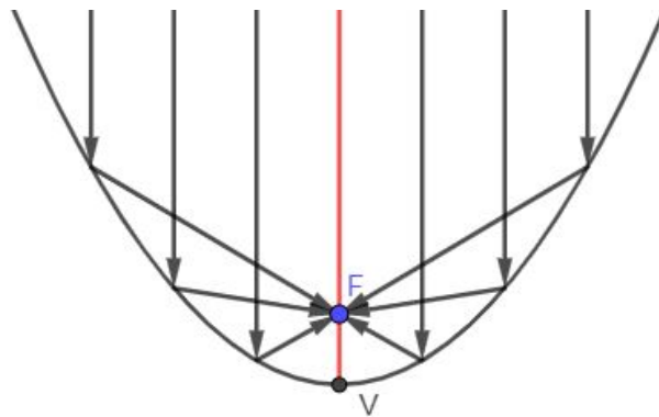
Figura 2.16: Propriedade refletora da parábola - I.
