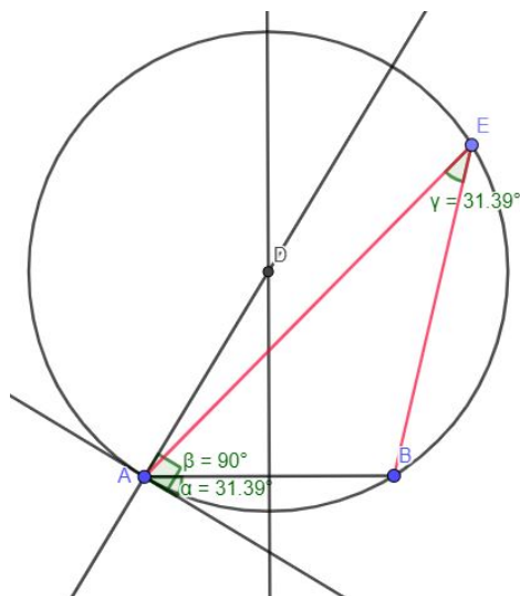
Figura 2.11: Quinto passo para construção do arco capaz. Fonte: Elaborado pela autora.
