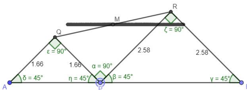
Figura 3.5: LG descrito pelo ponto M - Ponto P na posição inicial.
