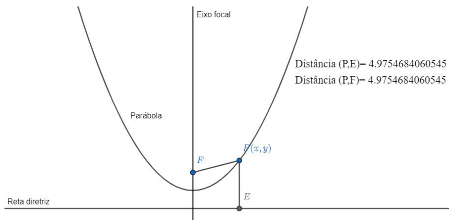
Figura 4.7: Definição de parábola - GeoGebra.
