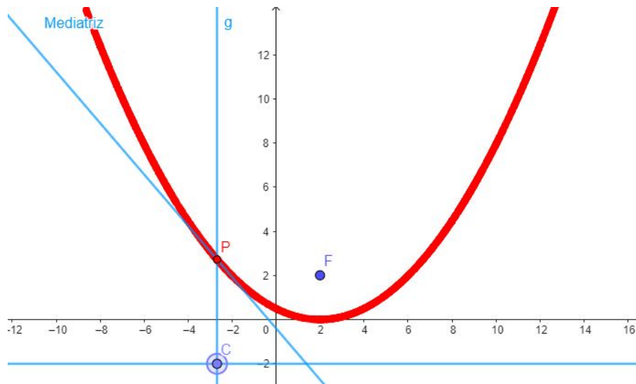
Figura 4.3: Construção da parábola
