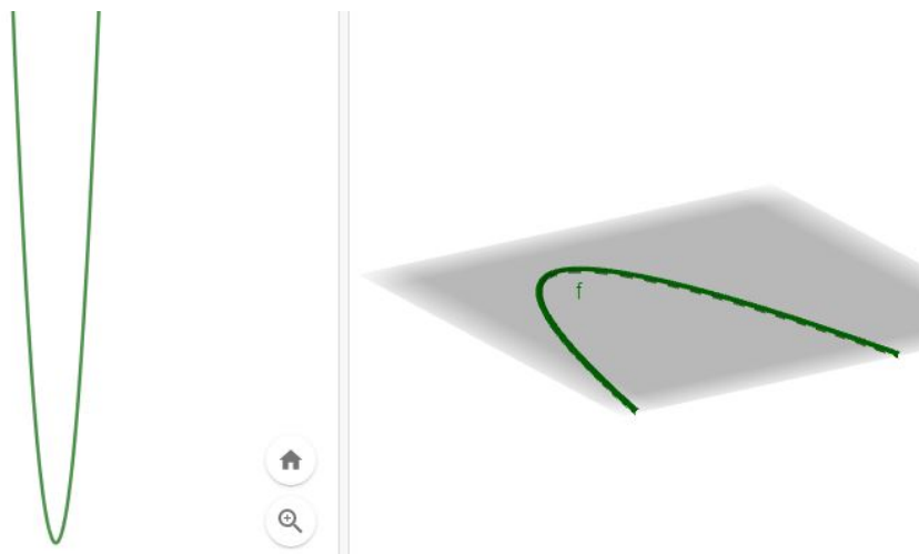
Figura 4.12: Primeiro passo para construção do parabolóide.
