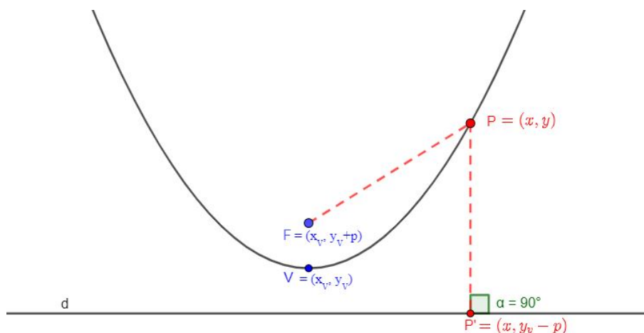
Figura 2.15: Parábola e seus elementos para demonstração da equação geral.
