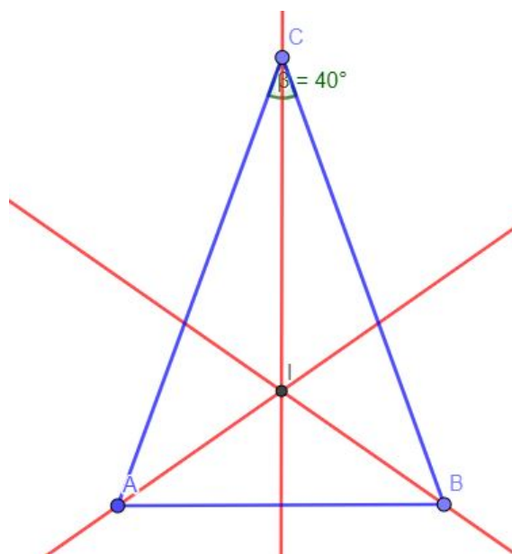
Figura 3.11: Exemplo 6: Incentro do triângulo ABC .
