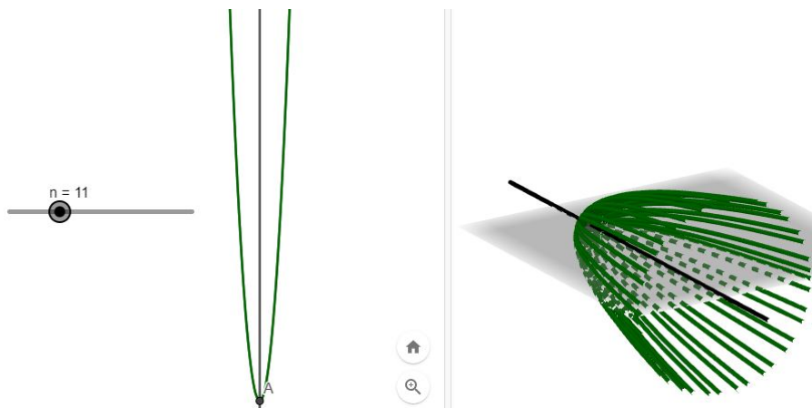
Figura 4.14: Construção do parabolóide após a 11 a rotação.
