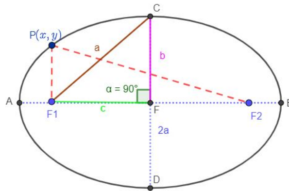
Figura 2.19: Elementos da Elipse Fonte: Elaborado pela autora.
