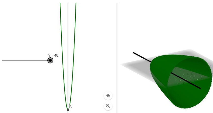
Figura 4.15: Construção do parabolóide após a 40 a rotação
