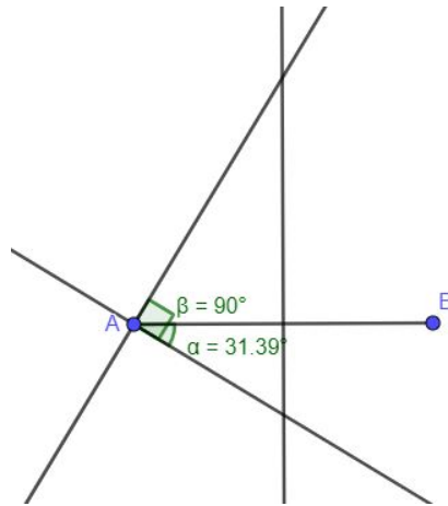
Figura 2.9: Terceiro passo para construção do arco capaz. Fonte: Elaborado pela autora.
