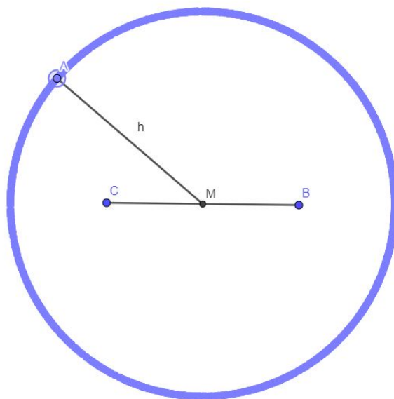
Figura 3.1: LG do vértice A.
