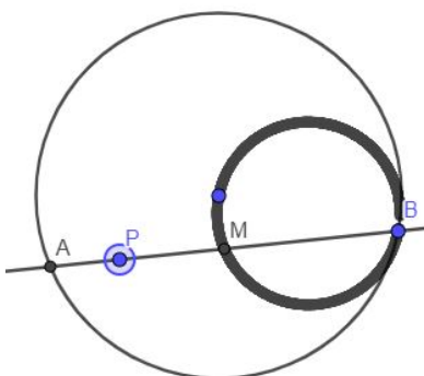
Figura 3.10: Ponto P interior à circunferência.
