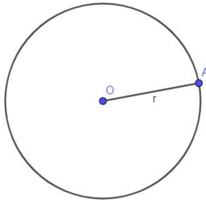
Figura 2.1: Circunferência como LG
