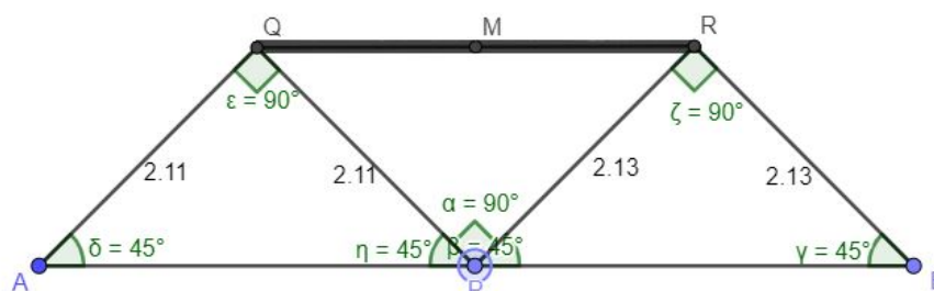
Figura 3.6: LG descrito pelo ponto M - Ponto P na posição final.
