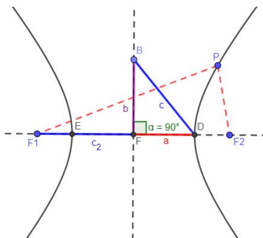
Figura 2.21: Elementos da hipérbole.
