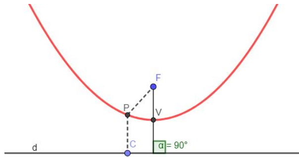
Figura 2.14: Vértice da parábola.
