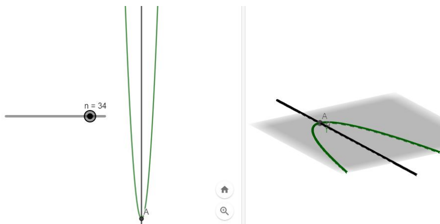
Figura 4.13: Construção do parabolóide - enfoque ao eixo de simetria.
