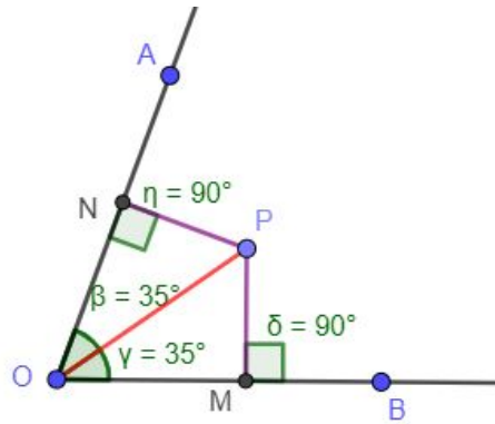
Figura 2.5: Bissetriz como LG Fonte: Elaborado pela autora.
