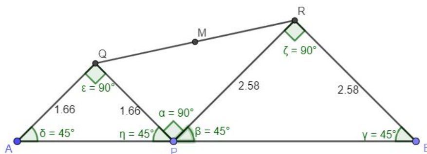
Figura 3.4: Representação geométrica do exemplo 3
