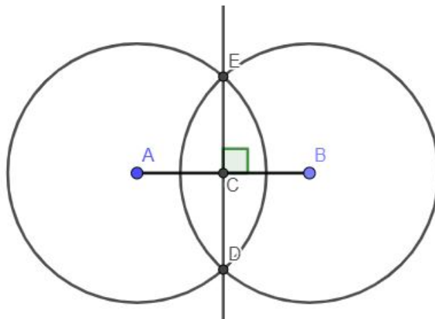
Figura 2.2: Construção da mediatriz de um segmento. Fonte: Elaborado pela autora.
