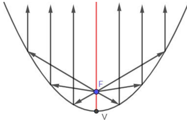
Figura 2.17: Propriedade refletora da parábola - II.
