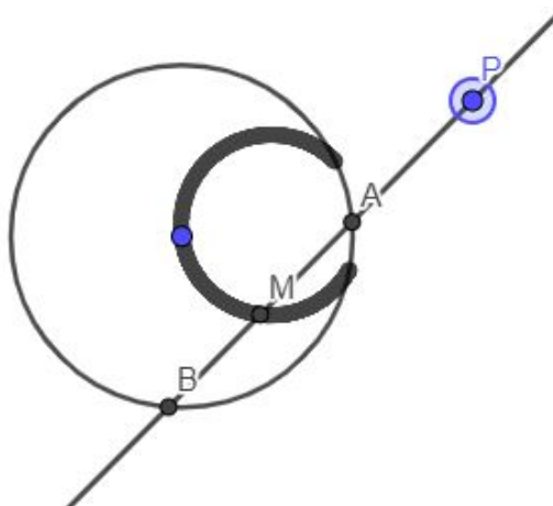
Figura 3.8: Ponto P exterior à circunferência.
