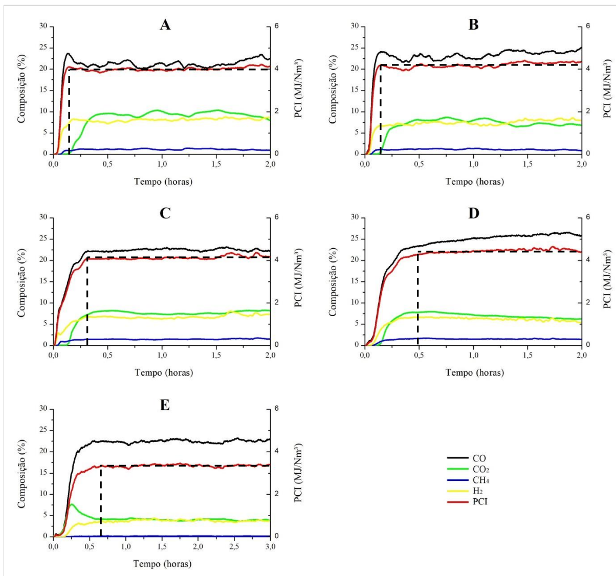
Figura 8 - Composição e poder calorífico inferior do gás obtido dos cavacos in natura (A), cavacos torrificados (B), pellets in natura (C), pellets torrificados (D) e carvão vegetal (E).
