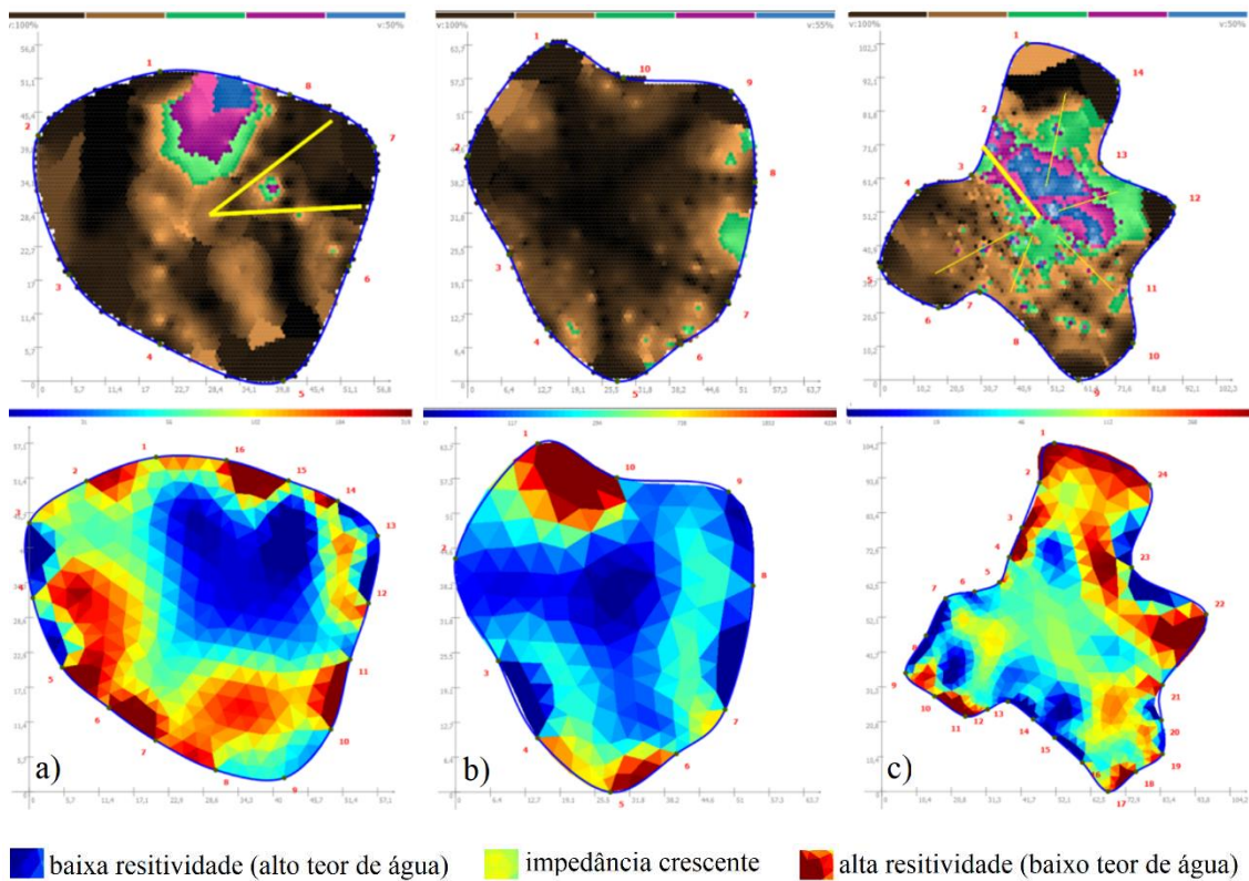
Figura 20 – Secções do tronco de indivíduos caracterizados de forma distinta quanto ao decaimento interno com o tomograma sônico (SoT) e de resistência elétrica (ERT).
