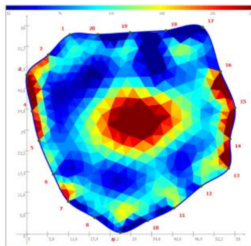
Figura 14 - Escala colorimétrica produzida pelo tomograma de resistência elétrica (ERT). Fonte: a autora
