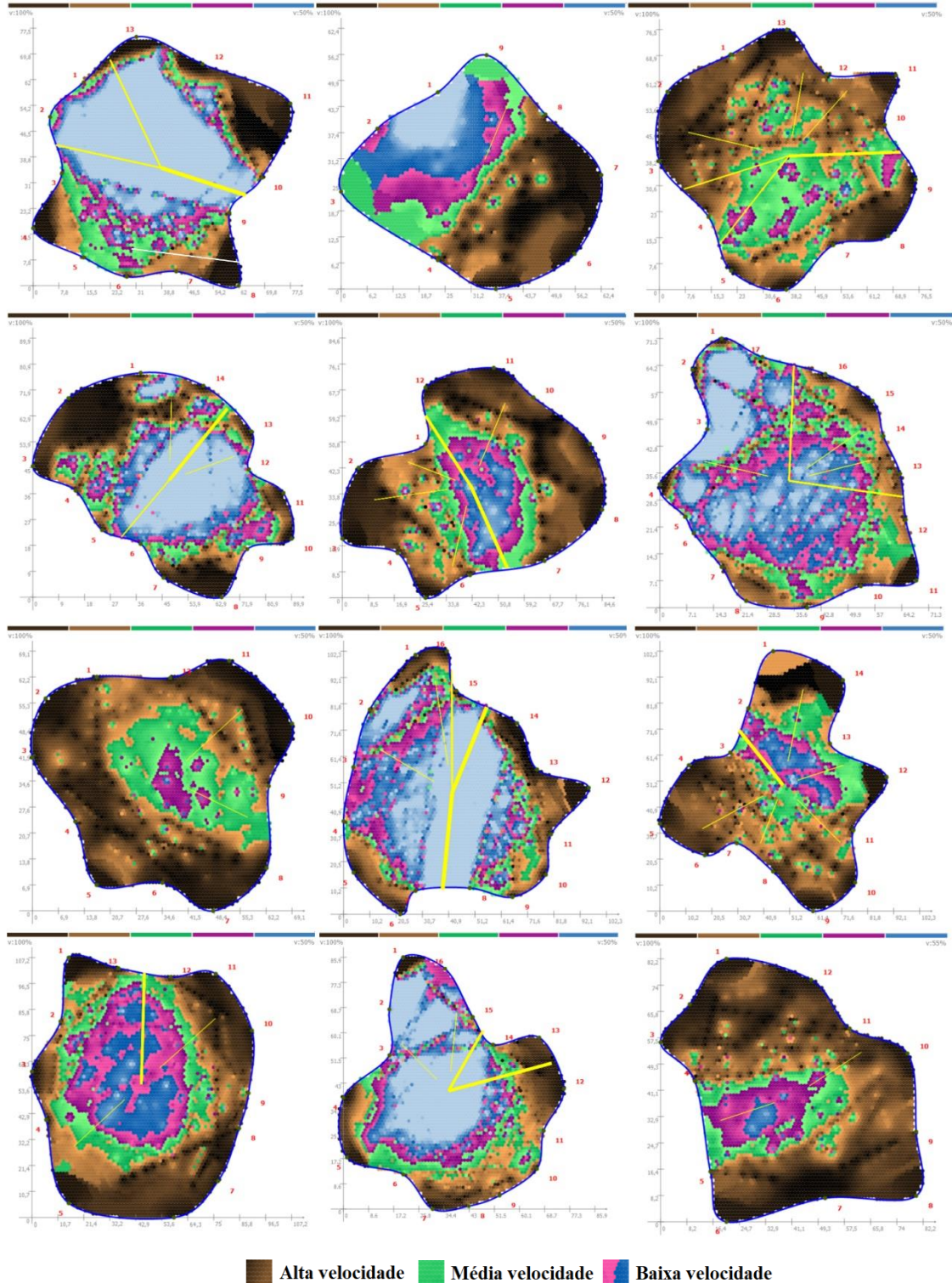
Figura 15 – Leituras das secções de indivíduos de Spathodea campanulata caracterizados com defeitos pronunciados da condição interna do tronco pelo tomograma sônico (SoT).
