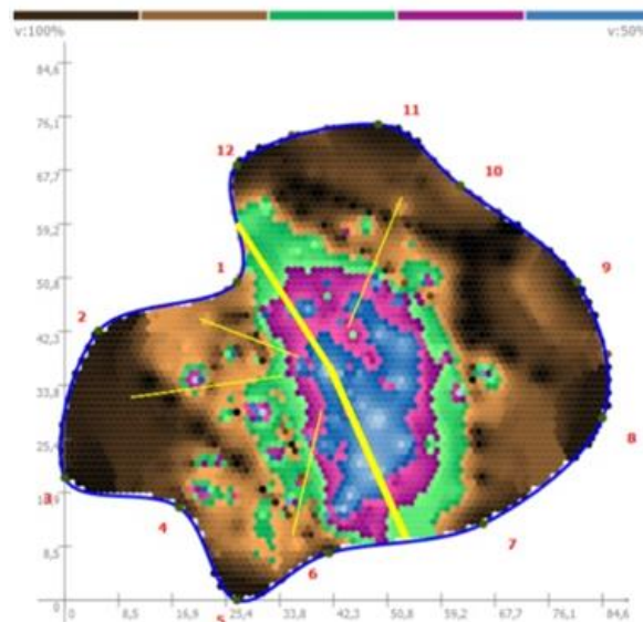
Figura 13 – Escala colorimétrica produzida pelo tomograma sônico (SoT).
