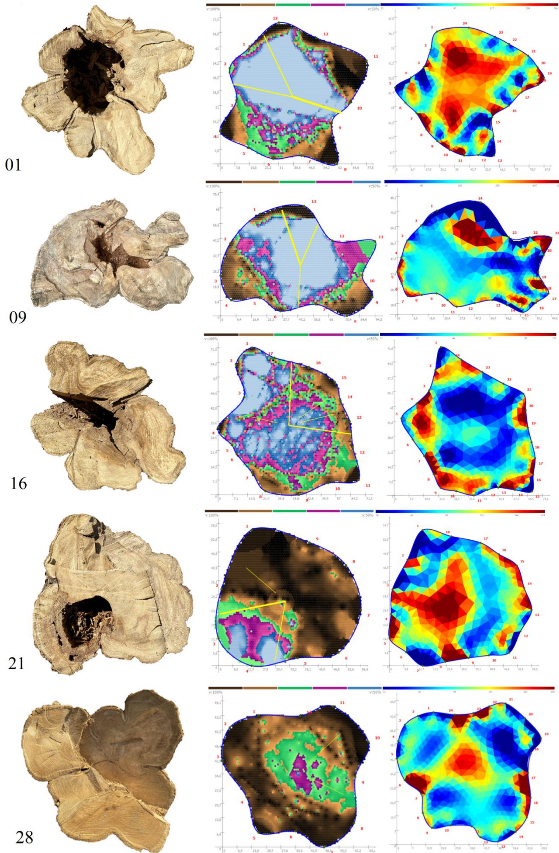
Figura 25 – comparação do corte do tronco dos indivíduos de Spathodea campanulata com os tomogramas sônico e de resistência elétrica.
