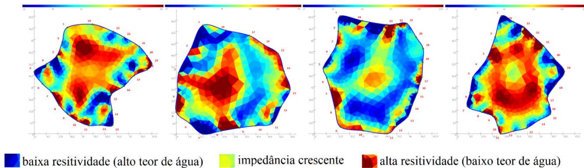
Figura 19 - indivíduos com regiões de baixa condutividade elétrica, mas com presença de cavidade previamente conhecida segundo tomograma de resistência elétrica (ERT).
