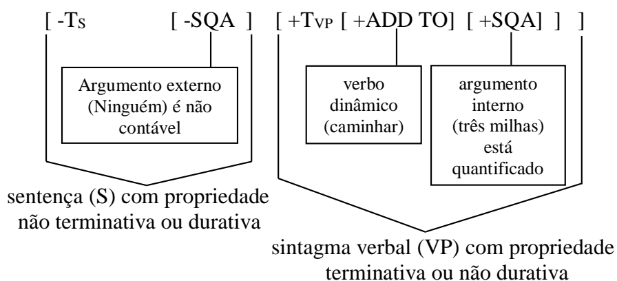
Figura 5 – Terminatividade da sentença.
