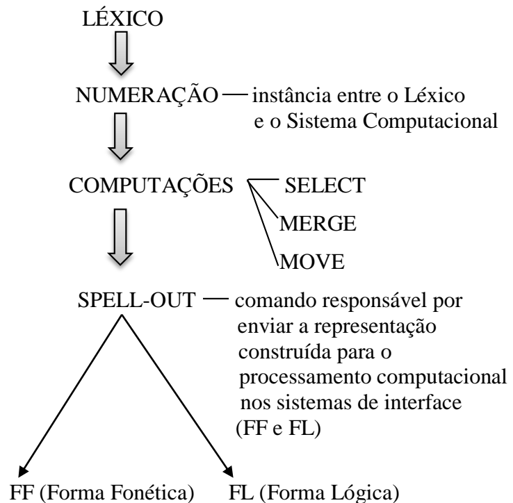
Figura 2 – O curso de uma derivação.
