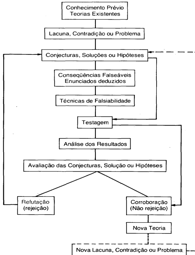
Figura 8 – Esquema proposto por Popper.
