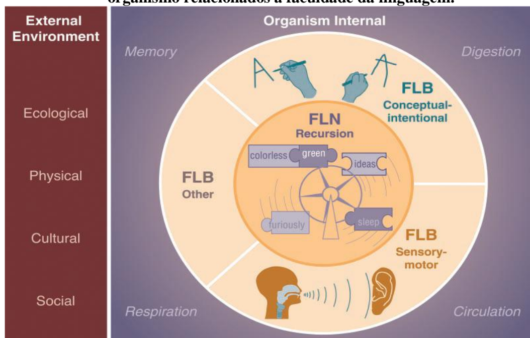
Figura 1 – Representação esquemática dos fatores internos e externos do organismo relacionados à faculdade da linguagem.
