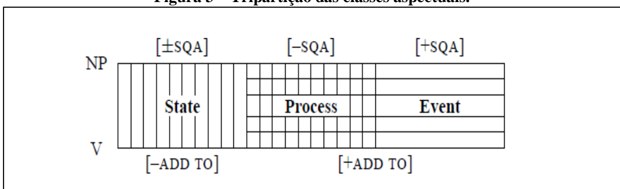
Figura 3 – Tripartição das classes aspectuais.
