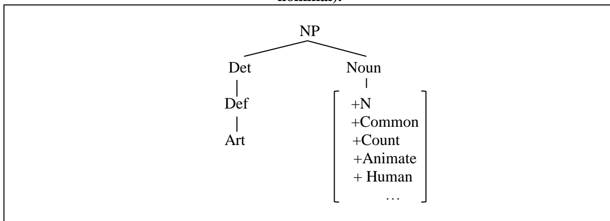
Figura 7 – Representação do nó Noun (nome) e do NP – Noun Phrase (sintagma nominal).
